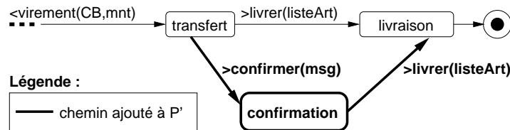
FIG. 5.5 – LTS du médiateur pour la suppression d'un acquittement
