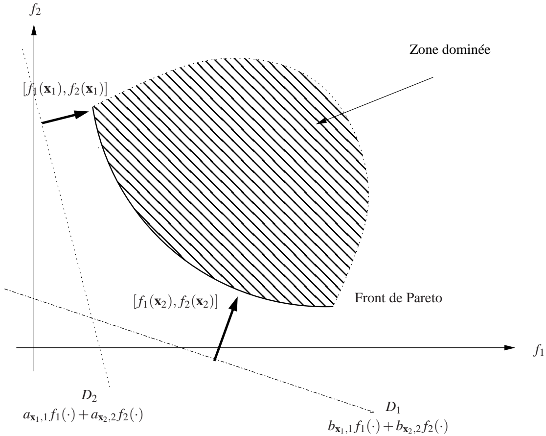
FIG. 5.1: Allure classique, dans l'espace d'arrivée, du front de Pareto d'un problème bi-objectif et correspondance entre un problème multi-objectif et une série de problèmes mono-objectifs. Si \mathbf{x}_1 et \mathbf{x}_2 sont optimaux au sens de Pareto pour le problème bi-objectif de minimisation de f_1 et f_2 , alors ils minimisent respectivement a_{\mathbf{x}_1,1}f_1(\cdot) + a_{\mathbf{x}_1,2}f_2(\cdot) et b_{\mathbf{x}_2,1}f_1(\cdot) + b_{\mathbf{x}_2,2}f_2(\cdot) .
