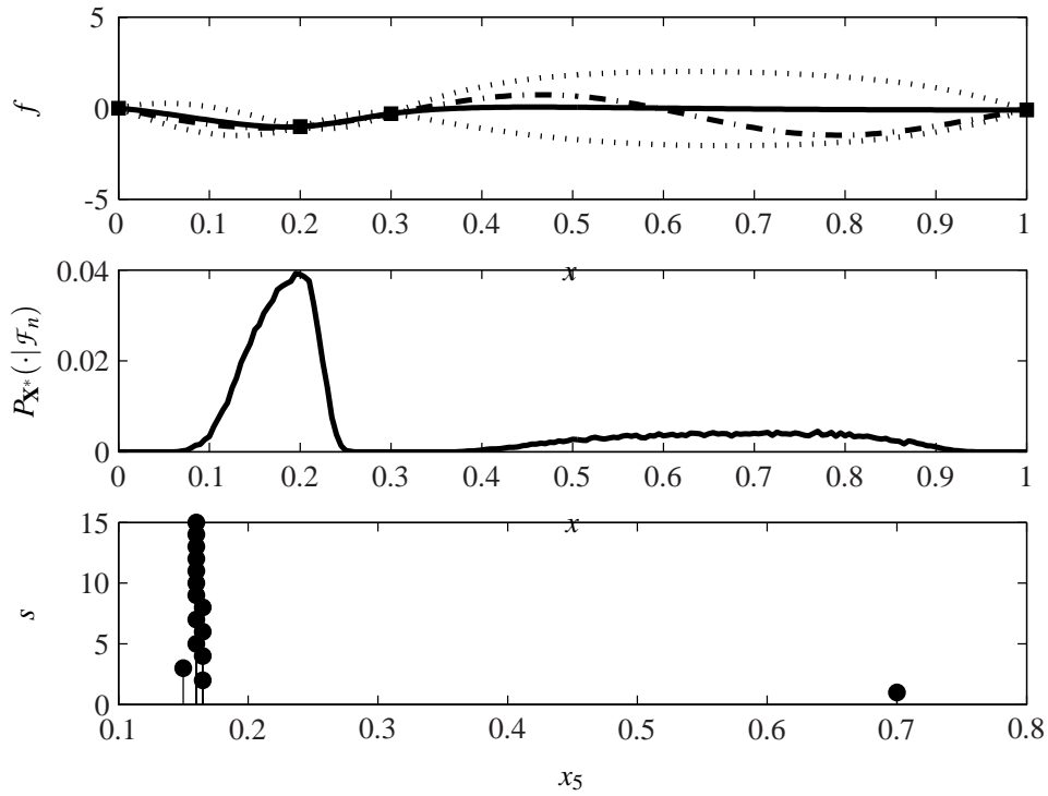
FIG. 2.2: (Partie supérieure) Prédiction par krigage (en gras) à partir de 4 résultats d'évaluation (carrés) de la fonction test utilisée pour la figure 1.11 (trait en pointillés) et intervalles de confiance associés (traits mixtes). (Partie médiane) Distribution conditionnelle des minimiseurs globaux. (Partie inférieure) Position de l'évaluation choisie par l'ECM en fonction de s . On constate que pour s \leq 8 , une imprécision apparaît pour devenir flagrante avec s = 1 .
