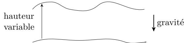
Figure 1.2: Allure du domaine pour les équations en eau peu profonde
