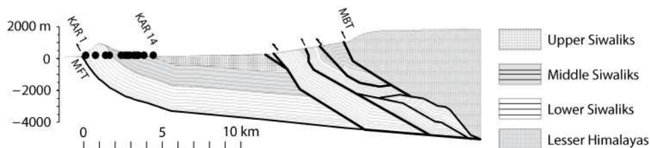
FIG. 5.2 – Coupe équilibrée de la Karnali River montrant la localisation des échantillons et la relation avec la structure tectonique locale; modifié d'après Mugnier et al. (1999) , van der Beek et al. (2006) .
