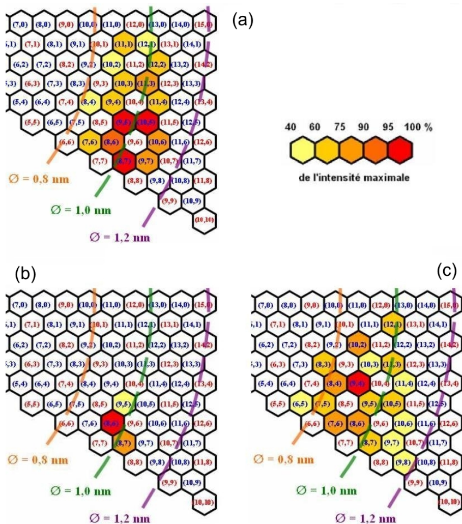
Figure 6.8 – Cartes d'intensités expérimentales de photoluminescence en fonction des indices des tubes concernées dans le repère de Hamada (a) avant sélection, (b) après sélection par la molécule pentacénique et (c) après sélection par la molécule quaterrylenique (D'après la thèse de Renaud Marquis, Strasbourg (2007))
