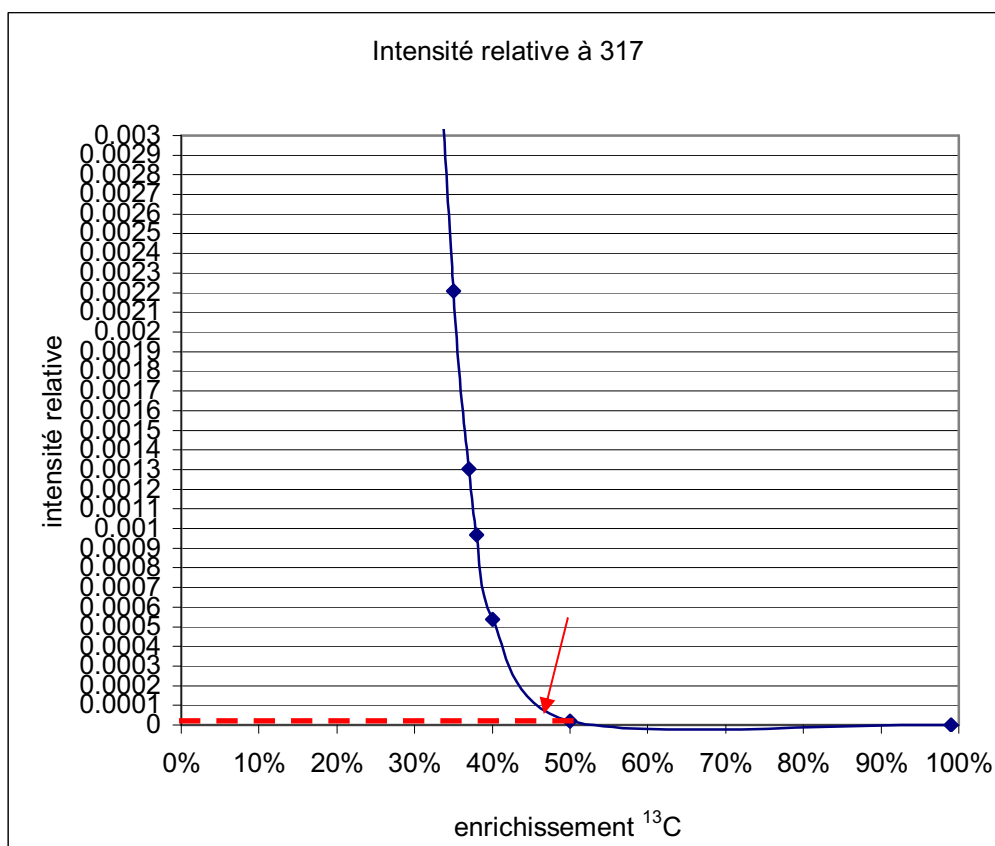
Figure II.3 : Intensité relative du pic majoritaire de la zéaralénone enrichie par rapport au pic à m/z 317 (pic majoritaire du composé totalement 12 C).
