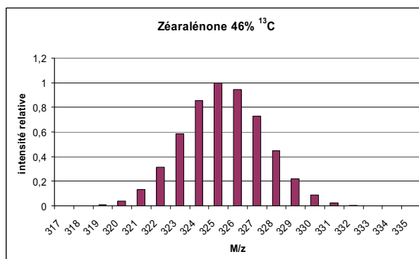
Figure II.4 : Massif isotopique calculé de la zéaralénone enrichie à 46% de 13 C (enrichissement minimal pour obtenir un pic du composé totalement 12 C ayant une intensité inférieure à 1/10 000).
