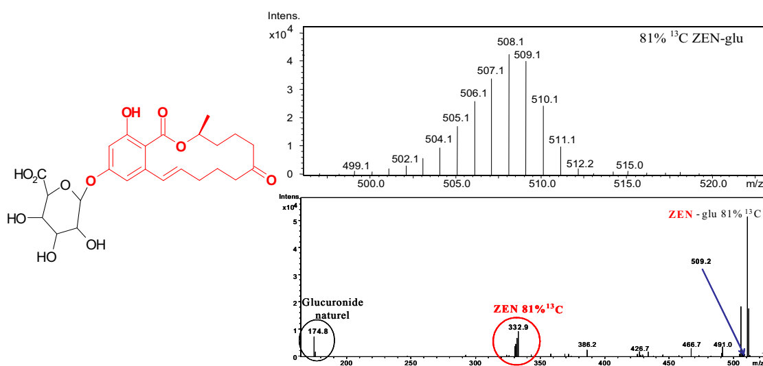
Figure IV.13 : ZEN glucuronide (gauche) ; Spectres de masse MS (droite haut) et \text{MS}^2 (droite bas) du dérivé ZEN-glucuronide enrichi à 81% de ^{13}\text{C} .
