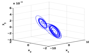
(a) Attracteur de Chua modifié.
