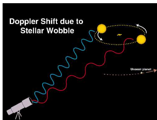
FIG. 2.1 – Illustration du décalage Doppler en longueur d'onde. (Source : http://cannon.sfsu.edu/gmarcy/planetsearch/tech/ )
