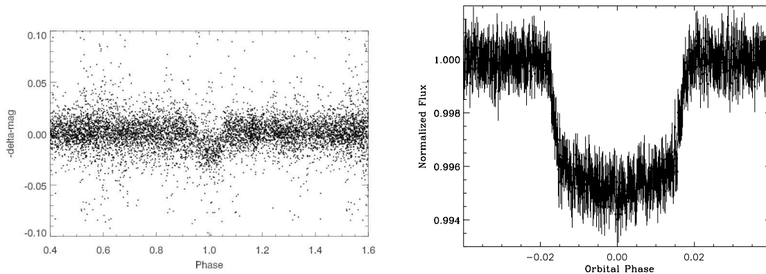
Fig. 4.1 – Courbes de lumière issus des instruments SuperWASP et CoRoT , pour les planètes WASP-12b (à gauche) et CoRoT_Exo_3b (à droite).
