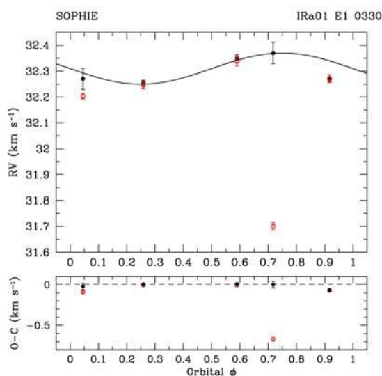
Fig. 3.8 – Effet de pollution par la Lune sur les mesures de VR. Exemple d'un jeu de VR mesurées sur une cible de faible luminosité. Les points rouges représentent les mesures non corrigées et les points noirs, les mesures corrigées.
