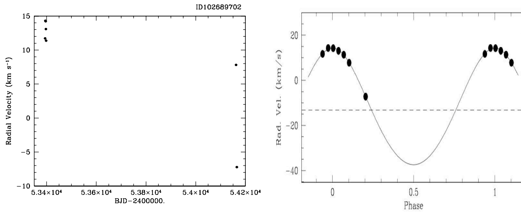
FIG. 6.4 – Mesures de VR FLAMES/GIRAFFE et SOPHIE du candidat ID 102689702 (à gauche), identifié comme étoile binaire, accompagnées du meilleur ajustement obtenu (à droite), les mesures étant remises en phase.
