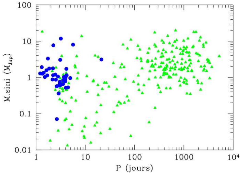
FIG. 1.4 – Diagramme mass-période des planètes connues. Les triangles verts représentent les planètes dont on ne connaît que la masse minimale. Les ronds bleus correspondent aux planètes dont la masse est exacte (non dégénérée par l'inclinaison du plan orbital par rapport à la ligne de visée).
