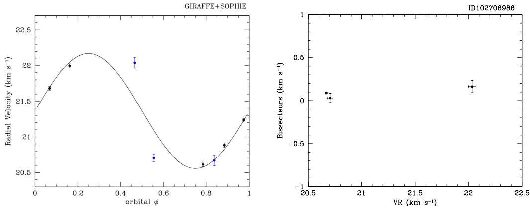
FIG. 6.6 – Mesures de VR du candidat ID 102706986 réalisées grâce à FLAMES/GIRAFFE et SOPHIE (à gauche). La figure de droite présente le bissecteur des CCF des mesures SOPHIE en fonction des mesures de VR. Les mesures FLAMES/GIRAFFE sont représentées en noir, tandis que les mesures SOPHIE sont en bleu.
