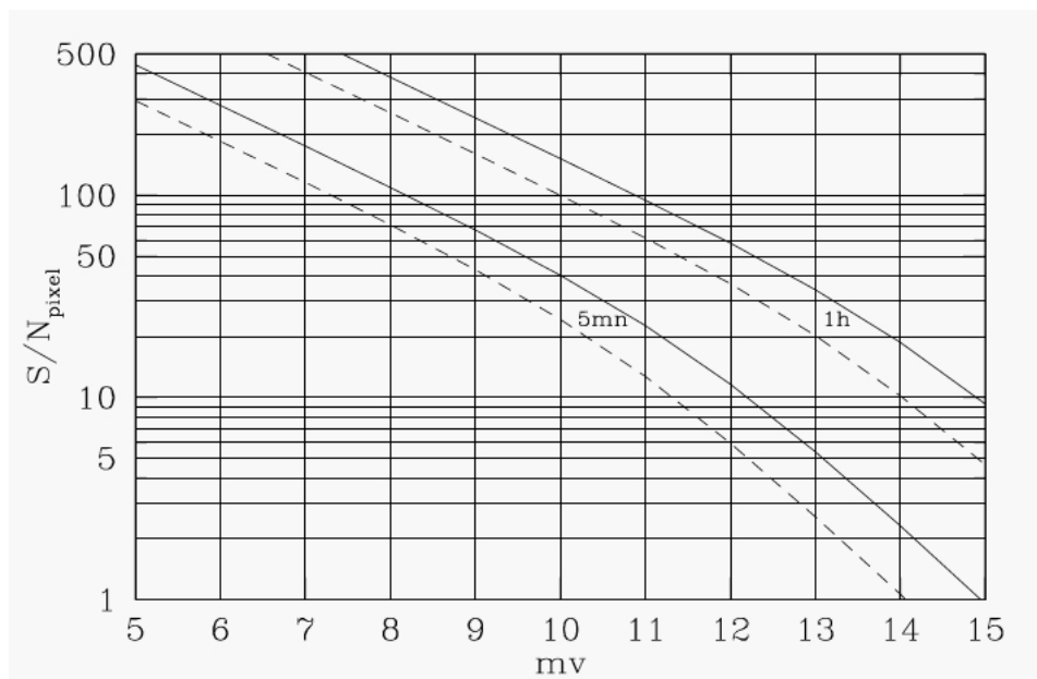
FIG. 2.12 – Performances nominales du spectrographe SOPHIE , par temps clair et un seeing de 2.5 arcsec, illustrant le niveau de S/N obtenu en fonction de la magnitude de l'objet observé et du temps de pose utilisé. En pointillés, la courbe représente les performances du mode HR et en ligne pleine, celles du mode HE.
