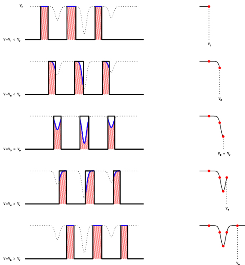
FIG. 2.4 – Schéma de principe de la méthode de corrélation croisée (tirée de la thèse de C. Melo).
