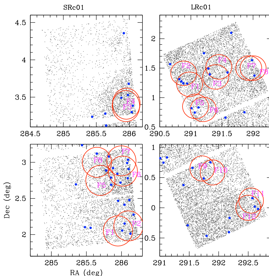
FIG. 6.10 – Disposition des champs d’observation FLAMES/GIRAFFE au sein des champs LRc01 et SRc01. Les points bleus représentent les candidats, les triangles verts représentent les étoiles binaires identifiées grâce à leur CdL, potentiellement intéressante à observer. Les points noirs en fond représentent l’ensemble des étoiles des champs LRc01 et SRc01.
