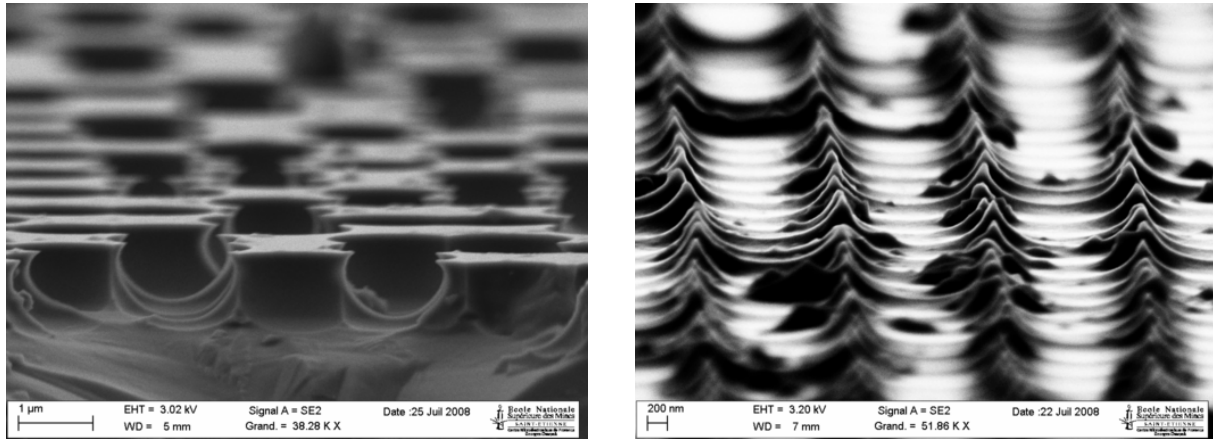
(a) Zone n° 1. Résultat d'une gravure à travers un masque de silice imparfaitement ouvert.
