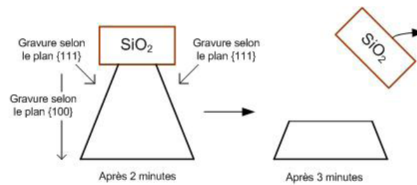
FIG. 3.21 – Schéma explicatif du décollage du masque de silice sur silicium qui intervient lorsque la sous gravure est trop importante.
