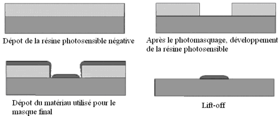
FIG. 3.37 – Procédure de réalisation du masque de chrome sur Germanium. Technique de lift-off « simplifiée ».
