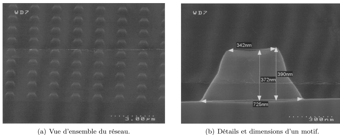
FIG. 3.28 – Images MEB des motifs de silice sur silicium du lot n° 3. (a) Vue d'ensemble. (b) Détails et dimensions.
