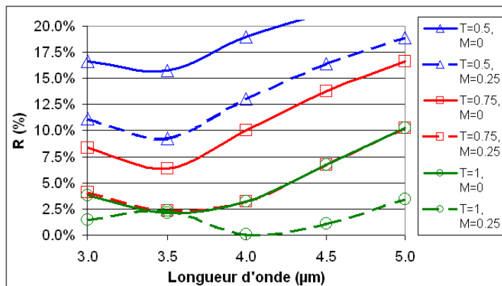
FIG. 2.15 – Facteurs de réflexion R en incidence normale, en fonction de la longueur d'onde incidente. Pour chaque valeur de hauteur T de pyramide ( T \in [0,5; 0,75; 1]\mu m ), deux tailles de méplat M sont simulées ( M = 0\mu m et M = 0,25\mu m ). Les autres paramètres sont fixes. La période P de la structure est égale à 1\mu m .
