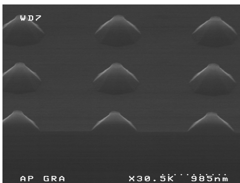
(c) Structure sur silicium obtenue par gravure au TMAH. P = 1,5\mu m .
