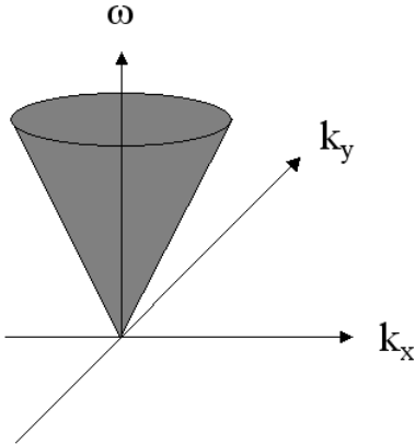
FIG. 2.24 – Surface de dispersion conique d'un milieu homogène bidimensionnel.
