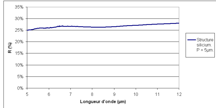
FIG. 4.9 – Facteur de réflexion mesuré sur l'échantillon de silicium gravé par TMAH et P = 5\mu m .
