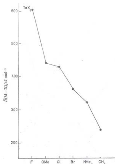
Figure 20 : Valeurs des enthalpies moyennes de liaison D(\text{M-X}) dans les composés \text{MX}_n gazeux avec M = \text{Ta} pour X = \text{F}, -\text{OCH}_3, \text{Cl}, \text{Br}, -\text{N}(\text{CH}_3)_2 et -\text{CH}_3 [Adedeji1979].
