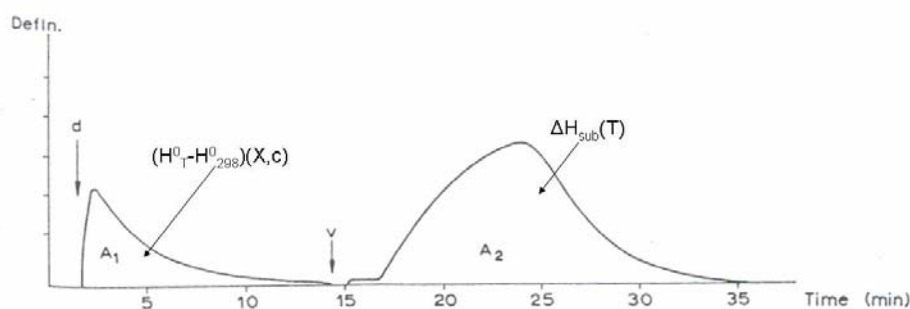
Figure 19 : Exemple d'un thermogramme de sublimation de l'anthracène, d = chute de l'échantillon, v = mise sous vide et defln = déflexion du galvanomètre [Adedeji1975].
