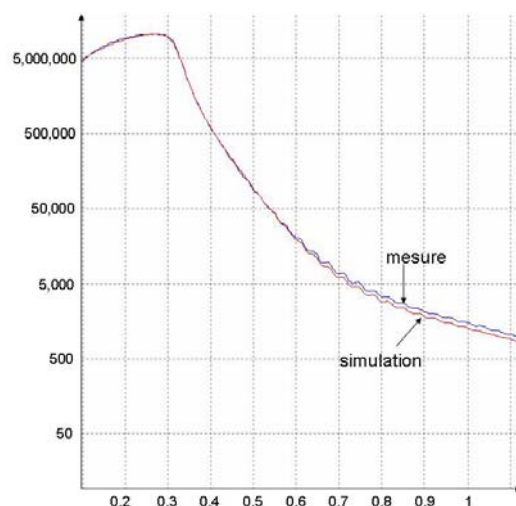
Figure 103 : Analyse de l'échantillon Al par réflectométrie.
