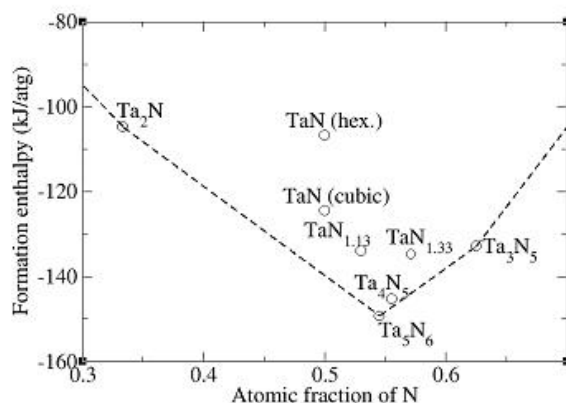
Figure 11 : Enthalpies de formation à 0 K de différents composés Ta_xN_y déterminées par calcul ab-initio [Lebacq2006].
