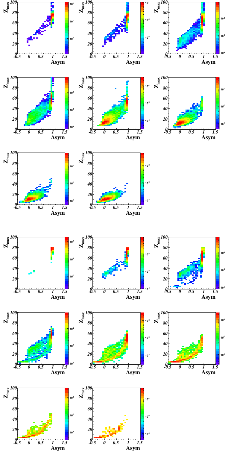
FIG. 5.5 – Système Au+Au à 80 MeV/u. Corrélations entre Z_{max} et Asym par tranches d'énergie transverse réduite, pour les événements sélectionnés avec Z_{max} émis à l'arrière. En haut : les données. En bas : le modèle.
