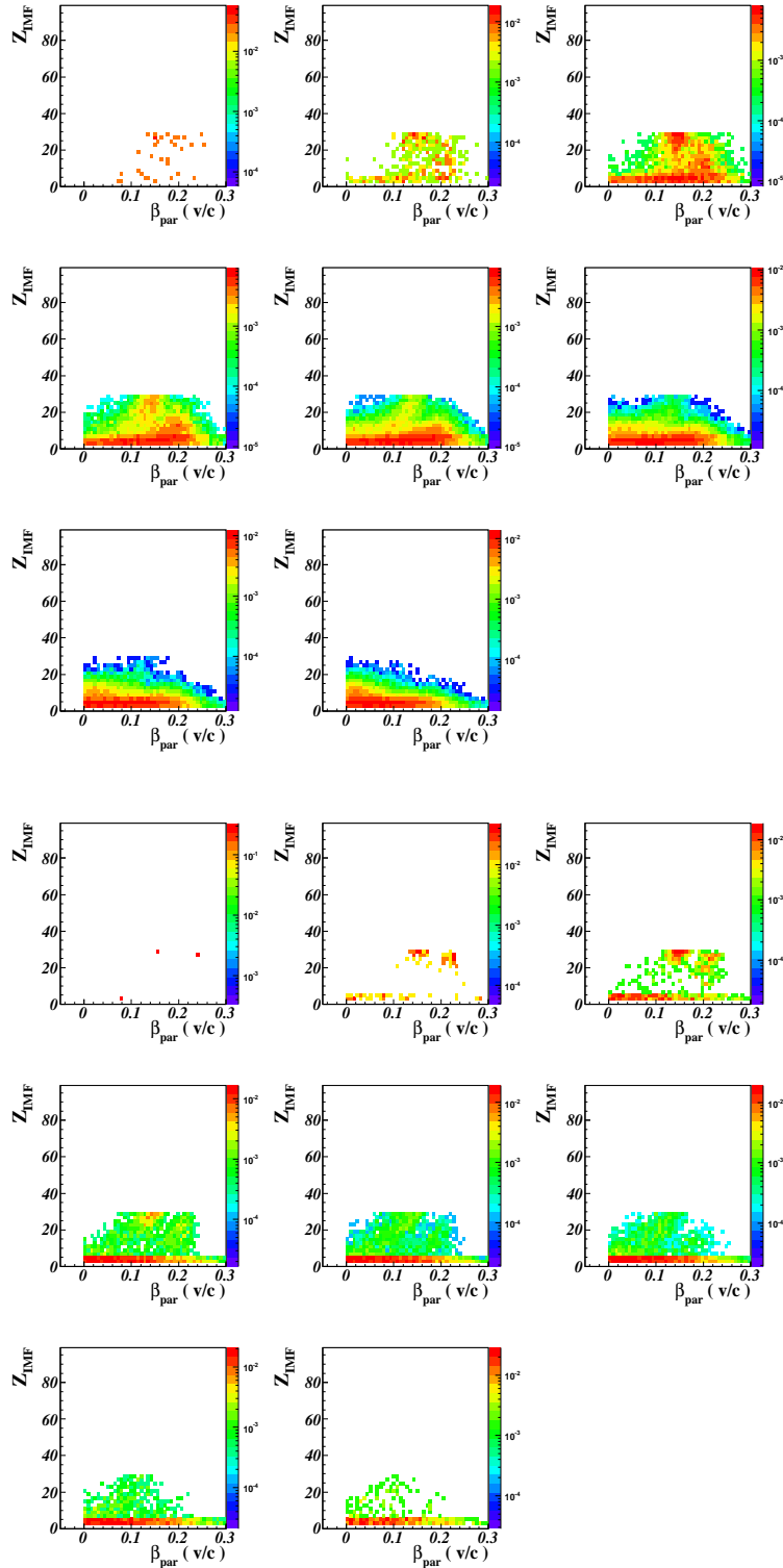
FIG. 5.7 – Système Au+Au à 80 MeV/u. Corrélations entre la charge Z des IMFs, de la branche gaz ( Z_{\text{max}} < 30 ), et leur vitesse parallèle au faisceau V_{\text{par}} , par tranches d'énergie transverse réduite, pour les événements où Z_{\text{max}} est émis à l'arrière. En haut : les données. En bas : le modèle.
