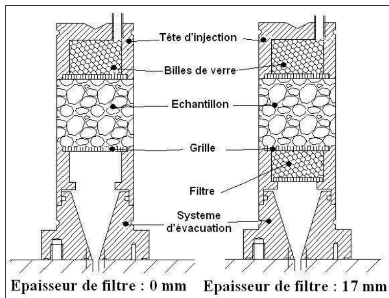
Figure 31 : Schéma du système d'injection et d'évacuation
