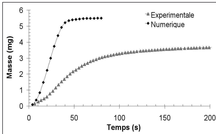
Figure 84 : Comparaison essai A1 et modélisation numérique (évolution de la masse)
