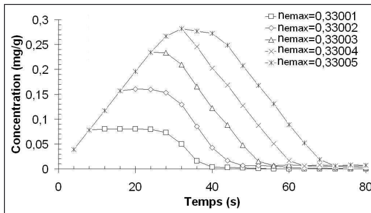
Figure 81 : Evolution de la concentration de l'effluent en fonction du temps pour différentes valeurs de n_{e_{max}}
