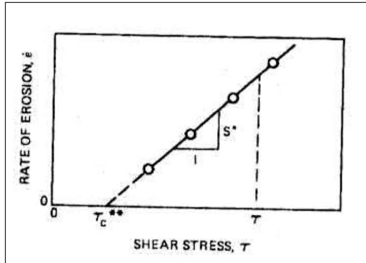
Figure 15 : Taux d'érosion en fonction de la contrainte de cisaillement hydraulique (Arulanandan et Perry, 1983)
