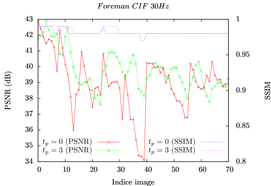
FIG. 5.11 : Placer l'instant de projection en milieu de GOF permet d'améliorer la qualité moyenne des images synthétisées.
