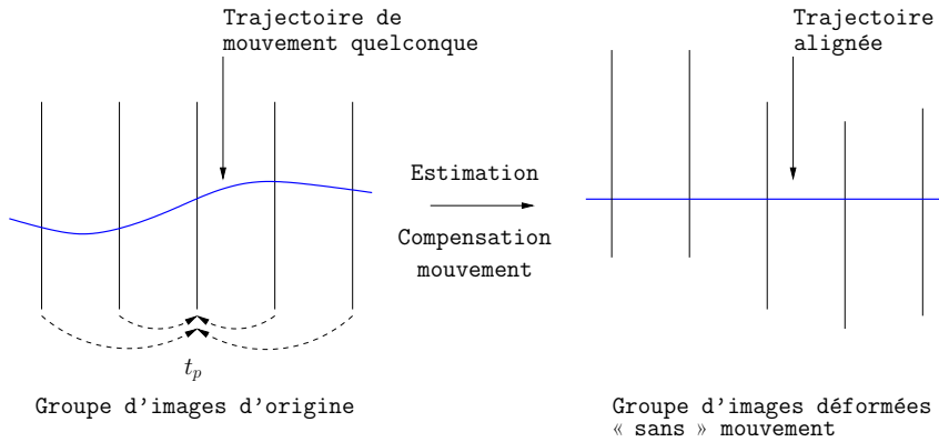
FIG. 5.2 : Illustration 1D de l'analyse temporelle. Les images du GOF sont projetées au même instant de projection t_p . À l'issue de cette projection, le groupe d'images déformées est décorrélaté temporellement.
