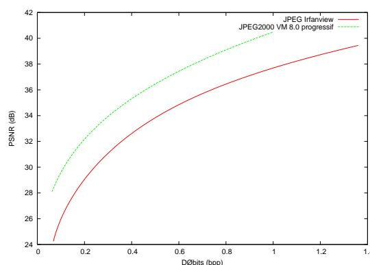
FIG. 1.13 : Comparaison des courbes PSNR=f(Débit) de JPEG et JPEG2000 avec l'image Lena 512. La compression JPEG a été effectuée avec le logiciel Irfanview. La compression JPEG2000 a été effectuée avec le codeur VM (« Verification Model ») 8.0 en utilisant le mode progressif à granularité fine.
