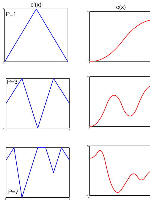
FIG. 2.15 : A gauche, courbes c'(x) obtenues en sommant P B-spline linéaires translattées. A droite, les courbes de flux obtenues en intégrant c'(x) .
