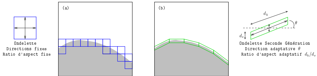
FIG. 1.9 : (a) La décomposition en ondelettes génère un grand nombre de coefficients significatifs autour d'une discontinuité, (b) Intégrer une dose d'anisotropie permet de capturer le contour et de générer un petit nombre de coefficients significatifs.
