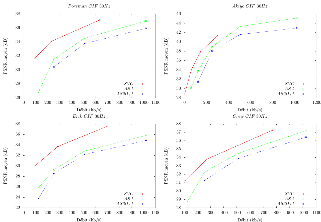
FIG. 5.14 : Courbes débit-distorsion obtenues pour quatre vidéo tests au format CIF 30 Hz.
