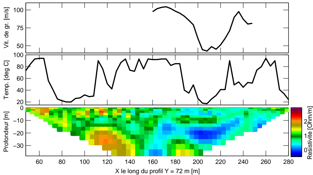
FIG. 4.18 – Vitesse de groupe, température et modèle de résistivité inversé le long du profil Y = 72 m. Les zones de surface conductrices humides correspondent à des zones de faible température. Lorsque la température augmente, le fluide se vaporise et la vapeur chaude assèche le milieu, le rendant moins conducteur et plus rapide. En profondeur le fluide reste sous forme liquide, sa température d'ébullition étant plus importante à cause de la pression.
