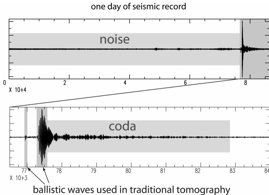
FIG. 1.3 – Un jour d'enregistrement continu incluant un séisme de grande magnitude. Environ 95 % de l'enregistrement est du bruit sismique, 4 % de la coda et les ondes directes utilisées pour l'imagerie sismique traditionnelle ne représentent qu'un pourcent du signal.
