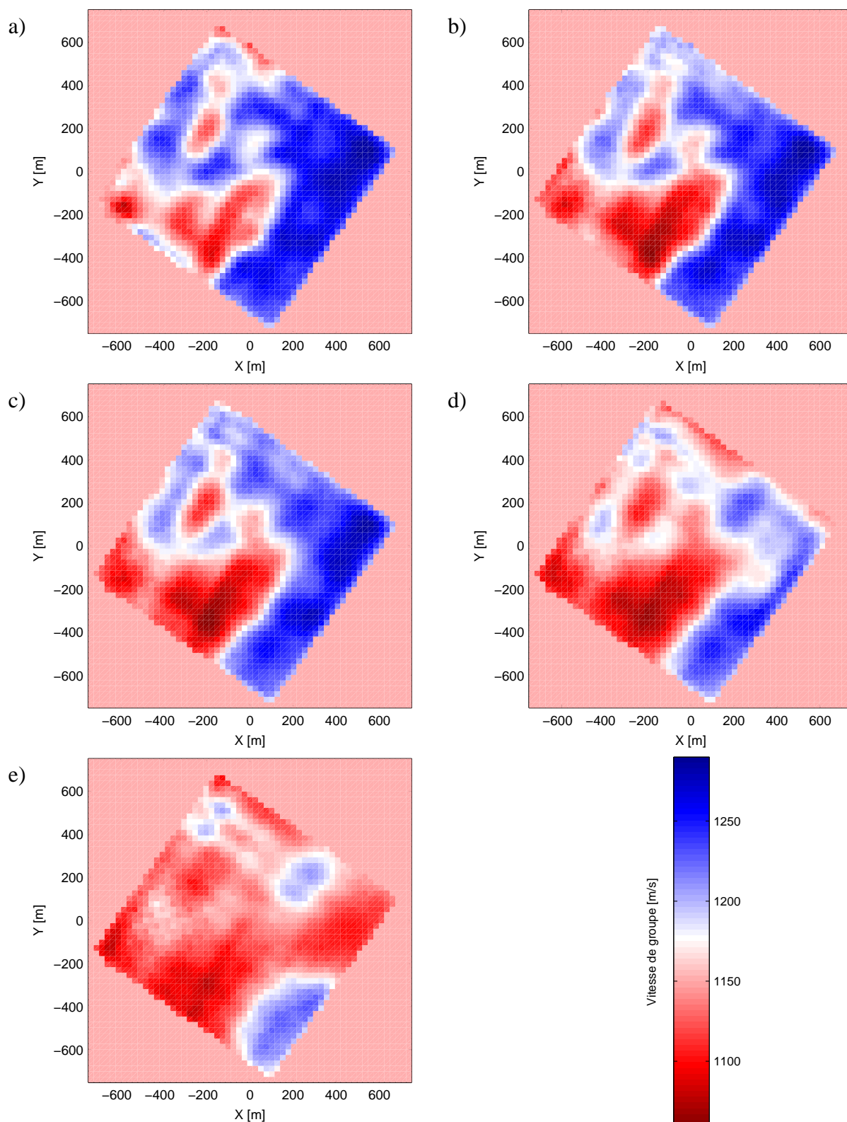
FIG. 2.13 – L’algorithme d’inversion est utilisé pour des tailles cellules élémentaires de 8 (figure a.) à 12 (figure e.) éléments dans les lignes de sources et de récepteurs (ces éléments étant séparés de 25 m). L’image est la même quelque soit la taille de cellule utilisée, mis à part le contraste ( i.e. , la valeur de la vitesse), le modèle obtenu étant d’autant plus lisse que la cellule est grande. Le modèle obtenu avec une cellule de 12 éléments est différent des autres modèles, à cause d’erreurs dans la mesure des temps de propagation.
