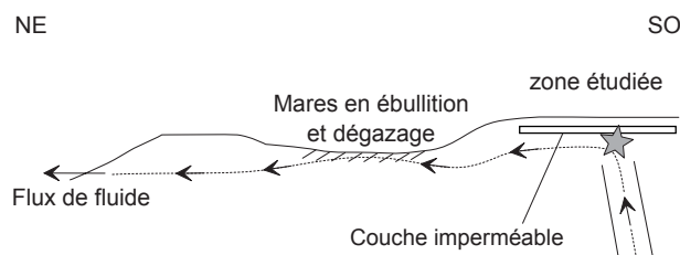
FIG. 5.9 – Modèle expliquant la présence simultanée d’une source acoustique et d’un dipôle électrique (indiqués par l’étoile grise), avec une fuite du fluide et ébullition et un dégazage en surface déportés par rapport à la position de ces sources.
