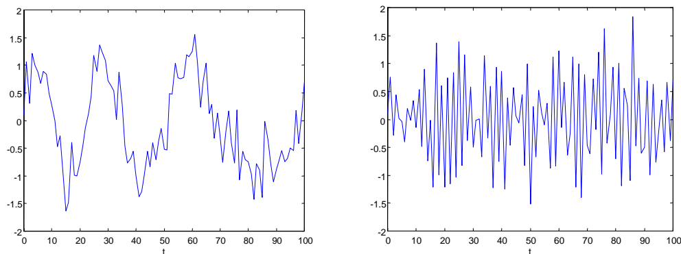
Figure 4.9. Deux signaux aléatoires de même variance.
