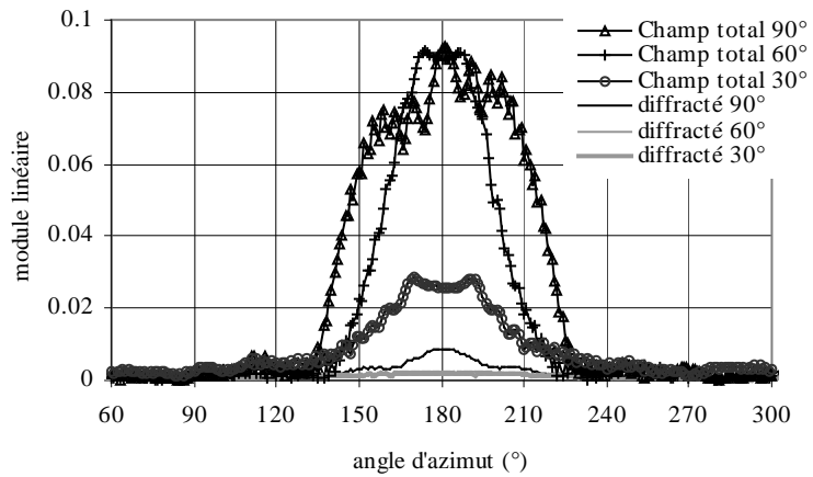
Figure 10b : Comparaison des niveaux (modules linéaire) entre la mesure du champ total et la valeur du champ diffracté pour les configurations multi-statique avec les angles de sites de 90^\circ , 60^\circ et 30^\circ présentés dans la figure 9b.
