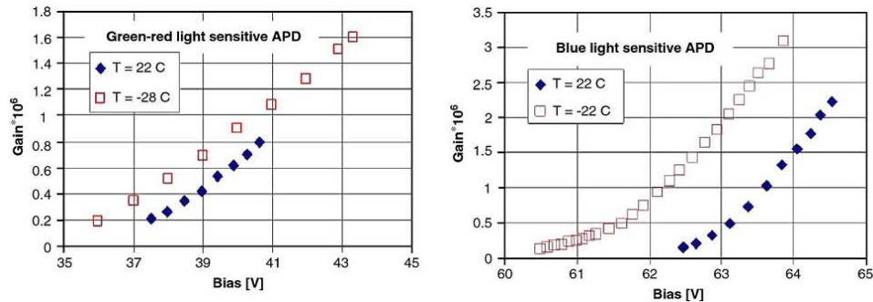
Graphique 4.30 : Présentation du gain des dispositifs CPTA.
