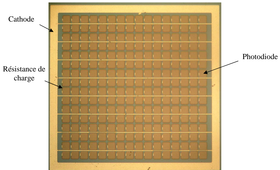
Figure 2.10 : Photographie d'un SiPM (fabrication LAAS) 16*16 photodiodes de 40 \mu m de côté.
