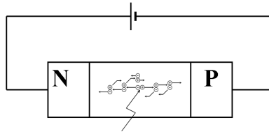
Figure 2.2 : L'avalanche dans les jonctions polarisées en inverse.
