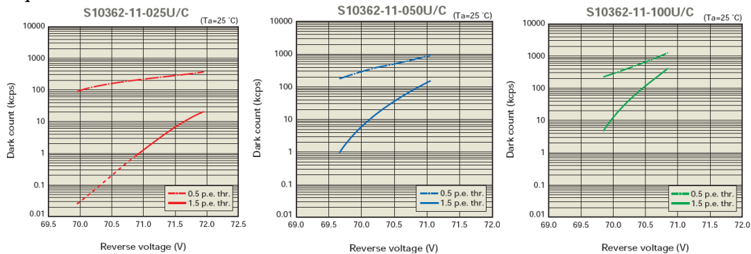
Graphique 4.31 : Le déclenchement thermique expérimental des trois SiPM de Hamamatsu en fonction de la tension d'alimentation.
