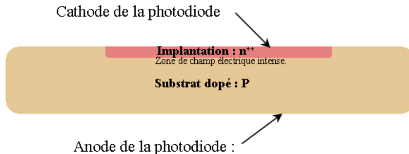
Figure 2.11 : Structure de la photodiode
