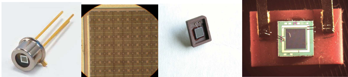
Figure 1.4 : Les SiPM de Hamamatsu [Réf 1. 27].
