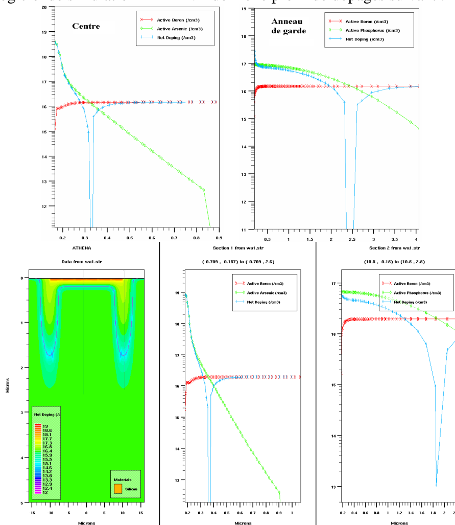
Graphique 3.1 : Profil de dopage, au centre et sur l'anneau de garde pour un substrat de résistivité 0,85 \Omega.cm (gauche) et un 0,75 \Omega.cm (droite).
