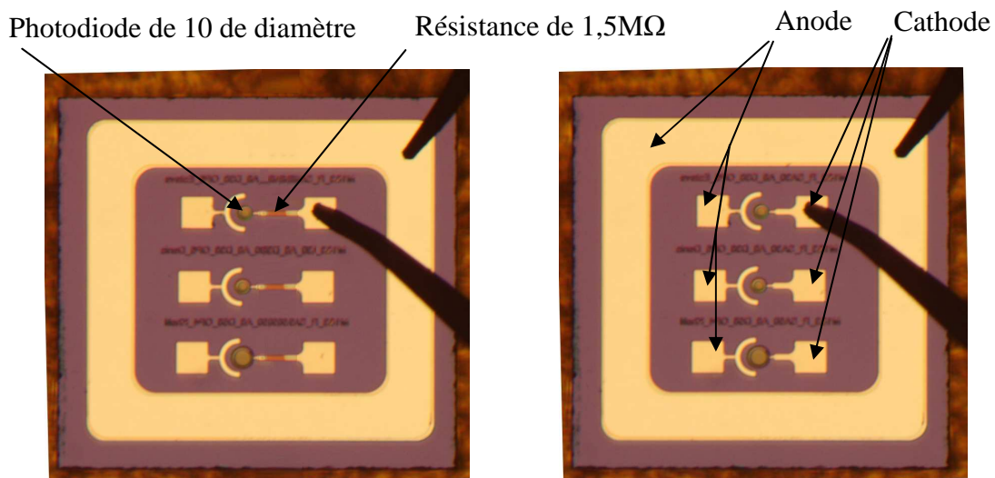
Figure 4.5 : Trois photodiodes de 10, 20 et 30 µm de diamètre, avec et sans resistance.
