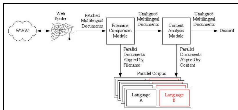
Figure 32. Architecture du système PTI
