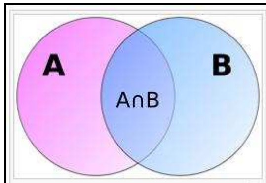
Figure 78. Intersection entre deux ensembles A et B 1
