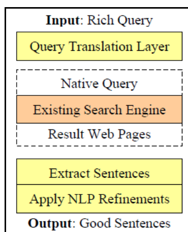
Figure 21. Etapes de traitement de GoogleLing
