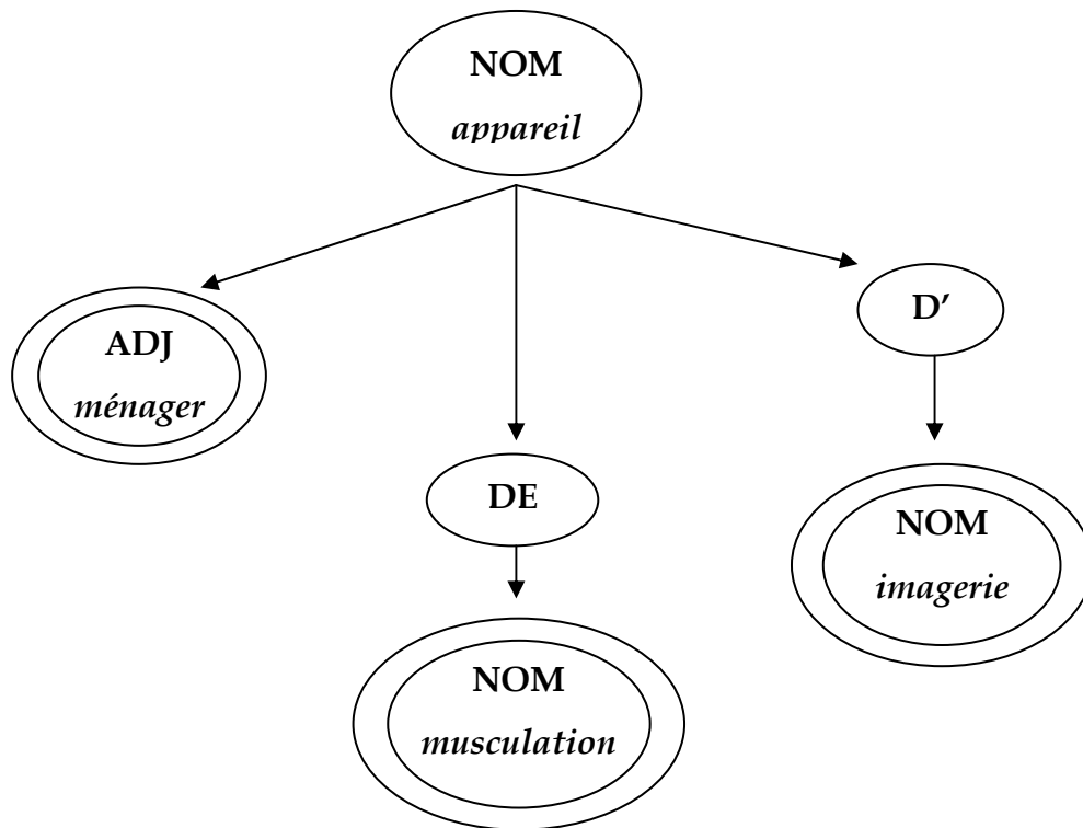
Figure 48. Graphe de décision des patrons syntaxiques pour l'identification des termes complexes
