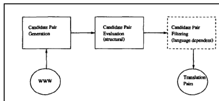
Figure 31. Architecture du modèle STRAND
