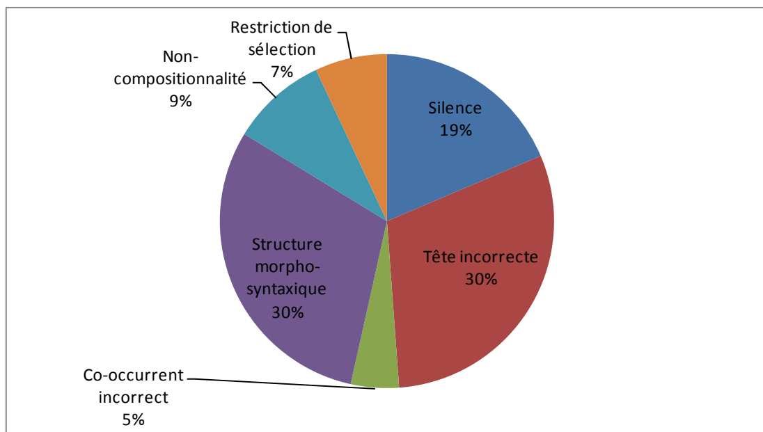
Figure 67. Proportion de traductions rejetées par catégories
