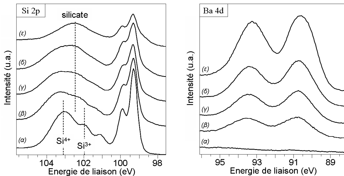
Fig. III.9 – Détail des spectres SR-PES des transitions (a) Si 2p et (b) Ba 4d acquis aux premières étapes du dépôt à température ambiante, (a) 0 eq. ML, (β) 0.2 eq. ML, (γ) 0.4 eq. ML, (δ) 0.5 eq. ML, (ε) 1 eq. ML.
