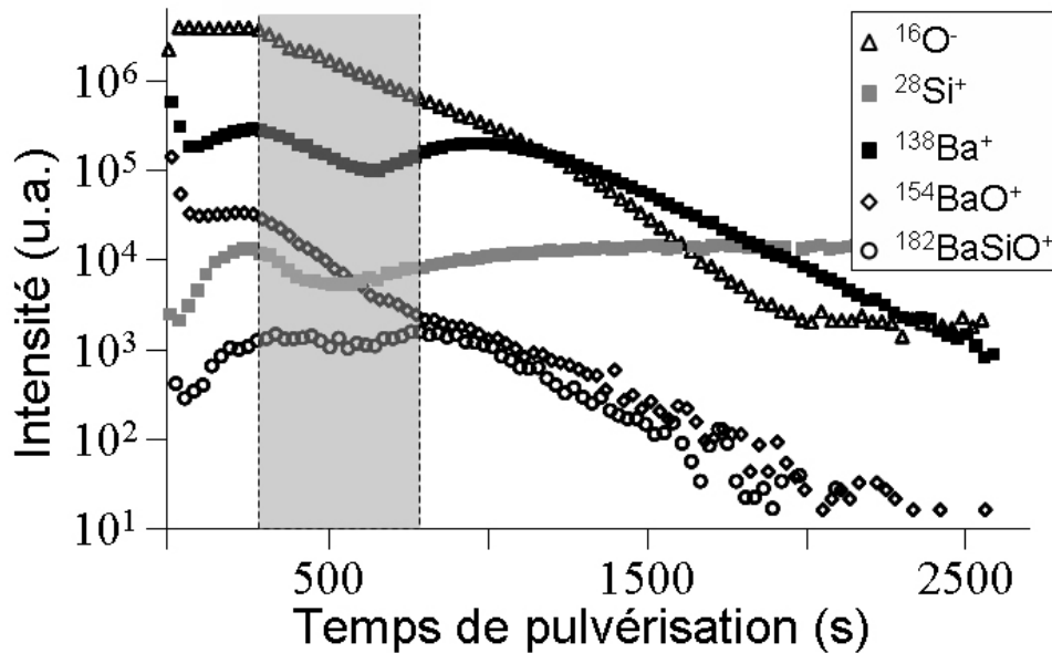
Fig. IV.10 – Profil SIMS d'un film de silicate de baryum, élaboré à 580 °C, par expositions à l'oxygène (6L) et évaporations de baryum successives.
