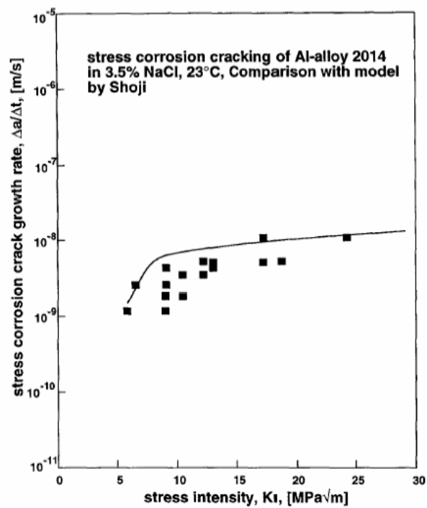
Figure III-12 : Effet du facteur d'intensité des contraintes sur la vitesse de propagation en CSC de l'alliage 2014 immergé deux fois par jour dans NaCl 3.5%. Les carrés sont les valeurs expérimentales et la courbe, les valeurs prédites par le modèle de Shoji [Vogt, 1998].
