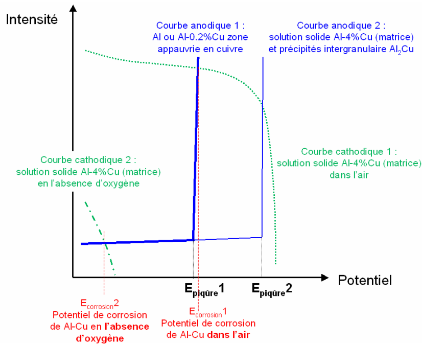
Figure II-21 : Courbe intensité potentiel de l'aluminium et de Al-4%Cu en solution chlorurée d'après [Galvele, 1970] : E_{piqûre\ 1} : potentiel de piqûre de la zone appauvrie en cuivre et E_{piqûre\ 2} : potentiel de piqûre de la matrice.
