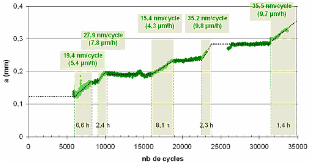
Figure IV-47 : Evolution au cours du temps du signal électrique converti en « longueur » de fissure pour un essai de FC sur éprouvette entaillée ( \sigma_{\max}=250 MPa, R=0.6 et f=0.1 Hz). On note les discontinuités du signal électrique dans les premiers instants.
