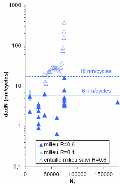
Figure IV-55 : a) Profondeurs et b) Vitesses de propagation de fatigue corrosion (i) déterminées sur des essais interrompus sur des éprouvettes lisses présentant des défauts intergranulaires semi-elliptiques isolés en supposant la vitesse constante (symboles pleins) et (ii) déterminées sur des éprouvettes entaillées instrumentées avec le suivi électrique (vitesse instantanée) (symboles ouverts) dans les mêmes conditions mécaniques ( R=0.6 , f=0.1 Hz, \sigma_{\text{max}}=250 MPa), La droite continue présente la vitesse moyenne de propagation transgranulaire des défauts semi-elliptiques isolées et la droite en pointillés présente la vitesse moyenne de propagation transgranulaire dans le cas des éprouvettes entaillées.
