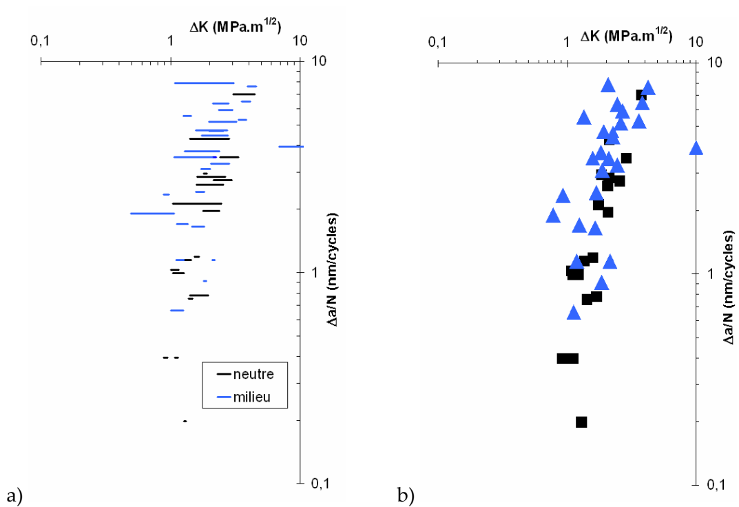
Figure IV-63 : Vitesse de propagation de la fissure transgranulaire, considérée constante a) en fonction du \Delta K_{inter/trans} et du \Delta K_{final} et b) en fonction d'une amplitude de facteur d'intensité des contraintes moyenne.
