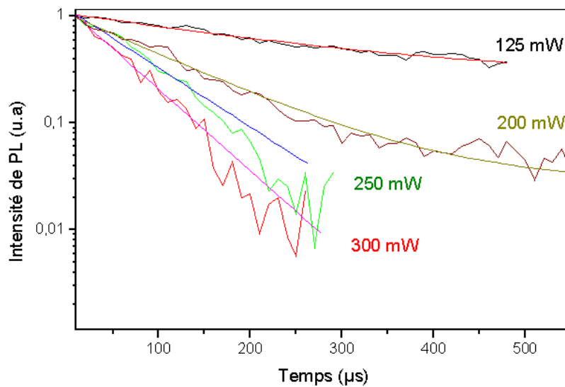
FIG. 4.8 – Variation du temps de déclin de photoluminescence à 1,53 \mu m correspondant à la transition {}^4I_{13/2} à {}^4I_{15/2} à la température ambiante dans le cas d'un guide plan pour différentes puissances d'excitation
