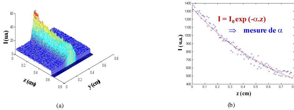
FIG. 2.14 – Profil de l'intensité à 1,55 \mu\text{m} de la lumière diffusée à 2D (a), et de l'intensité de lumière diffusée en fonction de la distance de propagation (b).
