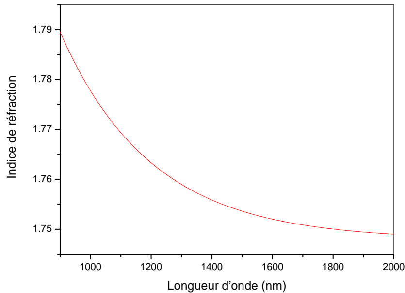
FIG. 2.10 – Courbe de dispersion d'indice d'une couche de silicium poreux de porosité égale à 62% et d'épaisseur égale à 5 \mu\text{m} en utilisant le modèle de Bruggeman
