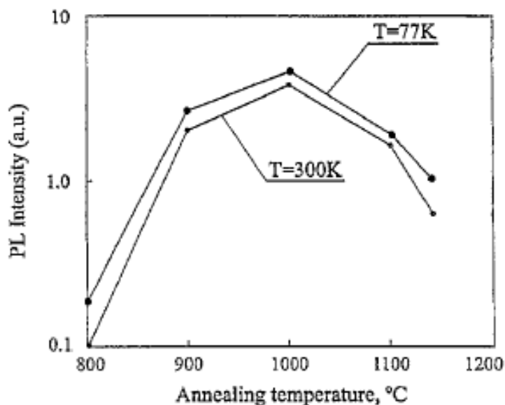
FIG. 1.9 – Intensité de PL à 300 K et 77 K du silicium poreux de type P dopé erbium en fonction de la température de recuit (RTA) [42]
