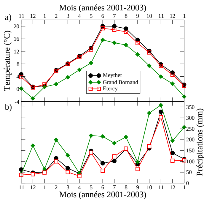
Figure 3.5: Température ( \pm 0,25^\circ\text{C} ), et précipitations ( \pm 0,1\text{mm} ) mensuelles aux stations d'Etercy, de Meythet et du Grand-Bornand de fin 2001 à début 2003.
