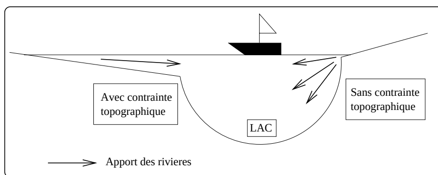
Figure 2.4: Illustration de l'effet de la topographie du lac sur la zone de mélange des apports.
