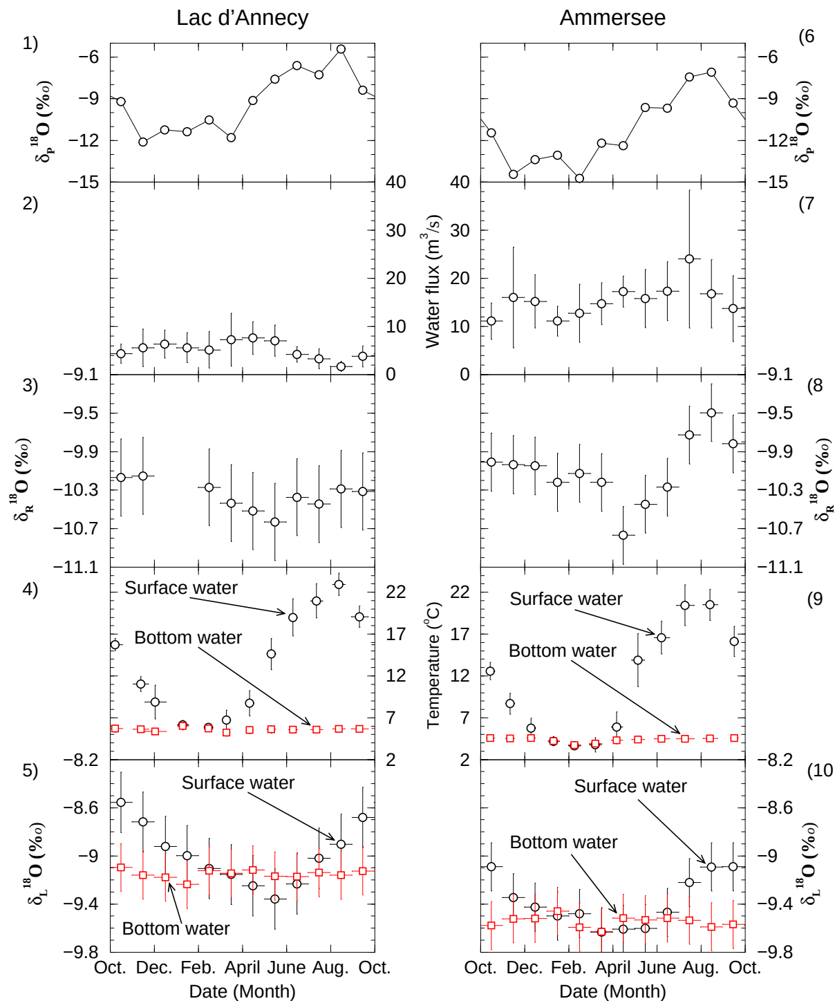
Figure 3.22: Observations moyennes mensuelles utilisées pour la calibration du MoHydIsoLac (voir détails dans le texte).
