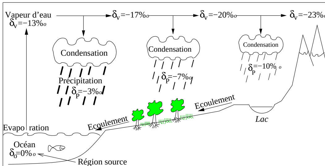
Figure 1.2: Cycle atmosphérique de l'eau associé au cycle isotopique. \delta_v : composition isotopique de la vapeur, \delta_p : composition isotopique des précipitations
