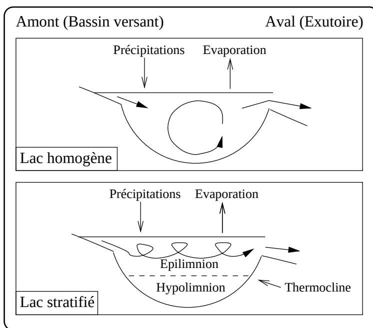
Figure 2.5: Illustration de l'effet de passage estival (ou 'summer bypass effect' en anglais).
