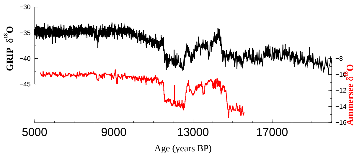
Figure 1.4: Comparaison de la reconstruction isotopique des précipitations à partir des coquilles carbonatées d'ostracodes benthiques à Ammersee (Allemagne) et à partir de la calotte glaciaire du Groenland (figure 1.3) entre 15 000 et 5 000 BP [von Grafenstein et al. , 1999a].
