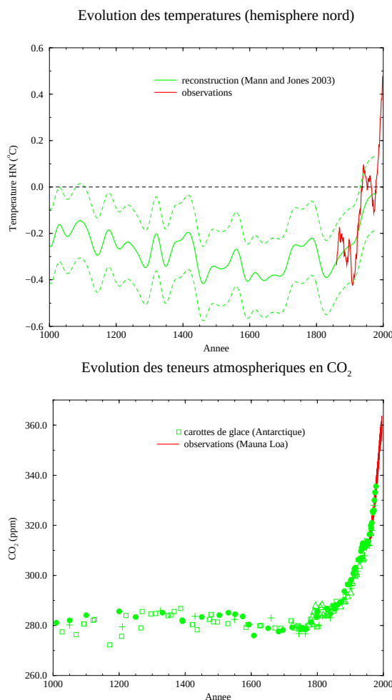
Figure 1.1: Reconstructions et observations des températures de l'hémisphère nord (haut) et des teneurs atmosphériques en CO_2 (bas).
