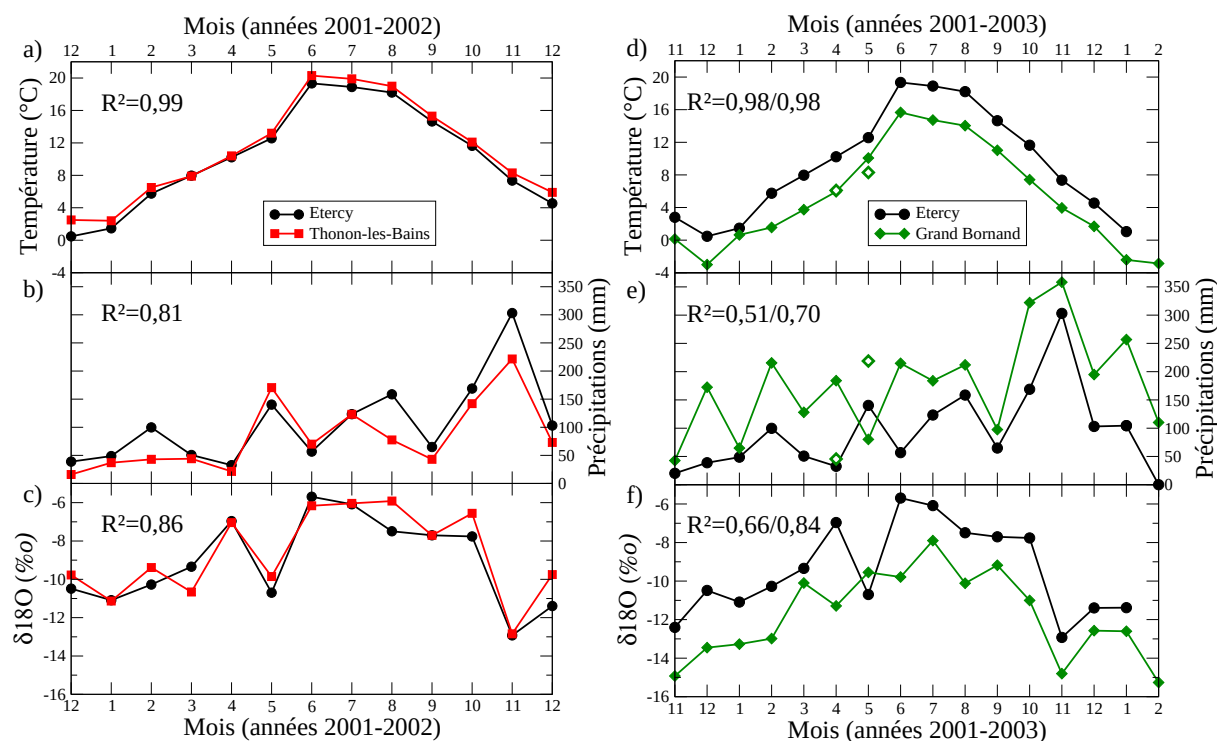
Figure 3.7: Température ( \pm 0,25^{\circ}C ) ( a et d ), précipitations ( \pm 0,1mm ) ( b et e ) et \delta^{18}O_P ( \pm 0,05\text{‰} ) ( c et f ) mensuelles aux stations d'Etercy, de Thonon-les-Bains et du Grand-Bornand de fin 2001 à début 2003. En d et e , les données des mois d'avril et de mai représentées par les losanges vides sont les moyennes mensuelles alors que les losanges pleins sont les moyennes du 1 Avril au 12 Mai et du 13 Mai au 30 Mai. Ces deux périodes correspondent aux périodes d'échantillonnage des précipitations à la station du Grand-Bornand (mesures isotopiques représentées par les losanges pleins en f ). En d , e et f , les deux coefficients de déterminations correspondent aux corrélations avec/sans les observations des mois 4 et 5 de l'années 2002.
