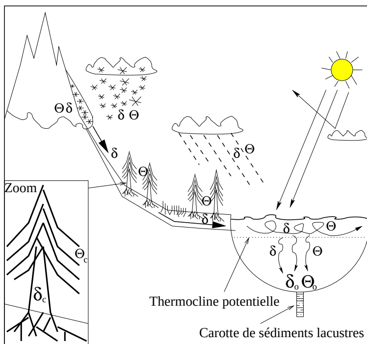
Figure 1.5: Schéma présentant les principales différentes origines de l'information isotopique (différents \delta ) et de l'information thermique (différents \Theta ) du signal isotopique enregistré dans les carbonates d'ostracodes benthiques préservés dans les sédiments ( \delta_o ) et du signal isotopique enregistré dans la cellulose des arbres ( \delta_c ).
