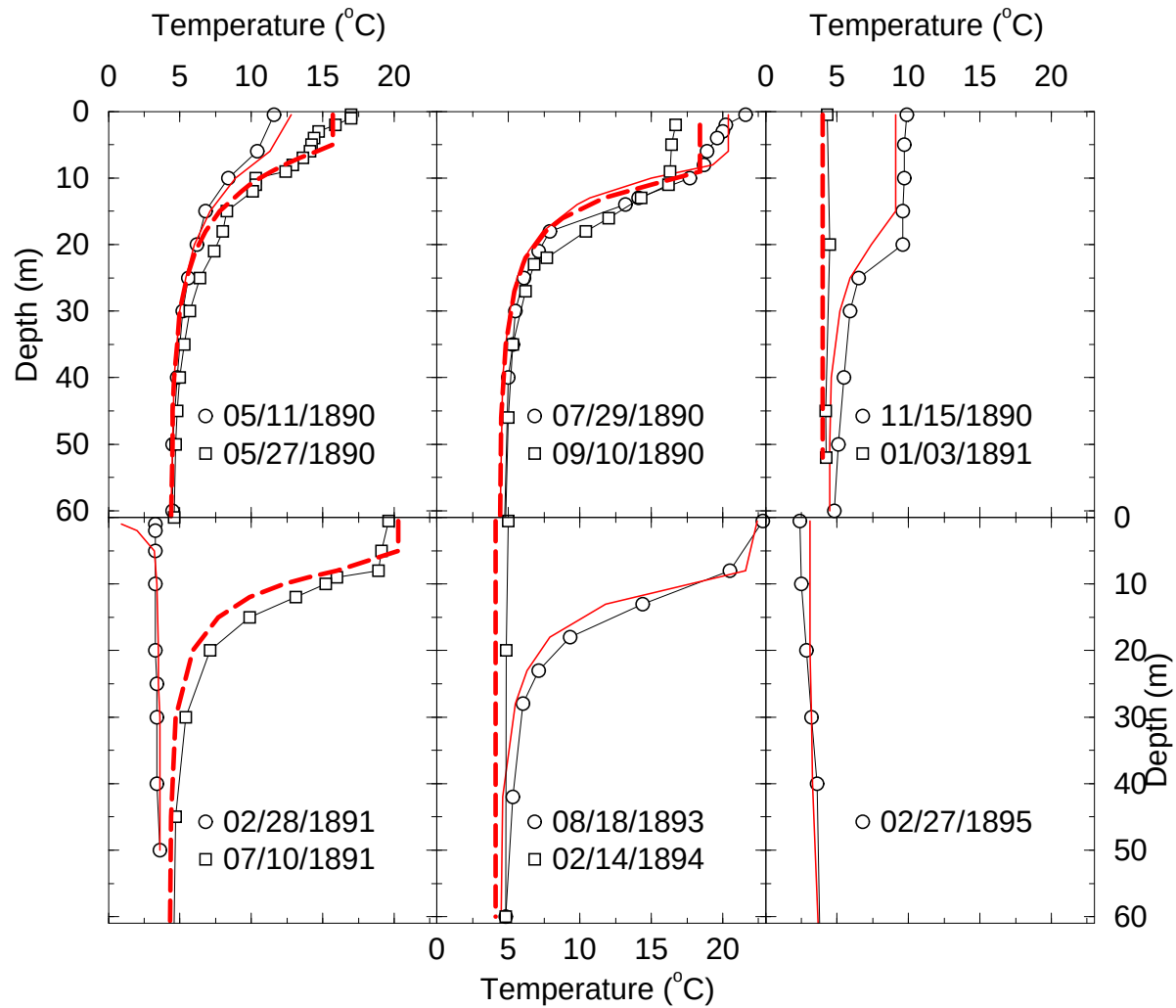
Figure 2.21: Observations historiques de la température du lac d'Annecy à la fin du XIX e siècle (symboles) [Delebecque, 1898]. Températures équivalentes simulées par le modèle (lignes). Les profils simulés expliquent 96% des profils observés (N=113).
