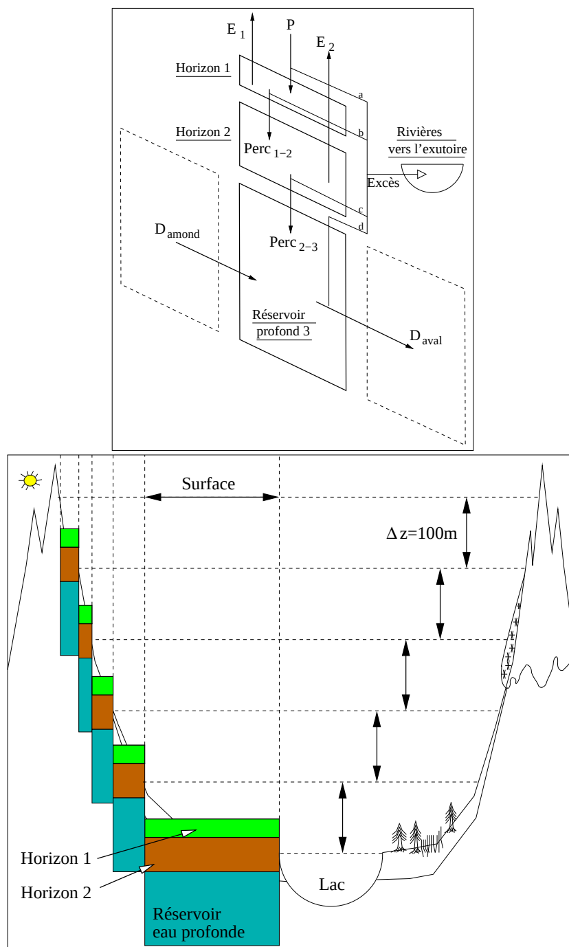
Figure 4.6: (Haut) Schéma des flux d'eau à l'échelle d'une maille altitudinale. P est la précipitation à la surface du sol qui se divise en infiltration dans sol-1 et en ruissellement vers les rivières pour l'excès d'eau qui ne peut être absorbé par le sol (flux a ). E_1 et E_2 sont les flux d'évapotranspiration à partir des horizons de sol 1 et 2. Perc_{1-2} et Perc_{2-3} sont les flux de percolation entre sol-1 et sol-2 , d'une part, et entre sol-2 et nappe-3 , d'autre part. D_{amont} et D_{aval} sont les flux d'eau latéraux entre les parties discrétisées du réservoir 3 d'eau profonde : gain depuis l'amont et perte vers l'aval. (Bas) Illustration de la discrétisation verticale du bassin versant par tranches de 100 m de dénivelé. Chaque maille altitudinale comprend trois réservoirs d'eau comme décrit sur la figure du haut. Les flux D_{aval} de la maille I est également dirigé vers les rivières.
