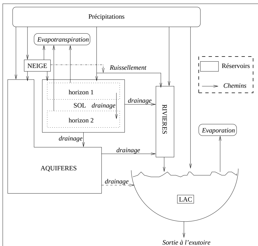
Figure 4.4: Schéma du cycle hydrologique d'un lac.
