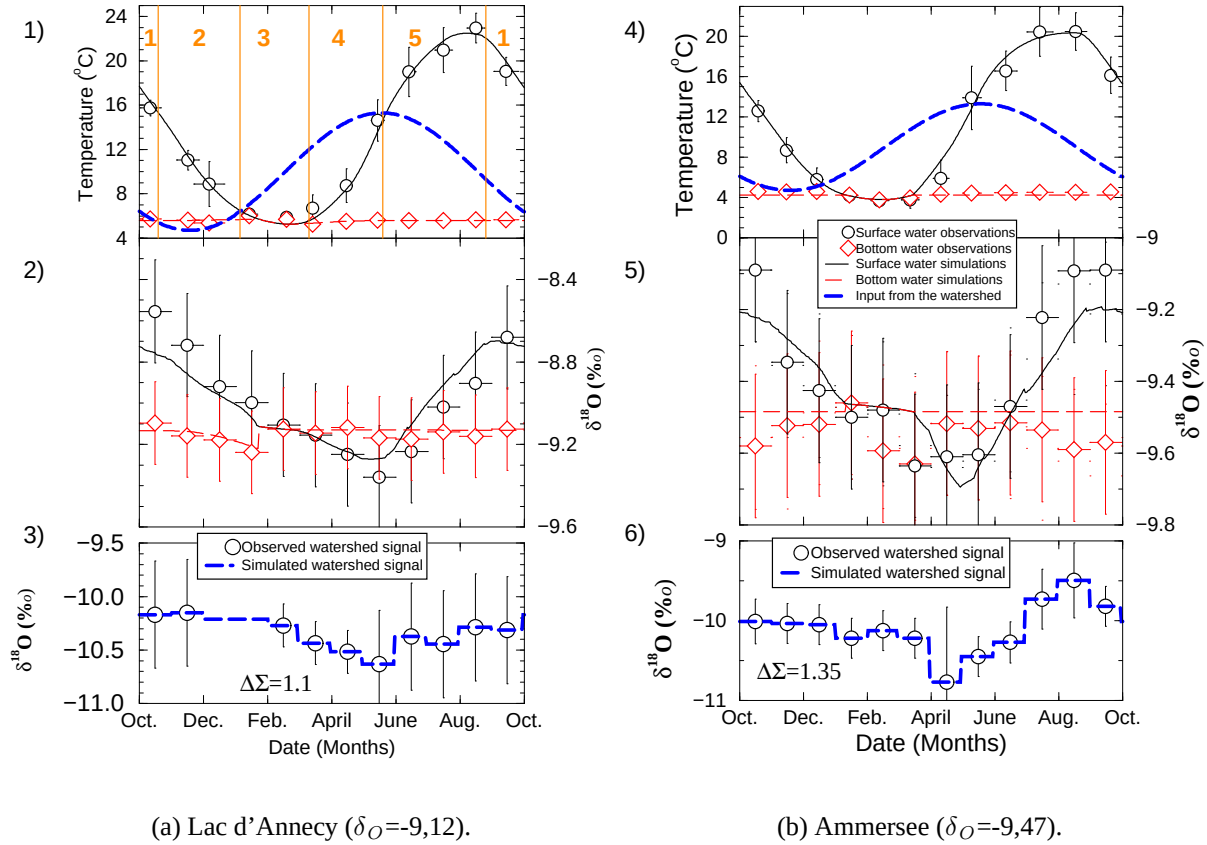
Figure 4.3: Résultats de la calibration climatologique du modèle isotopique de lac forcé par les observations hydro-isotopiques des bassin-versants. Lac d'Annecy : R^2=0,66 ; Ammersee : R^2=0,84
