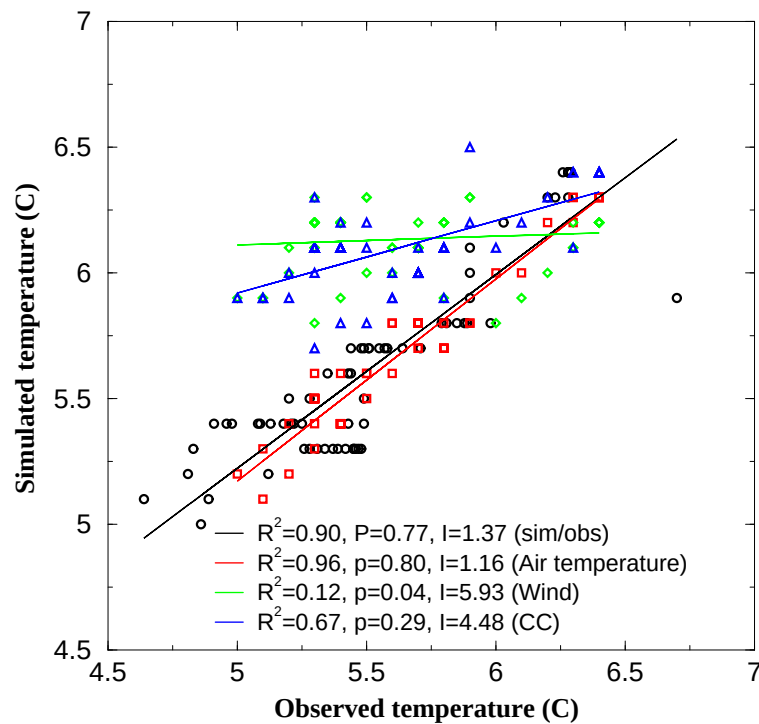
Figure 2.19: Corrélations entre observations et simulations des températures de surface et de fond à partir d'un forçage météorologique moyen mensuel (cercles noirs), d'un forçage moyen climatologique pour tous les paramètres sauf la température de l'air (carrés rouges) ou sauf la force du vent (losanges verts) ou sauf la couverture nuageuse (triangles bleus).
