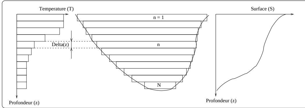
Figure 2.6: Illustration de la discrétisation verticale de la colonne d'eau lacustre.
