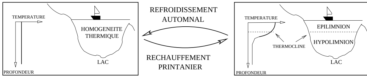
Figure 2.3: Schéma de la stratification et de l'homogénéisation thermique dans les lacs d'eau douce.
