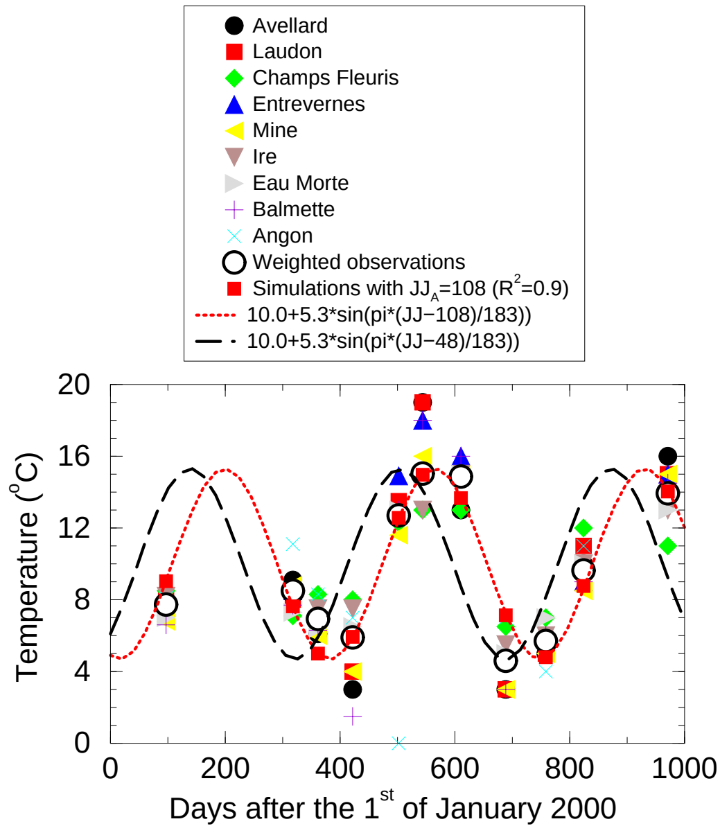
Figure 3.13: Observations et modélisation de la température des principales rivières du bassin versant du lac d'Annecy.
