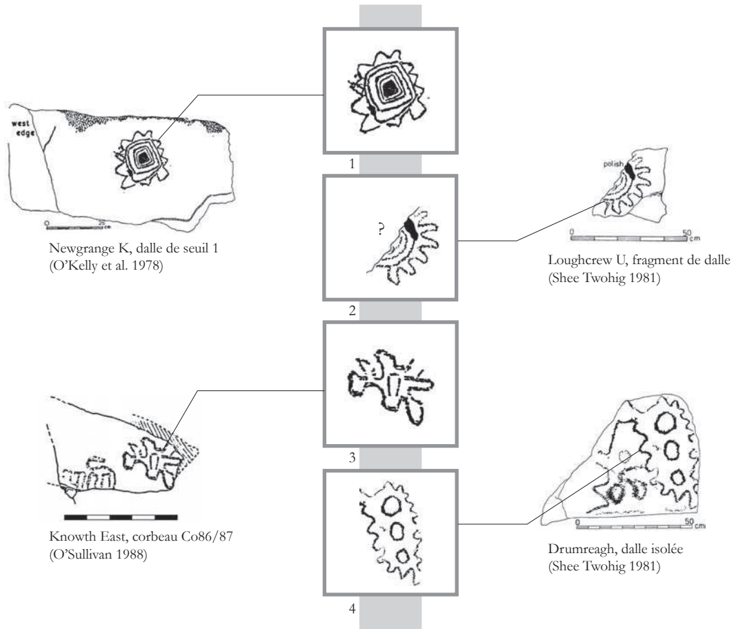
Figure 4.36 : Signes divers entourés par une ligne ondulée
