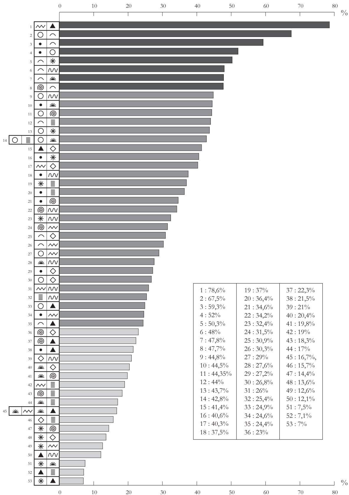
Figure 4.5 : Représentation graphique de la proportion des couples de signes
