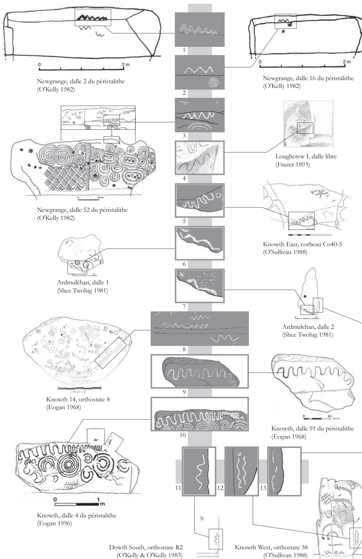
Figure 5.9 : Signes ondulés gravés le long d'une ligne de relief
