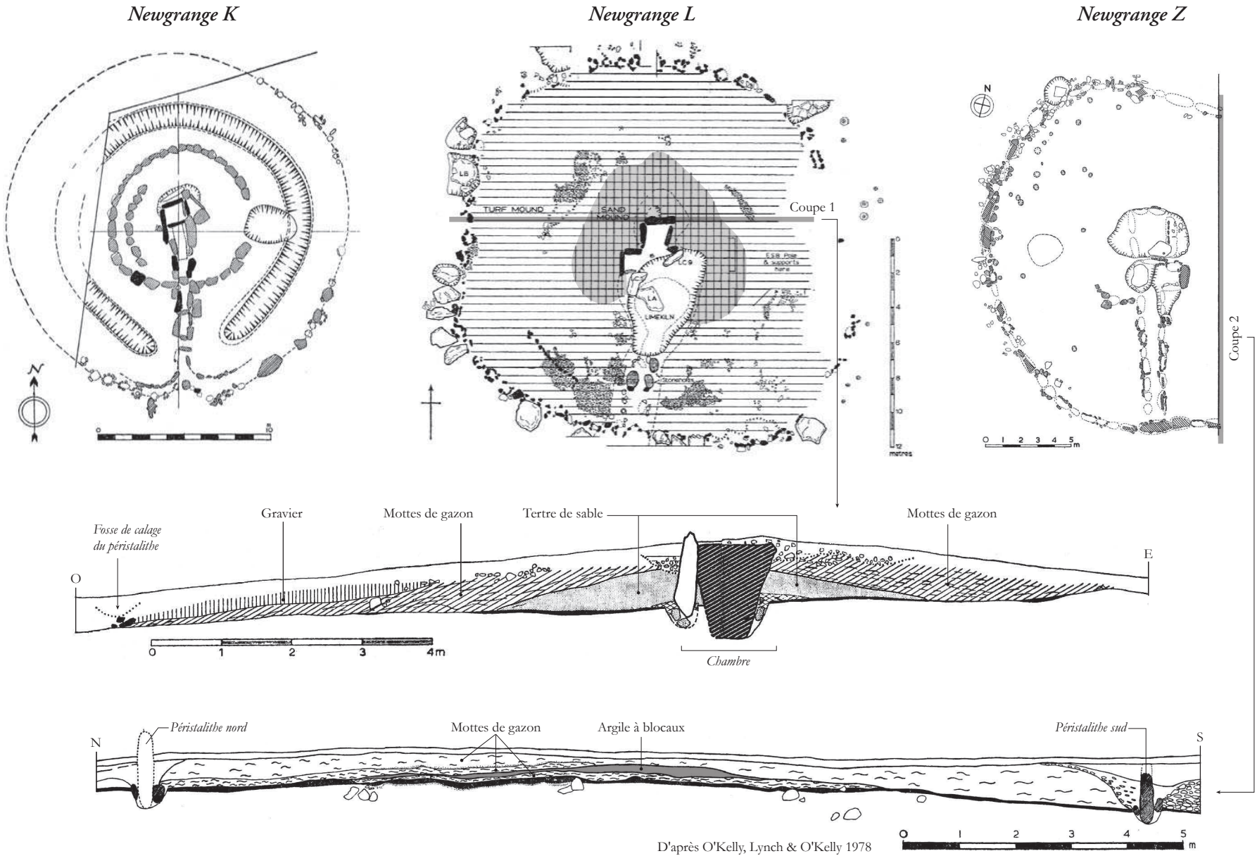
Figure 7.3 : Structures tumulaires de Newgrange K, L et Z
