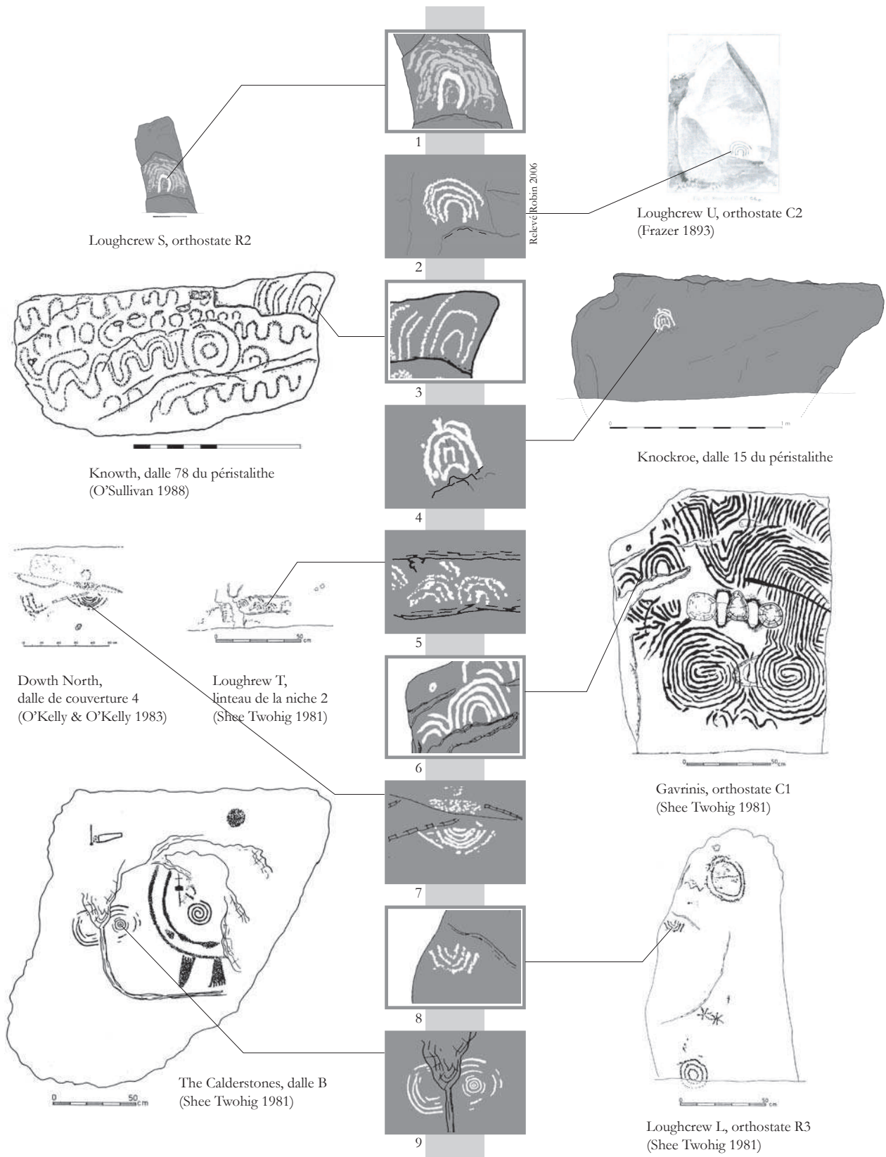
Figure 5.7 : Arceaux au contact d'une ligne de relief
