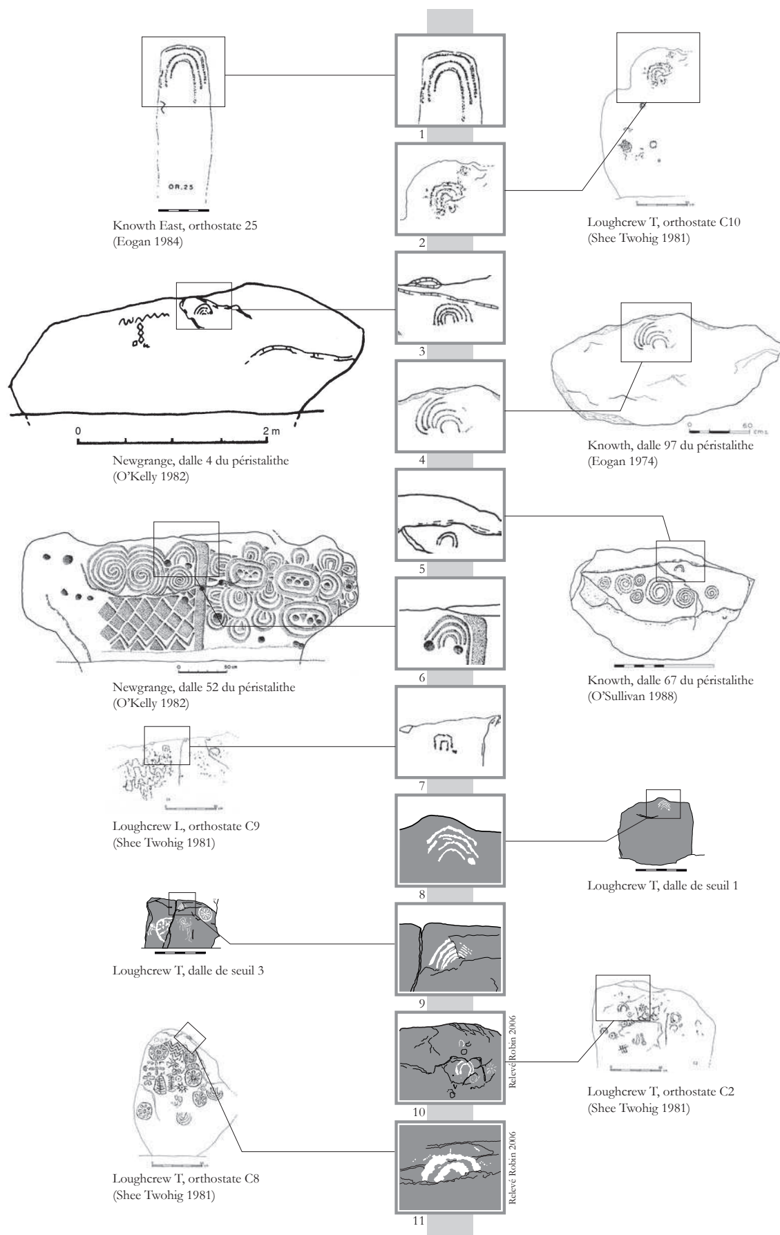
Figure 5.1 : Arceaux de type 2b en position sommitale
