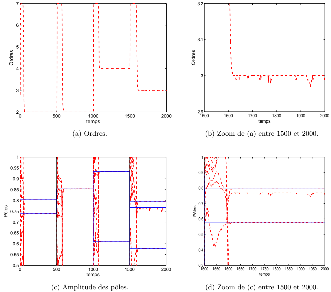
FIGURE 6.2 – Moyenne des estimées (ordres et pôles en pointillés rouge) obtenues par une simulation de Monte-Carlo de taille 100. Les modules des pôles du système réel sont tracés en trait plein bleu.
