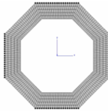
FIG. III-2.5 – Cellule octogonale
