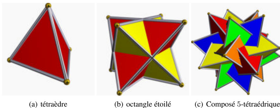
FIG. II-3.7 – Composés tétraédriques
