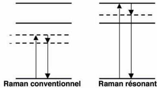
FIG. 2.6 – Schéma présentant les effets Raman conventionnel et résonant. Les lignes continues désignent des états électroniques réels et les lignes pointillées des états virtuels, c'est-à-dire qui ne sont pas des états propres du système.
