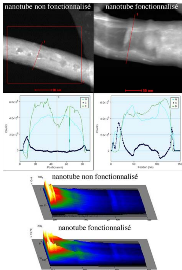
FIG. 4.16 – Images de champ sombre, profils de concentration de B, C et N et spectres lignes réalisés sur des nanotubes multifeuillets de type Chen non fonctionnalisé et fonctionnalisé par la quinuclidine.
