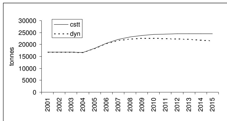
Figure 4. 14 : Evolution de la biomasse en tonnes dans le cas d'une amélioration de la sélectivité correspondant au scénario 2 à capacité de pêche constante (cstt) et lorsque la dynamique d'investissement est endogène (dyn).
