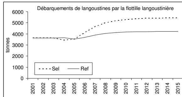
Figure 5. 5 : Débarquements de langoustine par la flottille langoustinière.
