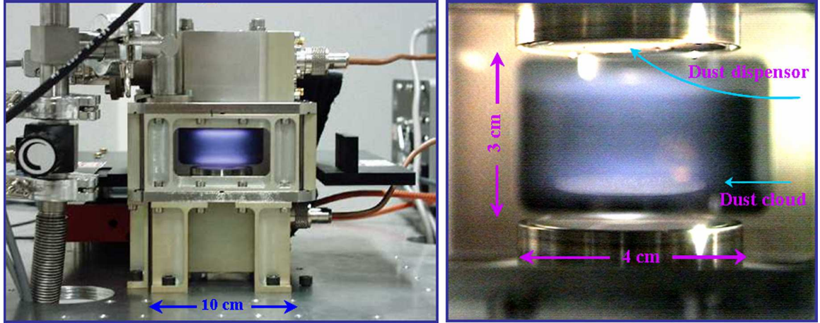
Figure II.2 Réacteur PKE : (a) vue générale, (b) vue de l'espace interélectrode avec un nuage de poussières en suspension au voisinage de la gaine inférieure.
