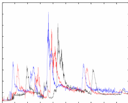
Figure 9 : répétition d'expériences chromatographiques. Trois expériences sont réalisées dans des conditions similaires. La superposition de leurs chromatogrammes révèle des variations du temps de rétention de l'ordre de la minute.
