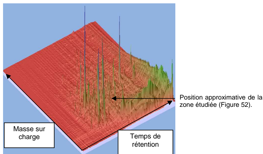
Figure 51 : exemple de spectrogramme obtenu. Cette image a été obtenue à partir du fichier global UF7376 en utilisant le logiciel de visualisation MSight du Swiss Institute of Bioinformatics.
