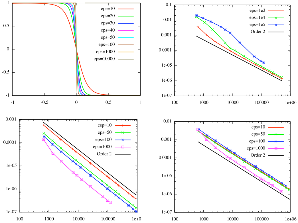
Figure 3.18: En haut à gauche, épaisseur du choc f_s en fonction du paramètre \varepsilon . En haut à droite, convergence asymptotique en norme L^2 sur la fonction f_s pour des valeurs très grandes de \varepsilon . En bas, convergence asymptotique en norme L^1 (à gauche) et norme L^2 (à droite) pour des valeurs raisonnables de \varepsilon .
