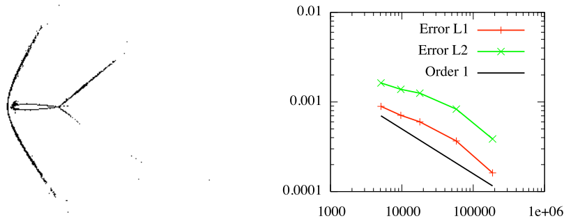
Figure 3.15: Écoulement supersonique autour du profil NACA0012. À gauche, iso-valeurs du nombre de Mach pour un maillage uniforme de 80 000 sommets. À droite, ordre de convergence spatial sur une suite de maillages uniformes en norme L^1 et L^2 .
