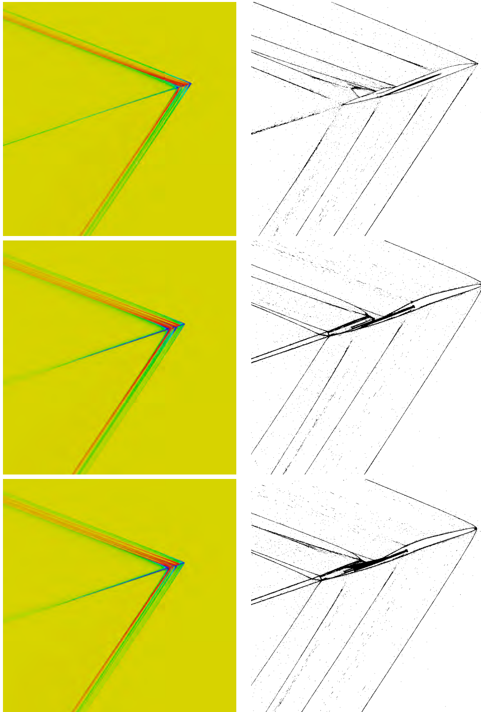
Figure 5.19: Coupe des maillages volumiques suivant le plan de symétrie Oxz pour chaque configuration. De haut en bas, les configurations SSBJ, low boom et low boom+dièdre.
