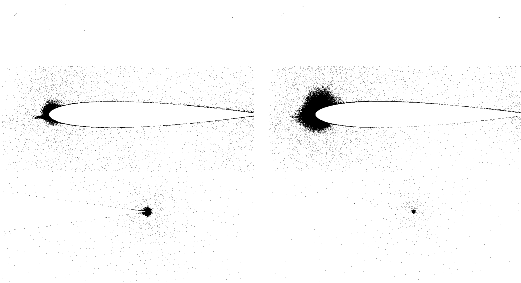
Figure 4.1: NACA0012 à Mach 0.63 et avec un angle d'attaque de 2 degrés. Comparaison des isolignes de pression et des maillages adaptés pour une adaptation sur la portance (à gauche) et sur la traînée (à droite). Les deux maillages comportent 80 000 sommets.
