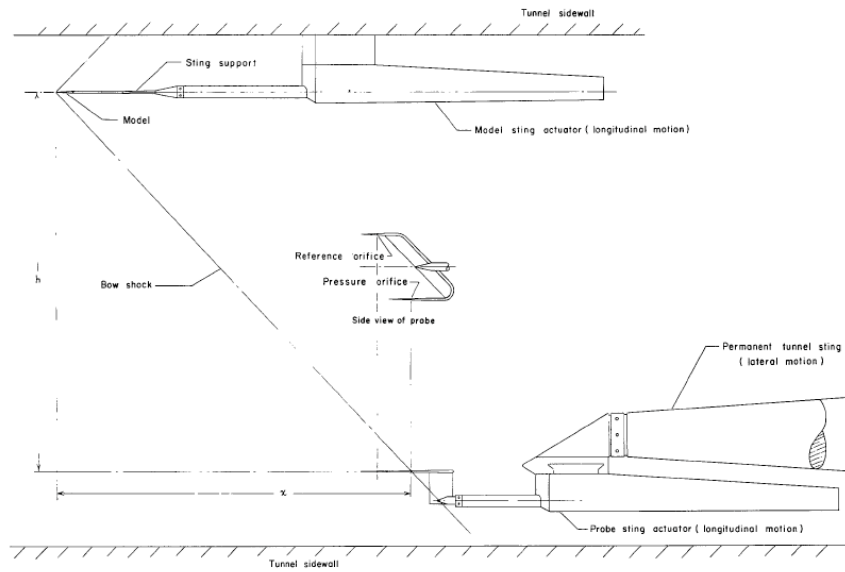
Figure 5.10: Représentation de la soufflerie supersonique utilisée dans [2].
