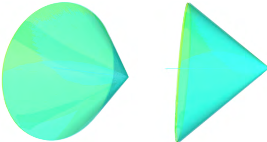
Figure 3.31: Jet d'affaire supersonique. Iso-surfaces du nombre de Mach qui représentent les cône de Mach émis par le jet dans tout le domaine de calcul. On notera que la solution n'est pas dissipée lors de la propagation des ondes de choc sur plusieurs kilomètres.
