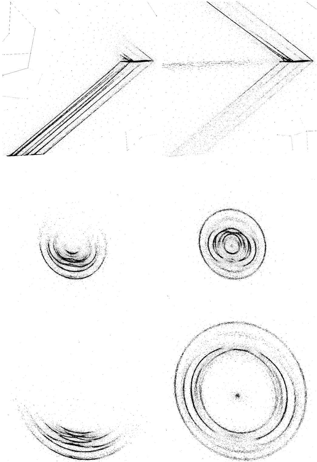
Figure 4.23: Coupes des maillages volumiques adaptés, cas adjoint à gauche et hessien à droite. Les plans de coupe (milieu et bas) sont donnés par la Figure 4.22 à gauche.
