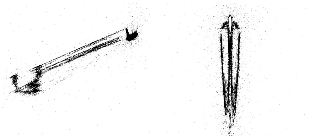
Figure 3.11: Simulation subsonique autour d'un Falcon à Mach 0.4 et pour un angle d'attaque de 10 degrés. Coupes volumiques dans le maillage final adapté comportant 2.5 millions de sommets. À gauche, coupe et vue de côté montrant l'anisotropie du maillage dans le sillage. À droite, coupe et vue au dessus de l'avion.
