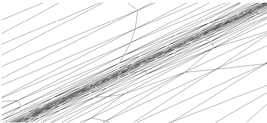
Figure 3.26: Zoom sur un des choc du maillage final adapté. On constate que l'anisotropie est cette fois préservée avec l'adaptation de maillage multi-échelles. Cette figure est à comparer à la Figure 3.3.
