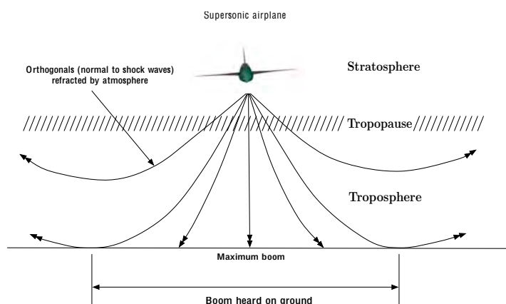
Figure 5.3: Illustrations du parcours des rayons acoustiques émis par l'avion. La région où ces rayons atteignent le sol est appelée carquette primaire.
