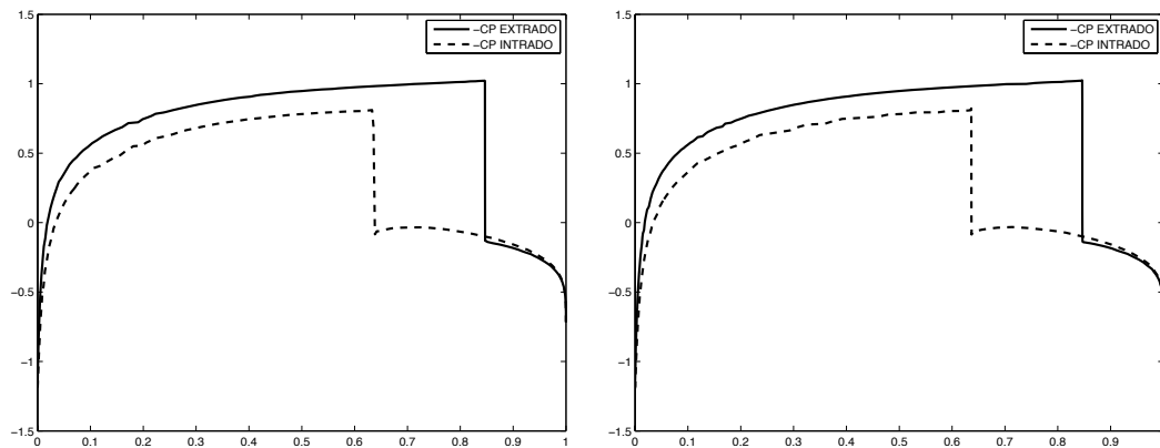
Figure 4.6: NACA0012 à Mach 0.85 et avec un angle d'attaque de 1 degré. A gauche, le cas test 5 et, à droite, le cas test 6. Représentation du coefficient de pression -C_p sur l'intrados et l'extrados du profil.
