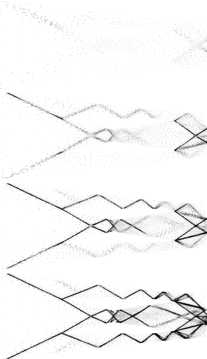
Figure 4.18: Maillages fins pour les quatre premières étapes du calcul adaptatif, i.e. , pour des complexités de 1000, 2000, 4000 et 8000 de haut en bas.
