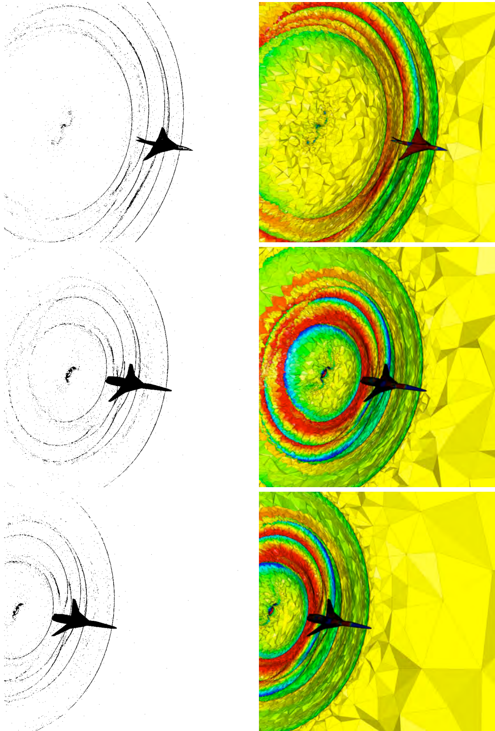
Figure 5.21: Coupe des maillages volumiques suivant le plan Oxy derrière chaque configuration. De haut en bas, les configurations SSBJ, low boom et low boom+dièdre.
