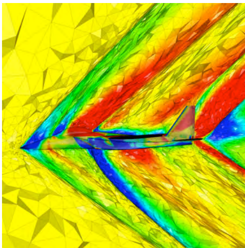
Coupe dans le maillage de calcul.
