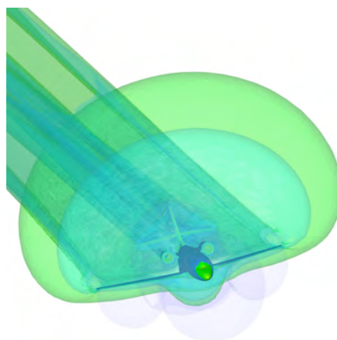
Iso-surfaces de la solution numérique.
