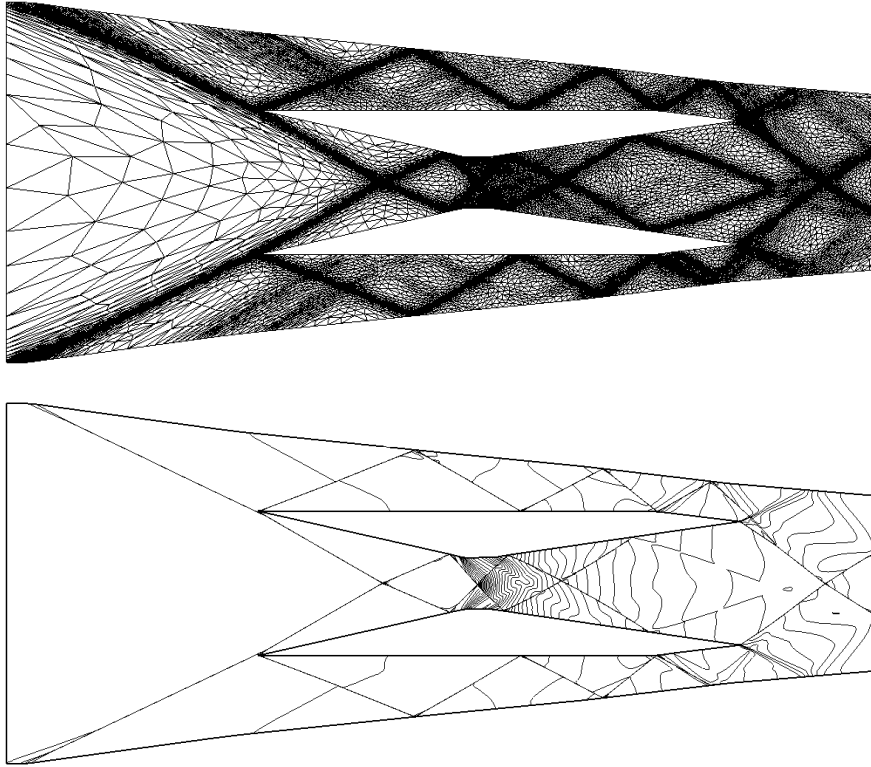
Figure 3.25: En haut, maillage final adapté en norme L^1 pour la simulation du scramjet contenant 22 566 sommets. En bas, les iso-valeurs de densité calculées sur ce maillage.
