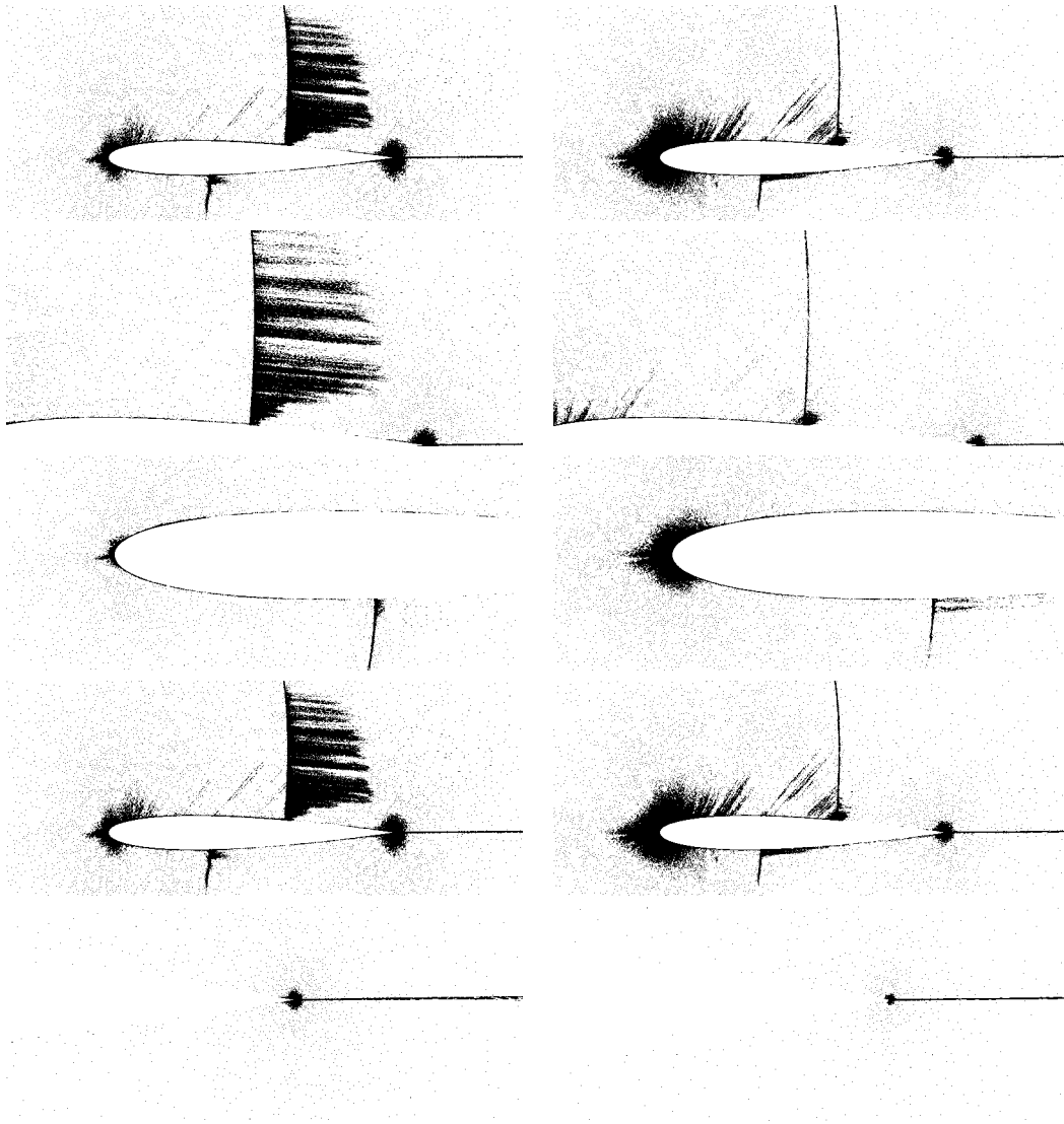
Figure 4.10: NACA0012 à Mach 0.8 et avec un angle d'attaque de 1.25 degrés. Représentation des maillages fins adaptés pour une adaptation sur la portance (à gauche) et sur la traînée (à droite). Les deux maillages comportent 80 000 sommets.
