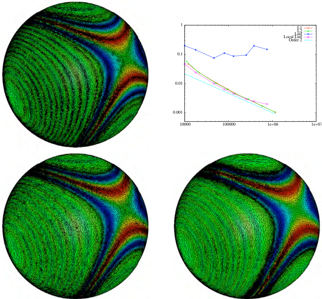
Figure 2.8: Maillages de surface adaptés minimisant l'erreur d'interpolation pour la fonction f_2 en norme \mathbf{L}^p avec p = [1, 2, \infty] . En haut à gauche, maillage en norme \mathbf{L}^1 , en bas à gauche, maillage en norme \mathbf{L}^2 et en bas à droite, maillage en norme \mathbf{L}^\infty . Chaque maillage est composé d'environ 245 000 sommets. En haut à droite, erreur d'interpolation pour chaque norme en fonction du nombre de points.
