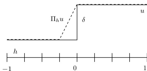
Figure 3.40: Représentation d'une marche 1D pour l'étude de la convergence des normes \mathbf{L}^p .
