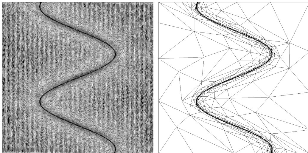
Figure 2.11: Maillages optimaux en norme \mathbf{L}^1 à gauche et \mathbf{L}^\infty à droite pour la fonction f_3 . Chaque maillage est composé d'environ 100 000 points.
