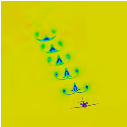
Turbulence numérique.
