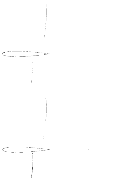
Figure 4.9: NACA0012 à Mach 0.85 et avec un angle d'attaque de 1 degré. Représentation des iso-lignes de pression pour une adaptation sur la portance (en haut) et sur la traînée (en bas). Les deux maillages comportent 80 000 sommets.
