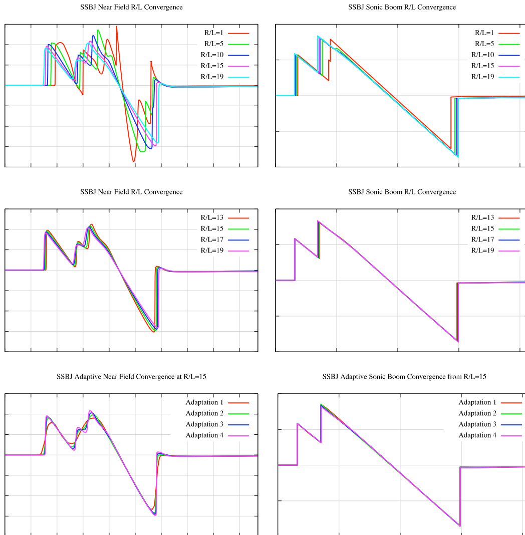
Figure 5.23: Signatures du champ proche de pression et bangs soniques associés pour le SSBJ. À gauche, on représente le champ proche \sqrt{R/L} \delta p en fonction de la position \mathbf{x} . À droite, on représente la pression en fonction du temps.
