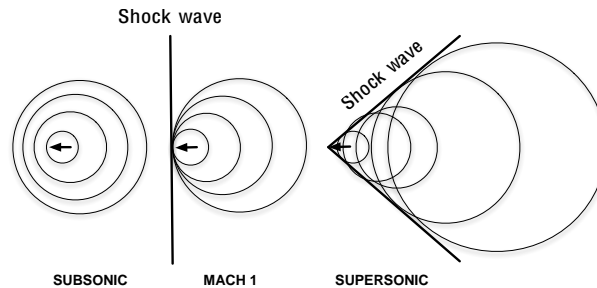
Figure 5.2: Signal acoustique dû à un objet mobile dans l'air. Lorsque l'objet dépasse la vitesse du son, les ondes acoustiques focalisent créant des ondes de choc. Elles forment un cône : le cône de Mach.
