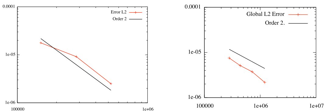
Figure 3.37: Courbe de convergence pour le nombre de Mach en norme L^2 . À gauche, pour le SSBJ, et à droite, pour le Falcon. Dans les deux cas, l'ordre deux théorique est atteint asymptotiquement.
