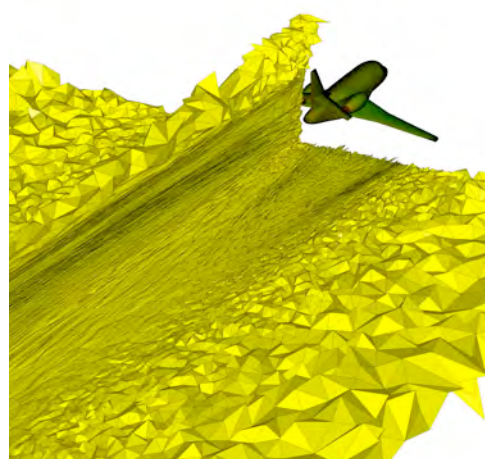
Représentation du maillage anisotrope adapté.
