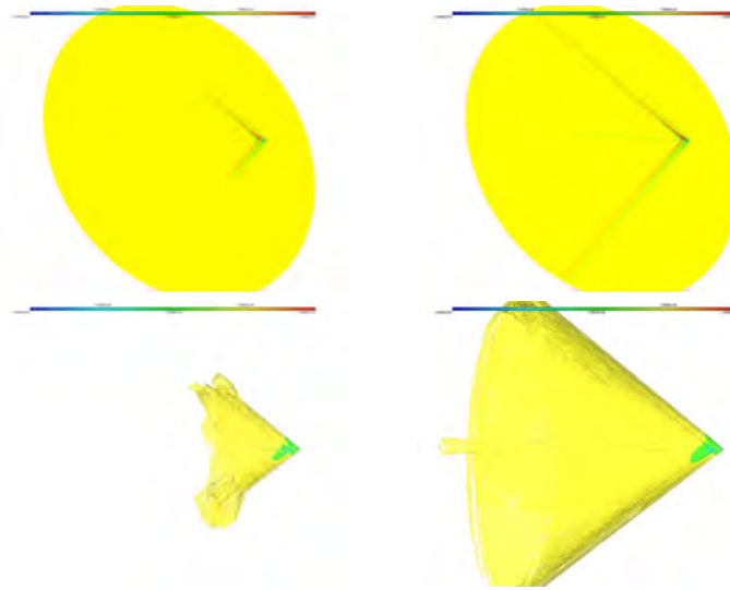
Figure 3.23: Comparaison d’une adaptation en norme L^\infty avec normalisation locale à gauche et d’une adaptation multi-échelles à droite. En haut, iso-valeurs du nombre de Mach. En bas, représentation du cône de Mach.
