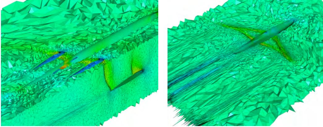
Figure 3.34: Jet d'affaire transsonique. Deux vues du maillage final adapté contenant 2025 231 sommets. On notera l'anisotropie du maillage à la fois pour le choc en lambda et pour le sillage de l'avion.
