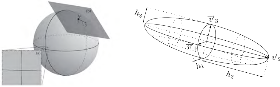
Figure 1.1: À gauche, la sphère est un exemple de variété riemannienne. En chaque point, il existe un plan tangent qui dépend de ce point, (a) et (b). Dans un plan (a), les propriétés métriques de la sphère sont approchées par les propriétés métriques du plan euclidien. À droite, représentation géométrique de la boule unité d'une métrique.
