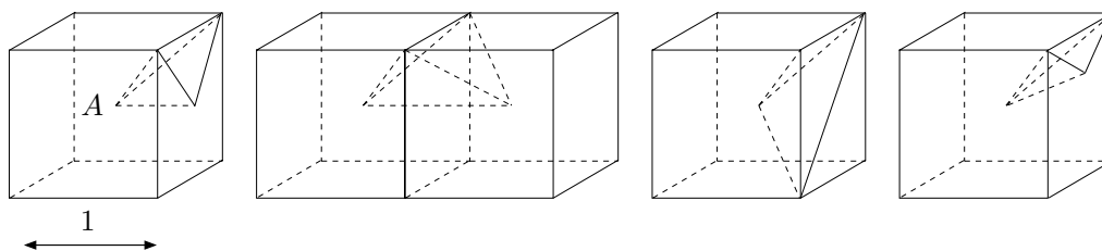
Figure 1.13: Tétrahédres de Sommerville 1, 2, 3, 4.
