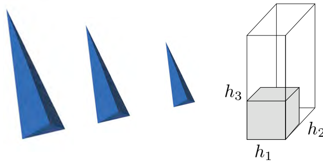
Figure 1.12: À gauche, différents éléments unitaires pour des métriques dont seulement la densité diffère. L'orientation et les quotients d'anisotropie sont conservés, seul le niveau de détail ou la précision est modifié. À droite, interprétation géométrique des quotients d'anisotropie en trois dimensions en terme de rapport de volumes.
