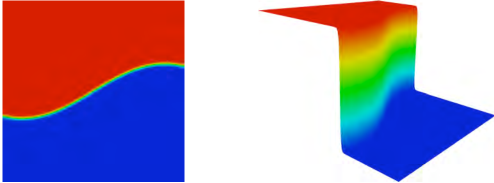
Figure 3.17: Modèle de choc C^\infty . À gauche, iso-valeurs de la fonction f_s , à droite, représentation en trois dimensions des valeurs de f_s
