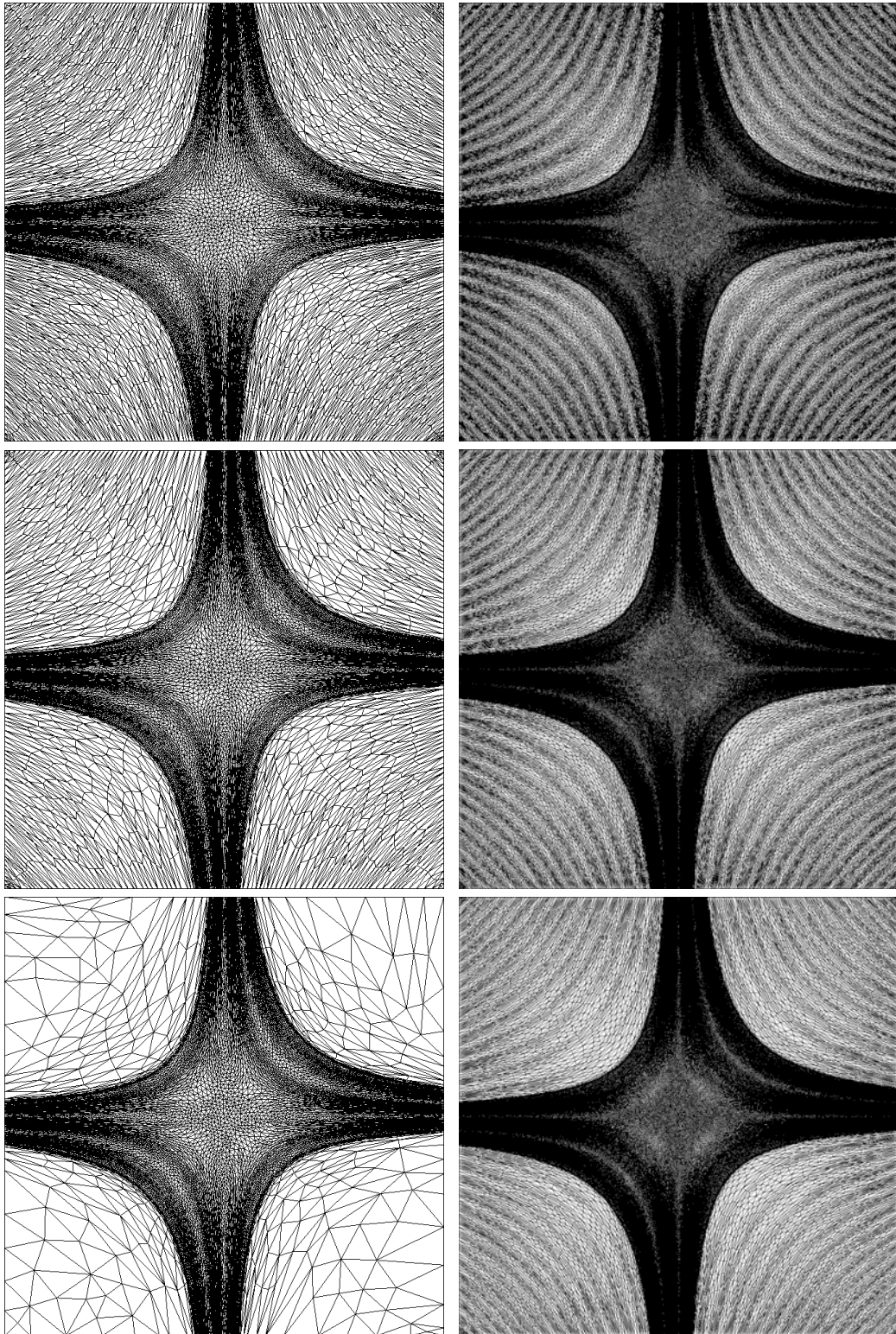
Figure 2.7: Maillages adaptés pour la fonction f_1 en norme \mathbf{L}^p avec p = [1, 2, 4] . Les maillages de gauche sont composés de 7 000 sommets et de 140 000 à droite. De haut en bas, maillages en norme \mathbf{L}^1 , \mathbf{L}^2 et \mathbf{L}^4 .
