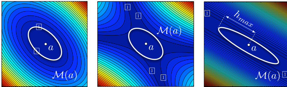
Figure A.3: Illustration de la boule unité de la métrique optimale lorsque H_e est quadratique : cas elliptique à gauche, hyperbolique au milieu et parabolique à droite. Dans ce dernier cas, une taille maximale h_{max} doit être choisie.
