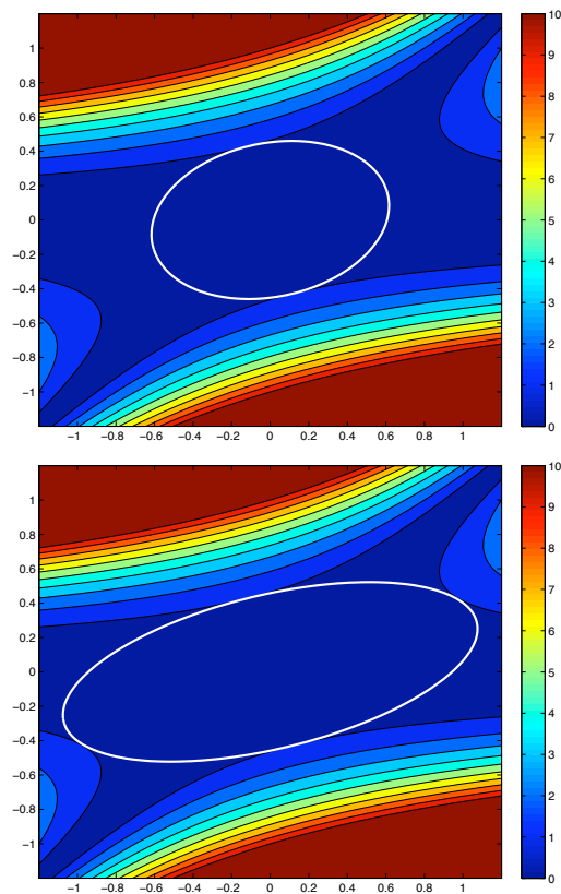
Figure A.7: Convergence vers la métrique optimale \mathcal{M}(\alpha_{opt}) pour le modèle d'erreur H_e = 10(xy^2 - y^3) . En haut, boule unité pour \mathcal{M}(0.5) et en bas boule unité pour \mathcal{M}(\alpha_{opt}) .
