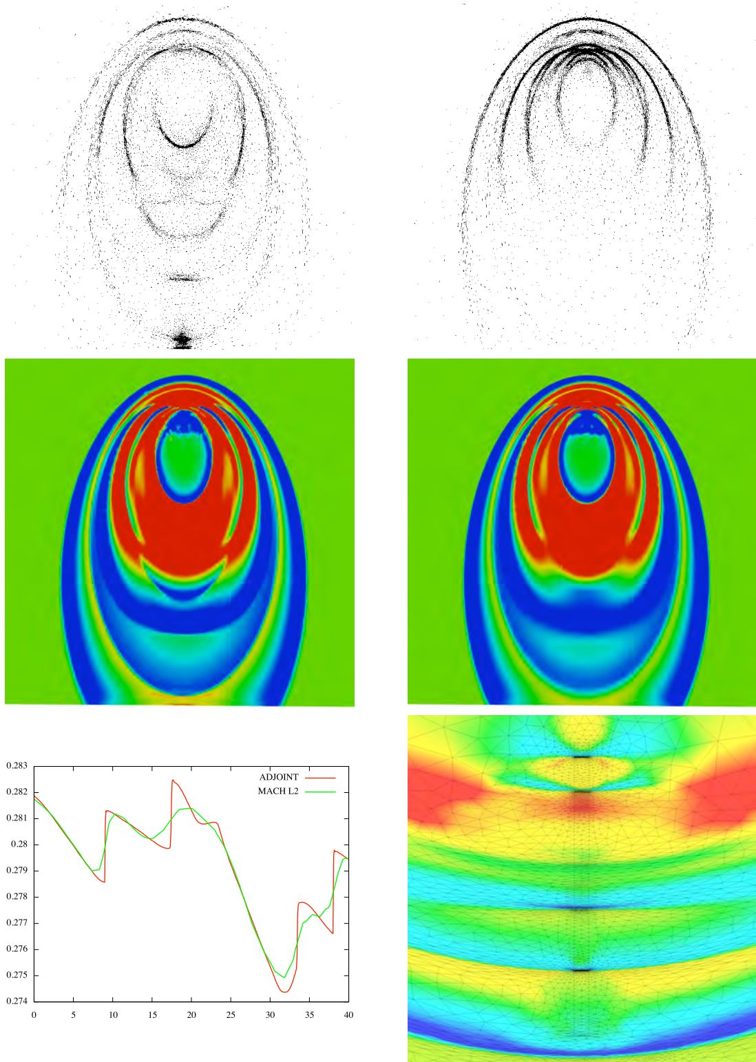
Figure 4.25: Coupes volumiques des maillages adaptés (haut) et nombre de Mach sur ces plans (milieu), pour les cas adjoint à gauche et hessian à droite. Le plan de coupe est donné par la Figure 4.22 à droite. En bas à gauche, coupe 1D suivant l'axe x dans le plan d'observation. En bas à droite, zoom sur le maillage de surface sur la zone d'observation.
