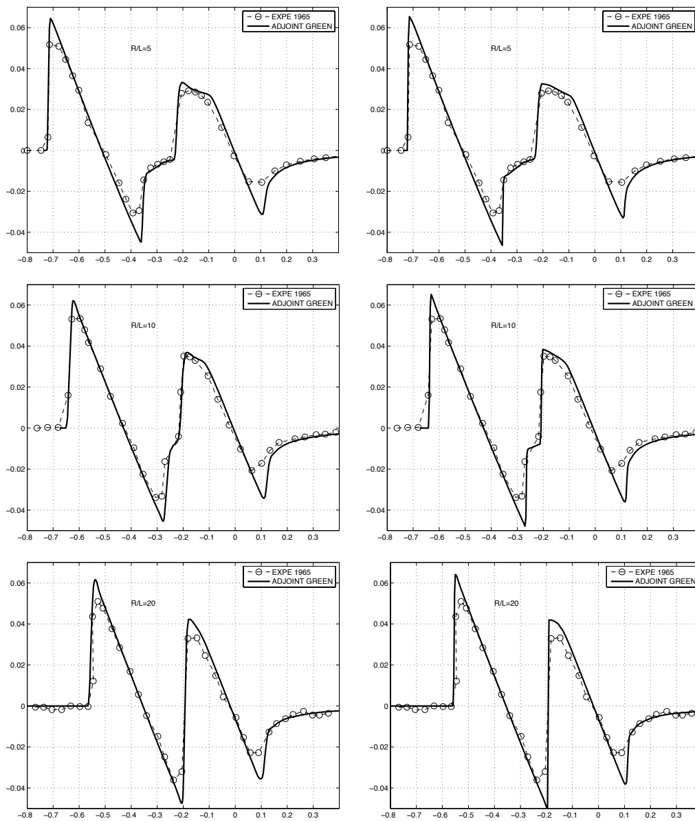
Figure 5.16: Adaptation de maillage basée sur l'adjoint (cas 6). On a utilisé le solveur HLLC, le schéma V_4 et la formule de Green pour la reconstruction du hessien. Signatures de pression obtenues sur les maillages adaptés comportant 2 millions de sommets (à gauche) et 4 millions sommets (à droite).
