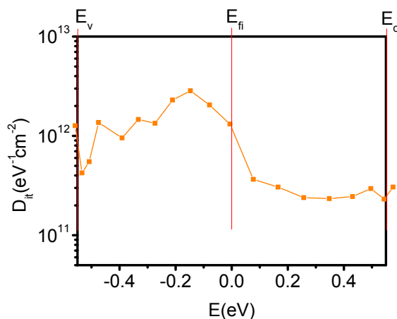
FIGURE 3.12: Répartition énergétique de la densité de défauts d'interface obtenue pour une structure FMIS avec de 4nm de silice, cette structure a subit un recuit sous N_2/H_2 à 425°C
