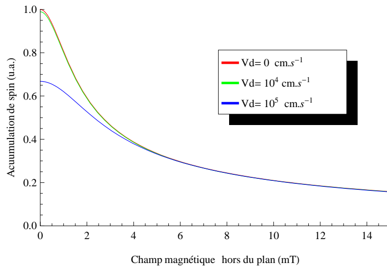
FIGURE 4.3: Calcul de l'effet de la vitesse de dérive non nulle sur l'effet Hanle (Amplitude normalisée pour v_d = 1000 \text{ cm.s}^{-1} )
