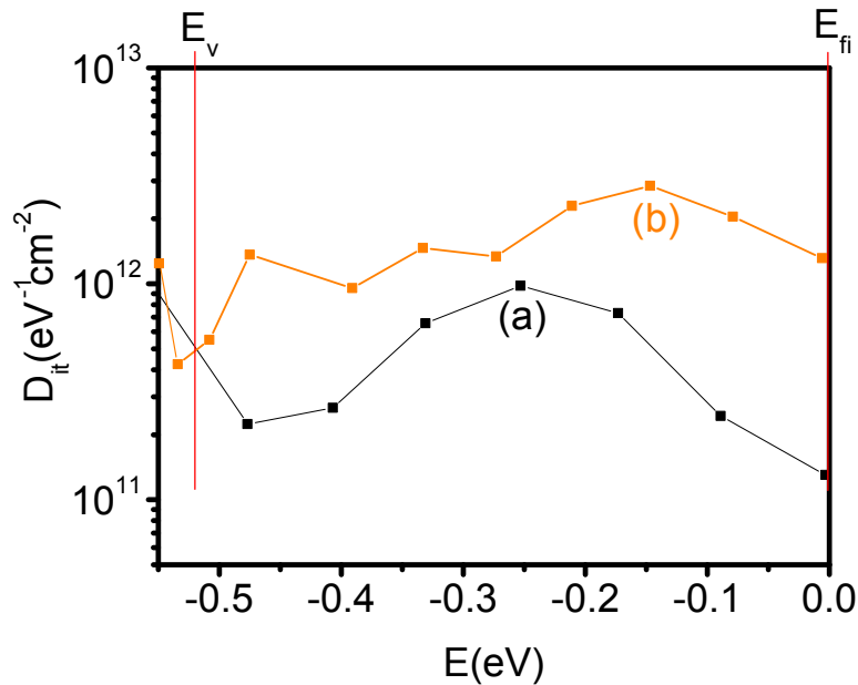
FIGURE 3.15: Répartition énergétique de la densités de défauts d'interface pour un échantillon de 4nm de silice avec recuit curatif (a) et sans recuit (b)
