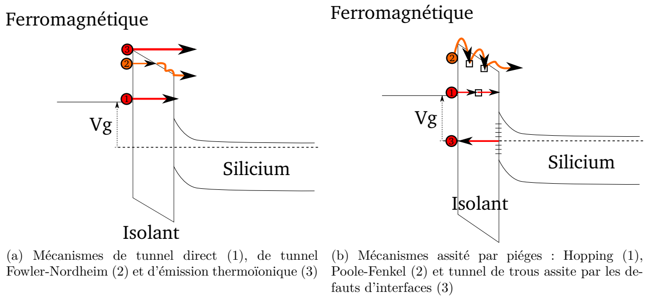
FIGURE 3.16: Mécanismes de transport dans une structure MIS
