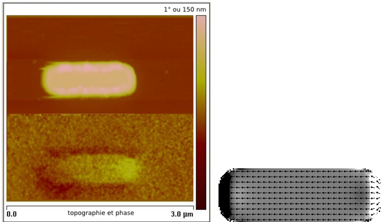
(a) Image de topographie (haut) et de phase d'un plot (bas) de 1.5 \mu\text{m} par 0.5 \mu\text{m} montrant une configuration monodomaine (b) simulation par différence finie de la divergence de l'aimantation
