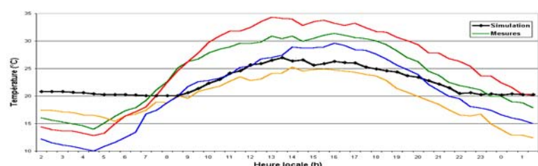
Figure 4 Comparaison entre les courbes de températures mesurées et calculées. Les courbes lisses représentent les températures
