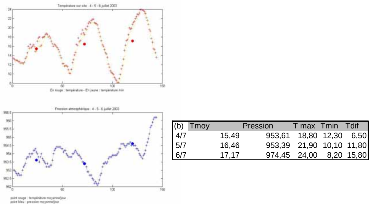
Figure 3.2.1 : (a) Données météorologiques : séries chronologiques (b) Données moyennes scalaires
