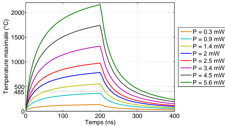
Figure 4.9 Évolution de la température au point chaud (coordonnées (r=0, z = -50 \text{ nm}) ) de l'empilement verre / ZnS-SiO 2 / InSb / ZnS-SiO 2 soumis à de excitations de puissance variable entre 0.1 mW et 5.6 mW.
