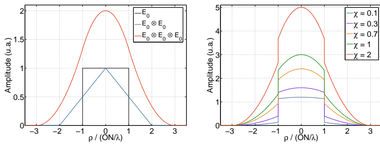
(a) Distribution du produit de convolution \tilde{E}_0(\rho) \otimes \tilde{E}_0^*(\rho) \otimes \tilde{E}_0(\rho) . Le terme résultant s'étale sur une distance trois fois plus importante que le terme \tilde{E}_0(\rho) .
