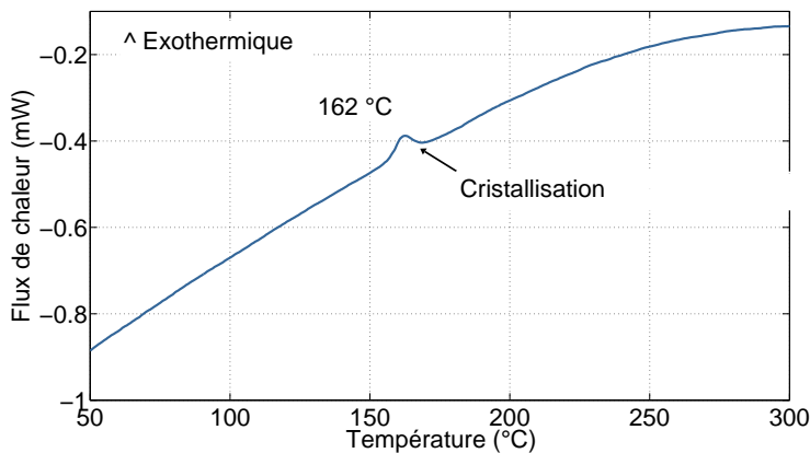
(a) Analyse thermique différentielle (DSC) sur une couche mince de 120 nm de InSb déposé par pulvérisation sur un substrat en silicium, chauffé avec une rampe de montée en température de 10^\circ\text{C}/\text{min} . La réaction exothermique observée à environ 160^\circ\text{C} traduit la cristallisation de la couche InSb.
