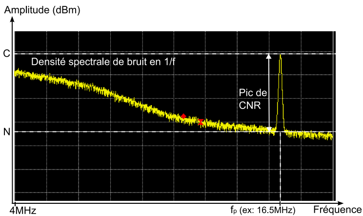
(b) Observation du signal à l'analyseur de spectre, laissant apparaître un pic de signal à la fréquence porteuse f_p , dont l'amplitude par rapport au niveau de bruit est définie comme le CNR ( Carrier to Noise Ratio ).
