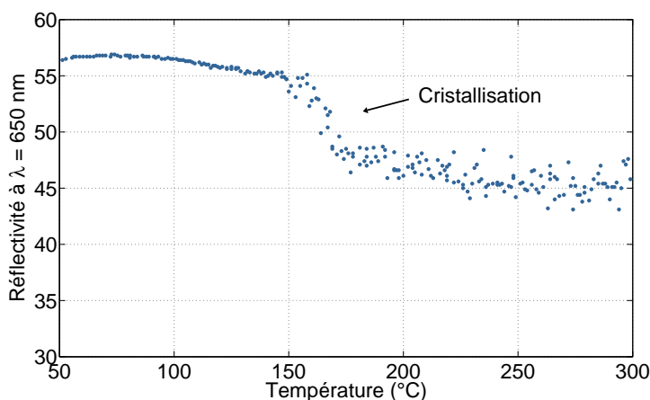
(b) Evolution de la réflectivité d'une couche mince (20 nm) de InSb avec la température (rampe de montée en température : 10^\circ\text{C}/\text{min} ). La chute de réflectivité due à la cristallisation de la couche observée autour de T = 160^\circ\text{C} .
