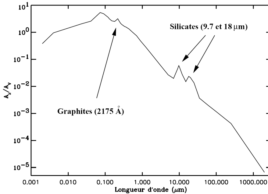
Figure I.9 – Loi d'extinction moyenne du milieu interstellaire de notre Galaxie (Mathis 1990). Extrait de la thèse d'Emeric Le Floch.
