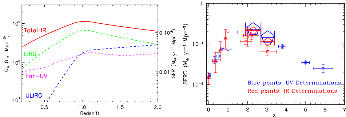
Figure I.13 – Evolution de la densité de formation stellaire avec le redshift (d'après Caputi et al. (2007); Tresse et al. (2007) (à gauche) et Reddy et al. (2008) (à droite)).
