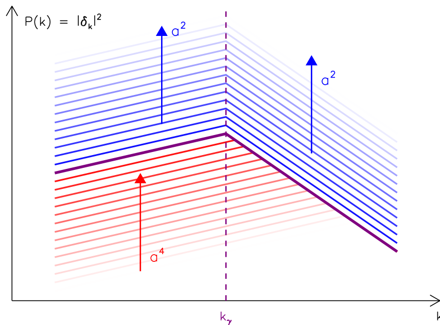
Figure I.3 – Evolution du spectre de puissance de la matière noire au cours du temps. En rouge, l'évolution au cours de la phase dominée par le rayonnement et en bleu, l'évolution au cours de la période dominée par la matière. En violet, on a le spectre de puissance au moment de l'égalité matière-rayonnement.
