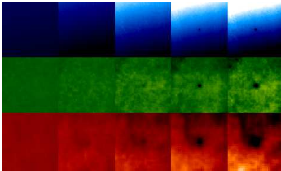
Figure IV.10 – Continus non uniforme obtenus pour chacune des 5 boîtes en flux S_{3.6} (des sources 3.6 \mu\text{m} les plus brillantes aux plus faibles) et à 24 , 70 et 160 \mu\text{m} (de haut en bas). Chaque image a une taille de 10' \times 10' .
