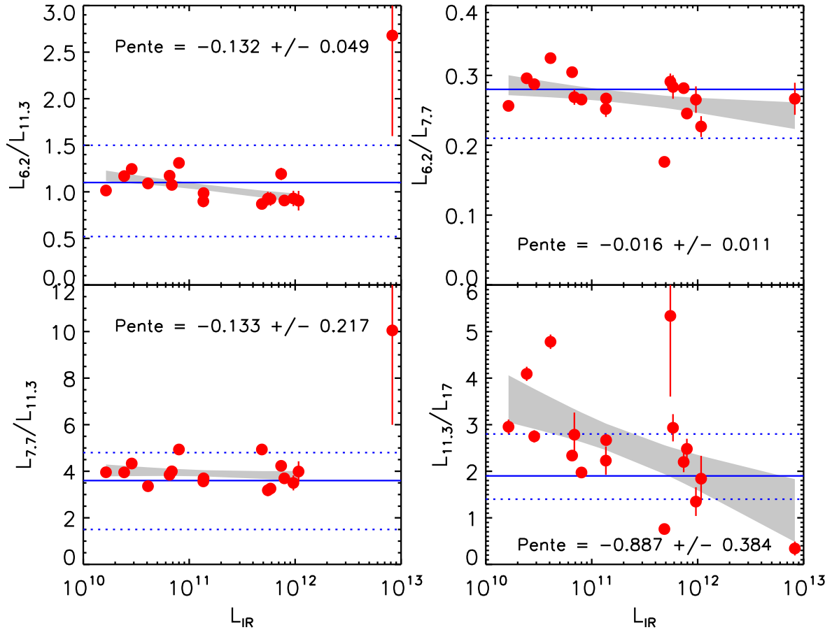
Figure V.19 – Variation des rapports entre différentes bandes de PAH en fonction de l'émission totale infrarouge pour les 17 galaxies de l'échantillon ModzSED. Les traits bleus horizontaux représentent la médiane (trait continu) et les quartiles à 10% et 90% (traits pointillés) mesurés par Smith et al. (2007) sur un échantillon local.
