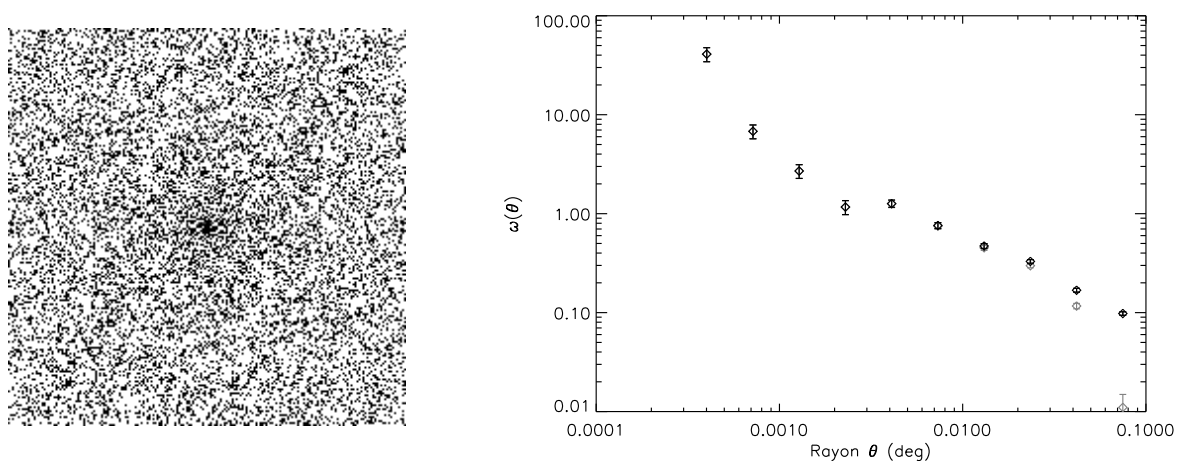
Figure III.4 – Illustration de la méthode d'estimation de la fonction de corrélation angulaire avec le stacking. Ceci a été réalisé sur une simulation où nous avons distribué 2000 sources dans une région de \sim 1^\circ \times 1^\circ . Le résultat du stacking est montré à gauche : on voit déjà clairement un excès au centre dû à la corrélation des sources. A droite, on montre la fonction de corrélation angulaire \omega(\theta) qui est le profil radial de l'image précédente divisée par la densité surfacique moyenne et à laquelle on a soustrait 1. Les points noirs sont corrigés des effets de bord et les points gris sont non corrigés : cette correction a un effet notable aux grandes échelles.
