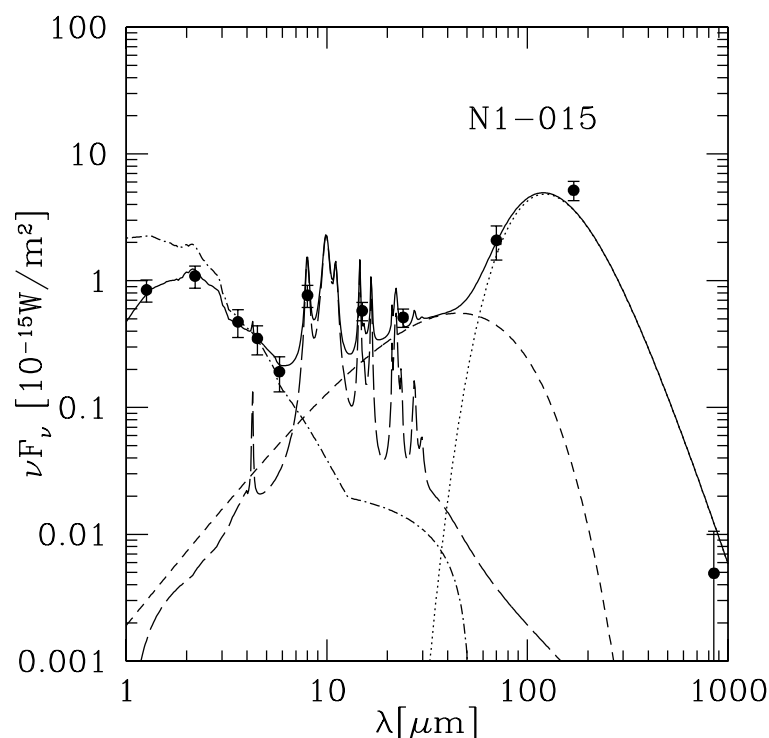
Figure I.10 – Contribution des différentes composantes de poussières à l'émission infrarouge d'une galaxie. L'émission des PAHs est représentée en tirets longs, celle des VSG est en tirets courts et celle des BG est en pointillés. La ligne pointillés-tirets représente l'émission des étoiles et la ligne noire continue est la somme de toutes ces composantes. Les points noirs sont les observations. Extrait de Sajina et al. (2006).
