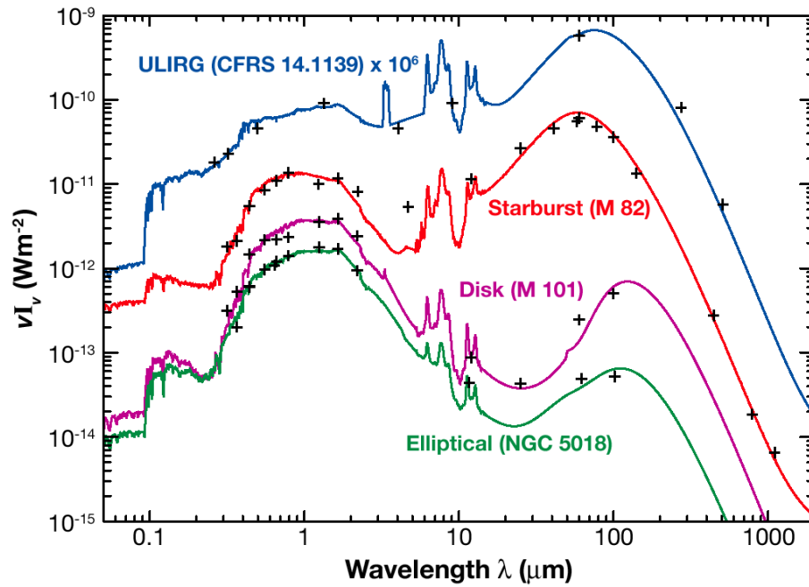
Figure I.11 – Distributions spectrales d'énergie de quatre galaxies représentatives depuis l'UV jusqu'au domaine millimétrique. Extrait de Lagache et al. (2005).
