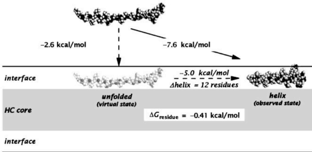
Figure 28 : Couplage partition/repliement de la méliittine dans une membrane de POPC. La formation de structures secondaires lors de la liaison à la membrane apporte une stabilité de 5 \text{ kcal}\cdot\text{mol}^{-1} , soit environ 0,41 \text{ kcal}\cdot\text{mol}^{-1} par résidu. D'après White & Wimley, 1999.
