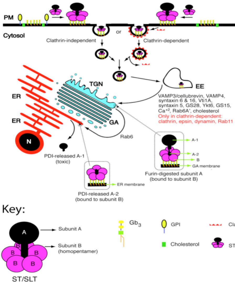
Figure 15 : Internalisation et trafic intracellulaire des toxines de Shiga et de type Shiga. EE, endosome précoce (EE pour « early endosome ») ; ER, réticulum endoplasmique ; ERAD, système de dégradation associé au réticulum endoplasmique ; GA, appareil de Golgi ; GPI, protéine ancrée au GPI ; N, noyau ; PDI, protéine disulfure isomérase ; PM, membrane plasmique ; ST, toxine de Shiga ; SLT, toxine de type Shiga ; TGN, réseau trans -golgien.
