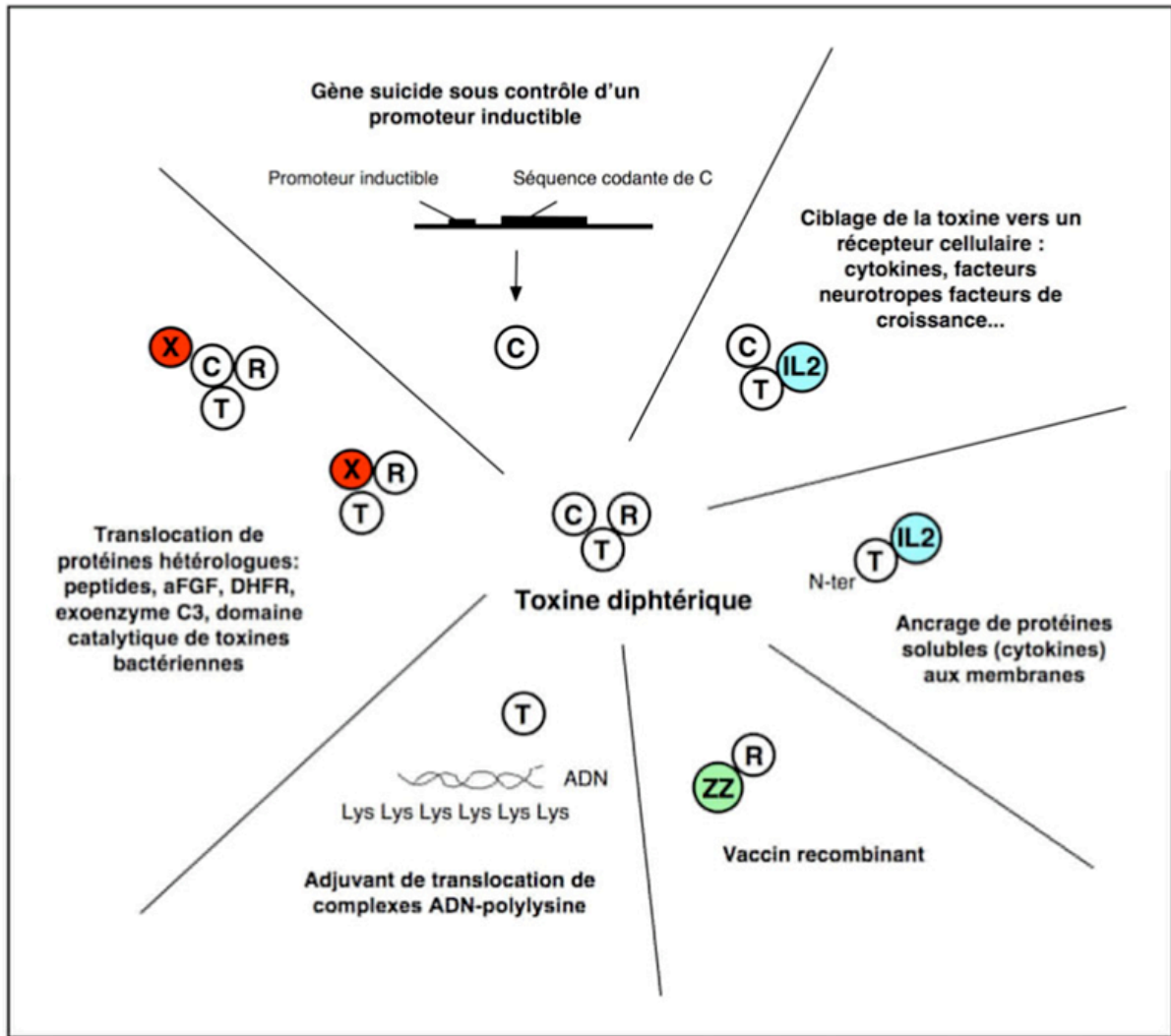
Figure 51 : Utilisation biotechnologique de la DT.
