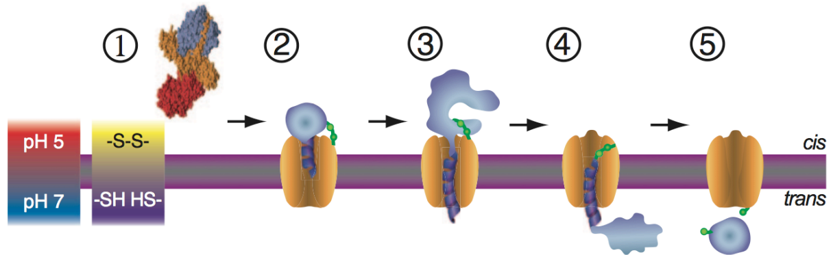
Figure 33 : Modèle de translocation du domaine catalytique de la BoNT à travers son composant B. (1) Structure cristallographique de la BoNT/A avant l'insertion dans la membrane. (2) Insertion de la BoNT/A dans la membrane, (3) et (4) étapes transitoires de translocation dans la membrane, (5) étape de libération du composant A dans le cytosol. Les conditions expérimentales miment la membrane des endosomes et leur environnement aqueux. D'après Fisher & Montal, 2007.
