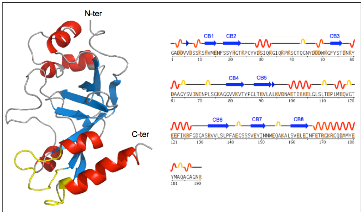
Figure 40 : Structure du domaine catalytique de la DT à pH 5 et séquence (PDB : 1DTP). Les hélices sont représentées en rouge et les brins \beta (CB) en bleu. Dans la structure, les deux boucles 66-78 et 169-176, dont le positionnement est différent par rapport à leur positionnement dans le domaine C dans la DT observée à pH 7,5, sont représentées en jaune. Les résidus chargés sont surlignés en orange. D'après Weiss et al. 1995.
