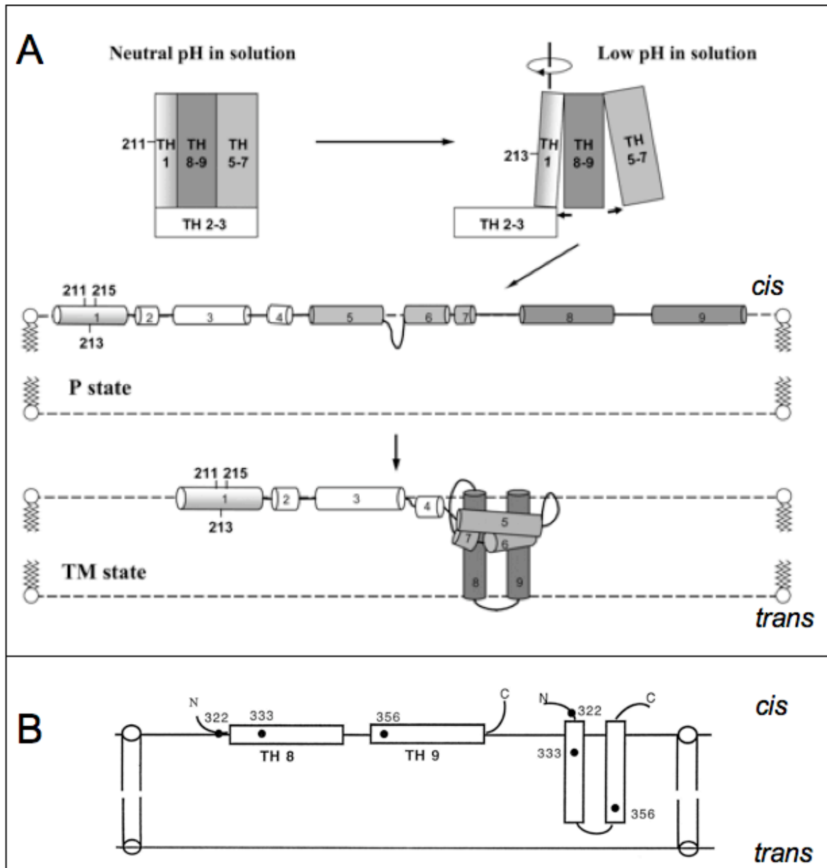
Figure 43 : Topologie du domaine T de la toxine diphtérique inséré dans les membranes selon les états P et TM. (A) Conformations du domaine T dans les membranes dans les états P (conformation à la surface de la membrane) et TM (conformation transmembranaire). D'après Wang et al. , 2006. (B) Localisation des mutations ayant permis d'identifier les positions des hélices TH8 et TH9. D'après Wang et al. , 1997b.
