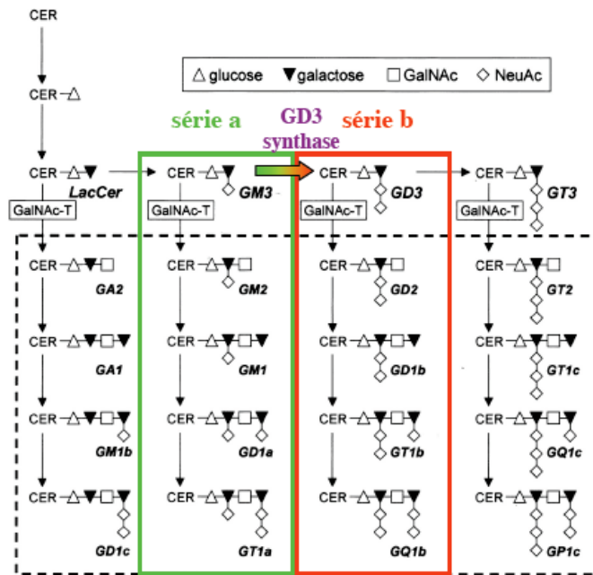
Figure 6 : Schéma de la synthèse des gangliosides. CER : céramide ; GalNAc : N -acétylgalactosamine ; LacCer : lactosylcéramide ; NeuAc : acide sialique ou neuraminique. La mutation de la N -acétylgalactosaminyl-transférase (GalNAc-T) est à l'origine de l'absence des gangliosides complexes compris dans le rectangle en pointillé. D'après Bullens et al. , 2006.
