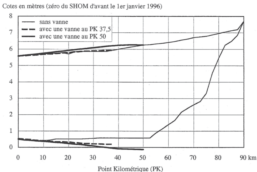
Figure 11 - Modélisation de la modification des niveaux de pleine mer et de basse mer par l'implantation, dans la partie médiane de l'estuaire de la Loire, d'une vanne régulatrice du niveau de basse mer.
