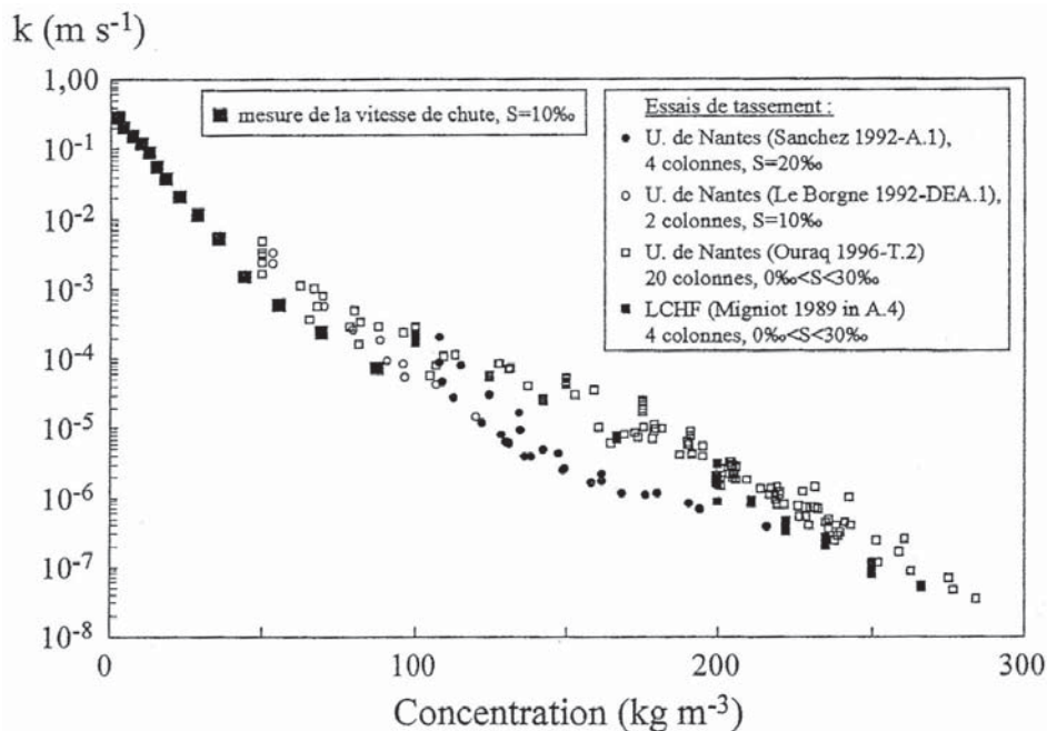
Figure 3 - Variation du coefficient de perméabilité en fonction de la concentration C pour des vases de l'estuaire de la Loire et pour différentes salinités S .
