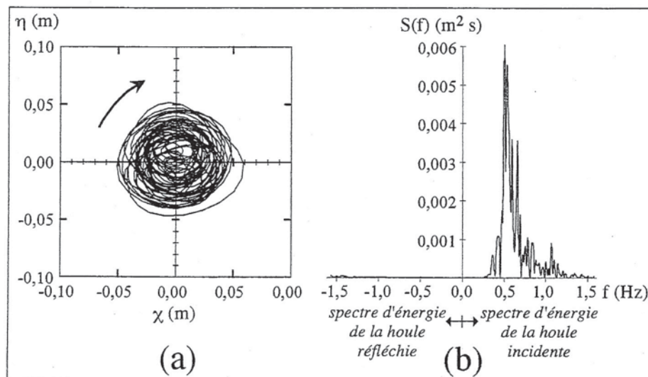
Figure 28 - Résultats correspondant à l'essai n° 12 (houle irrégulière avec une fréquence spectral pic de 0,5 Hz). (a) Trajectoire dans le plan \chi - \eta . (b) Spectre d'énergie de F=\eta+i\chi .
