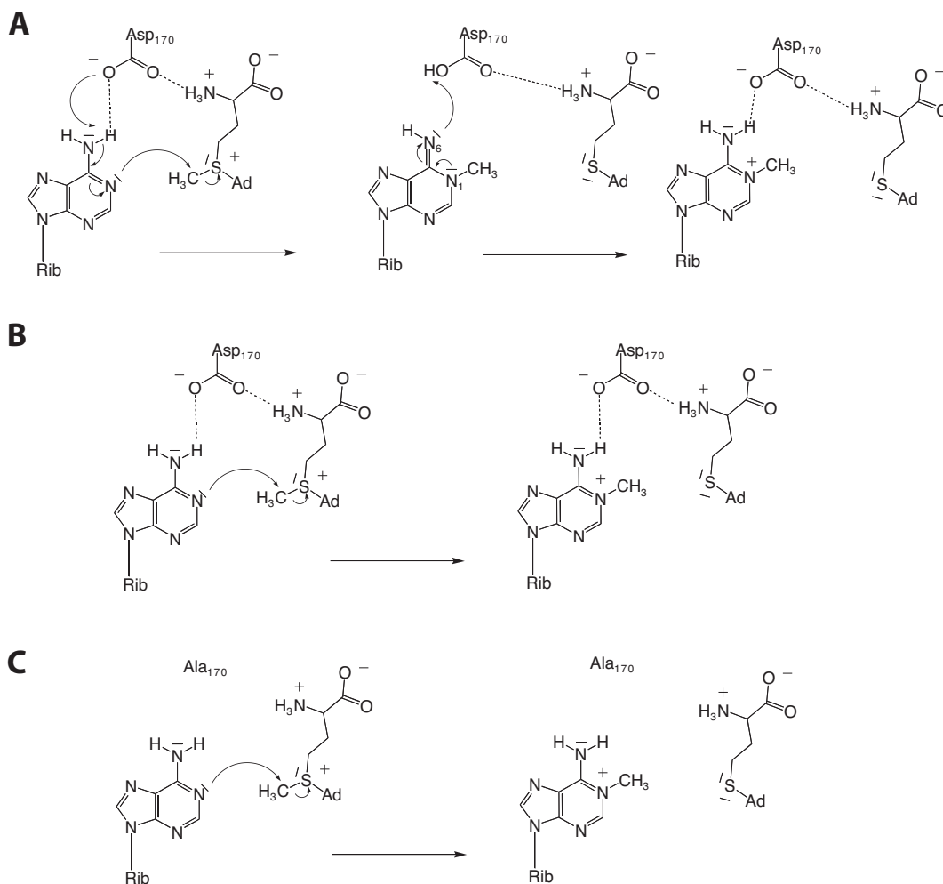
FIGURE 7.3 – Mécanismes possibles pour la formation du m 1 A
