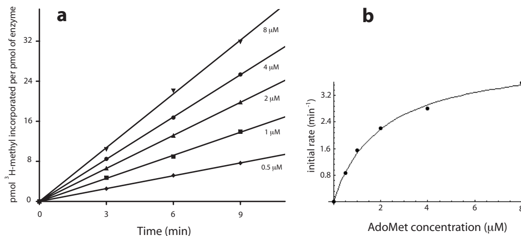
FIGURE 7.2 – Détermination des paramètres cinétiques k_{cat} et K_M Exemple de l'enzyme TrmI sauvage. a : Cinétique d'incorporation du 3 H-méthyle dans l'ARNt f Met pour différentes concentrations de SAM (0.5, 1, 2, 4, 8 μM). b : Fit des vitesses initiales d'incorporation à l'équation de Michaelis et Menten :
