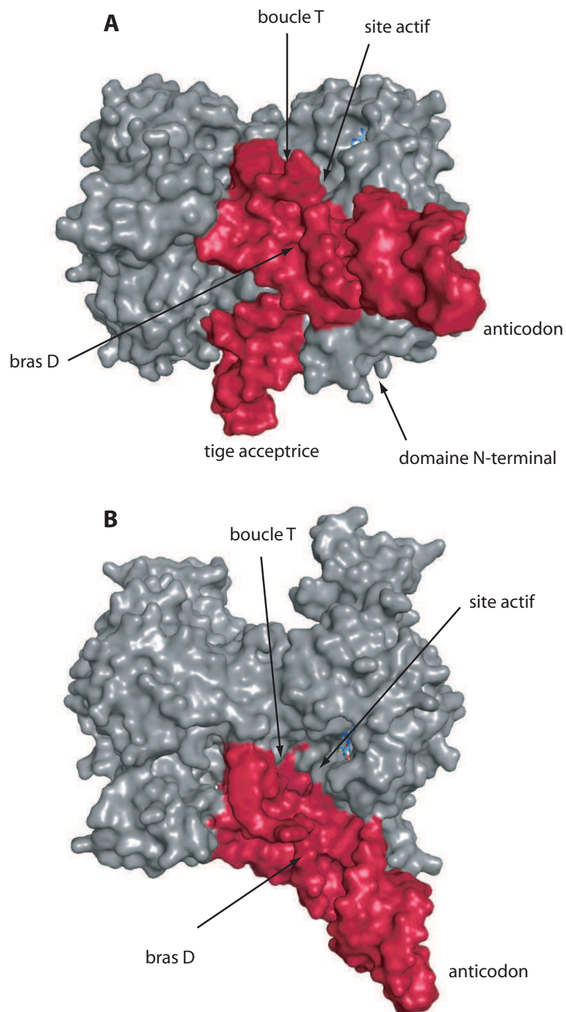
FIGURE 8.2 – Modèle d’amarrage manuel d’un ARNt entier
