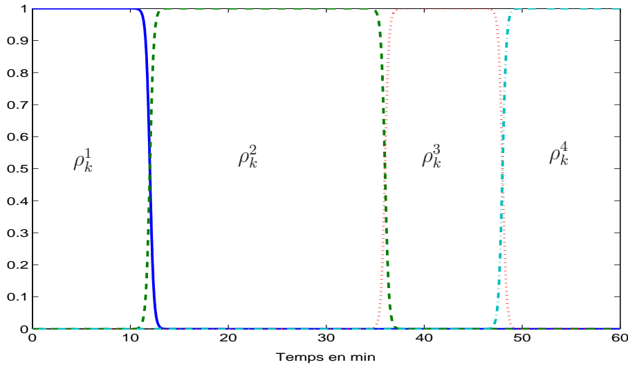
FIG. 3.9: Evolution des fonctions d'activation \rho_k^i
