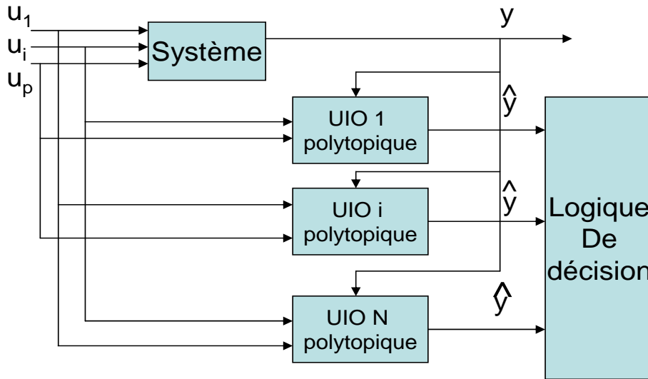
FIG. 3.12: Schéma de détection par UIO
