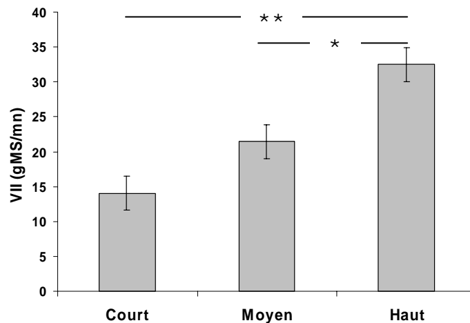
Figure II : Vitesse d'Ingestion Instantanée (VII en gMS/mn) pour les trois couverts (moyennes \pm erreurs standards) - * p < 0.05 , ** p < 0.01 ; Instantaneous Intake Rates (gDM/mn) for the three swards (means \pm S.E.) - * p < 0.05 , ** p < 0.01 (Short, Medium and Tall swards)
