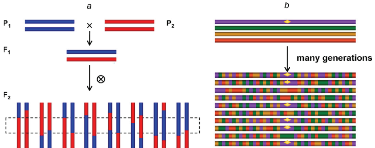
Figure 1.10 : Comparaison de l'étendue du DL (et donc de la résolution potentielle des associations marqueurs/caractères) entre les approches de cartographie classique (à gauche) et les études d'associations (à droite). Tiré de Zhu et al. (2008)
