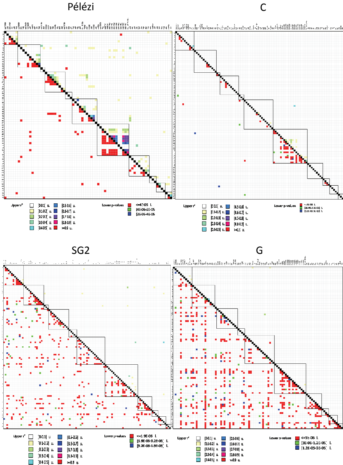
Figure 4.11 : Matrice de DL pour les groupes Pélézi, C, SG2 et G. Au-dessus des diagonales valeurs de r^2 , en dessous des diagonales valeurs des p-values associées aux tests exacts. Les seuils de r^2 sont donnés en légende. Les seuils de p-values sont les seuils de 1, 5 et 10% après correction de Bonferroni. Les carrés mis en évidence dans la matrice correspondent aux différents groupes de liaison de la carte génétique
