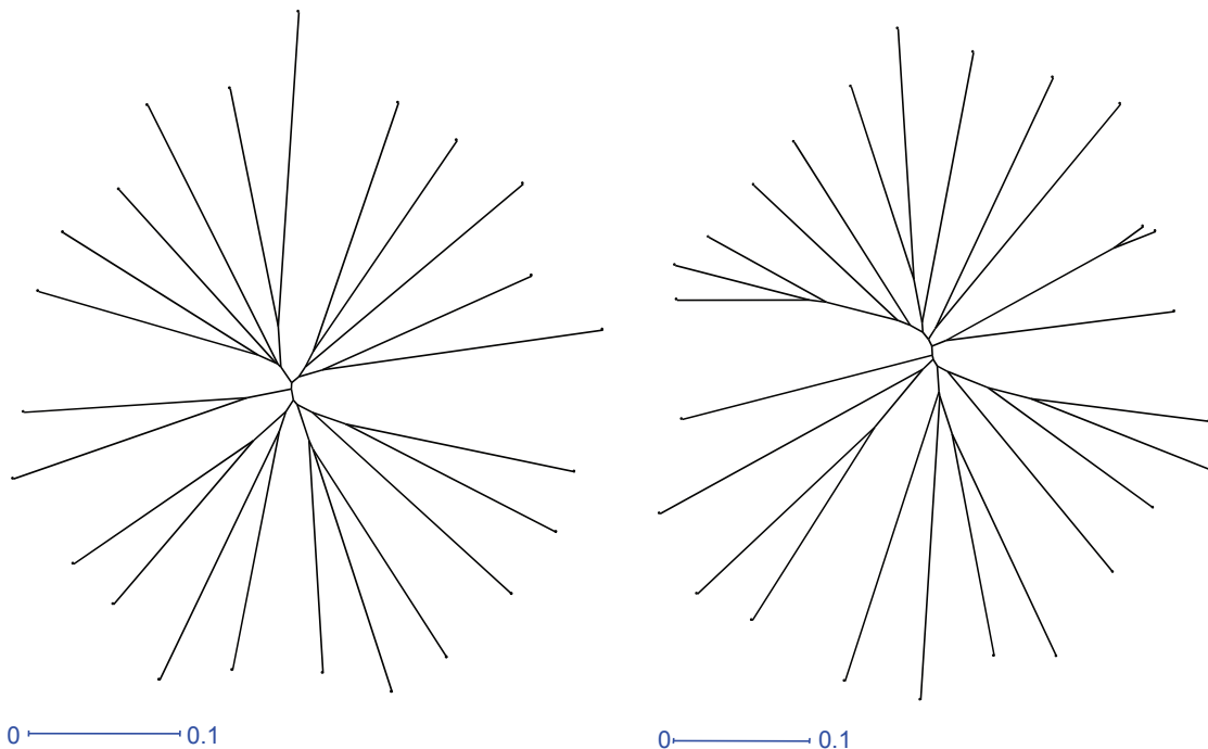
Figure 5.2 : Arbres NJ des sous-échantillons des groupes C (à gauche) et G (à droite). Les échelles de distance données correspondent à l'index de Simple-Matching
