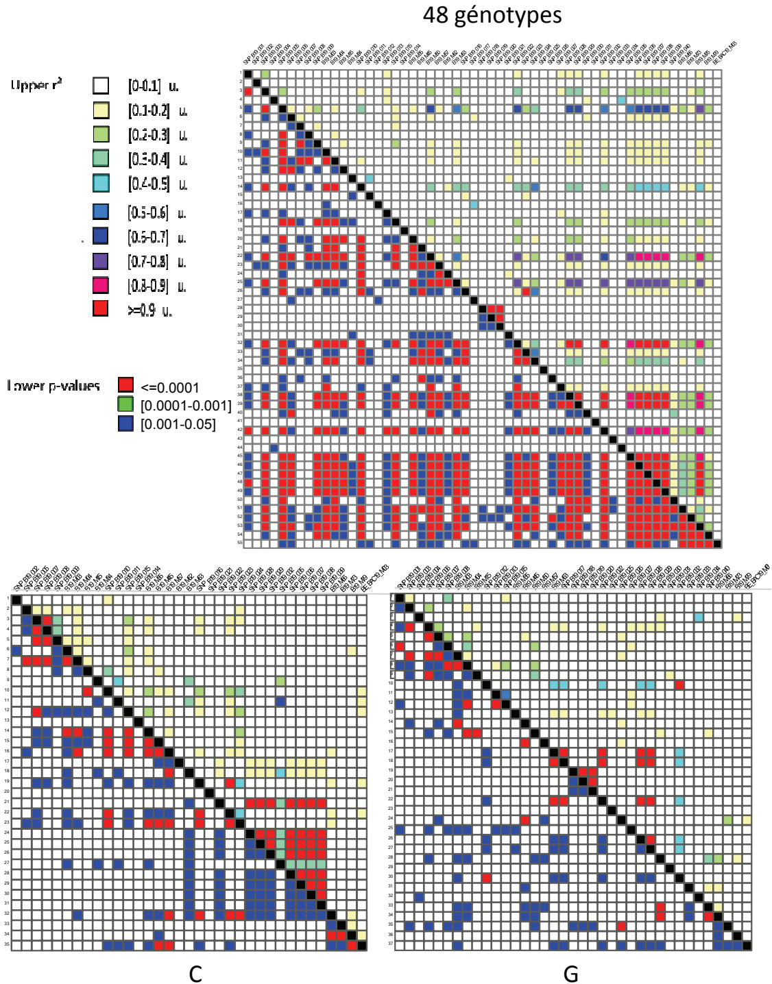
Figure 5.7 : Matrices de DL du clone BAC 111018 entre marqueurs 2 à 2. Au-dessus des diagonales sont présentées les valeurs de r^2 (les seuils sont donnés en légende), en dessous les valeurs des p-values associées aux tests exacts de Fisher aux seuils de 1 pour 1000, 1 pour 100 et 5 pour 100 (sans correction)
