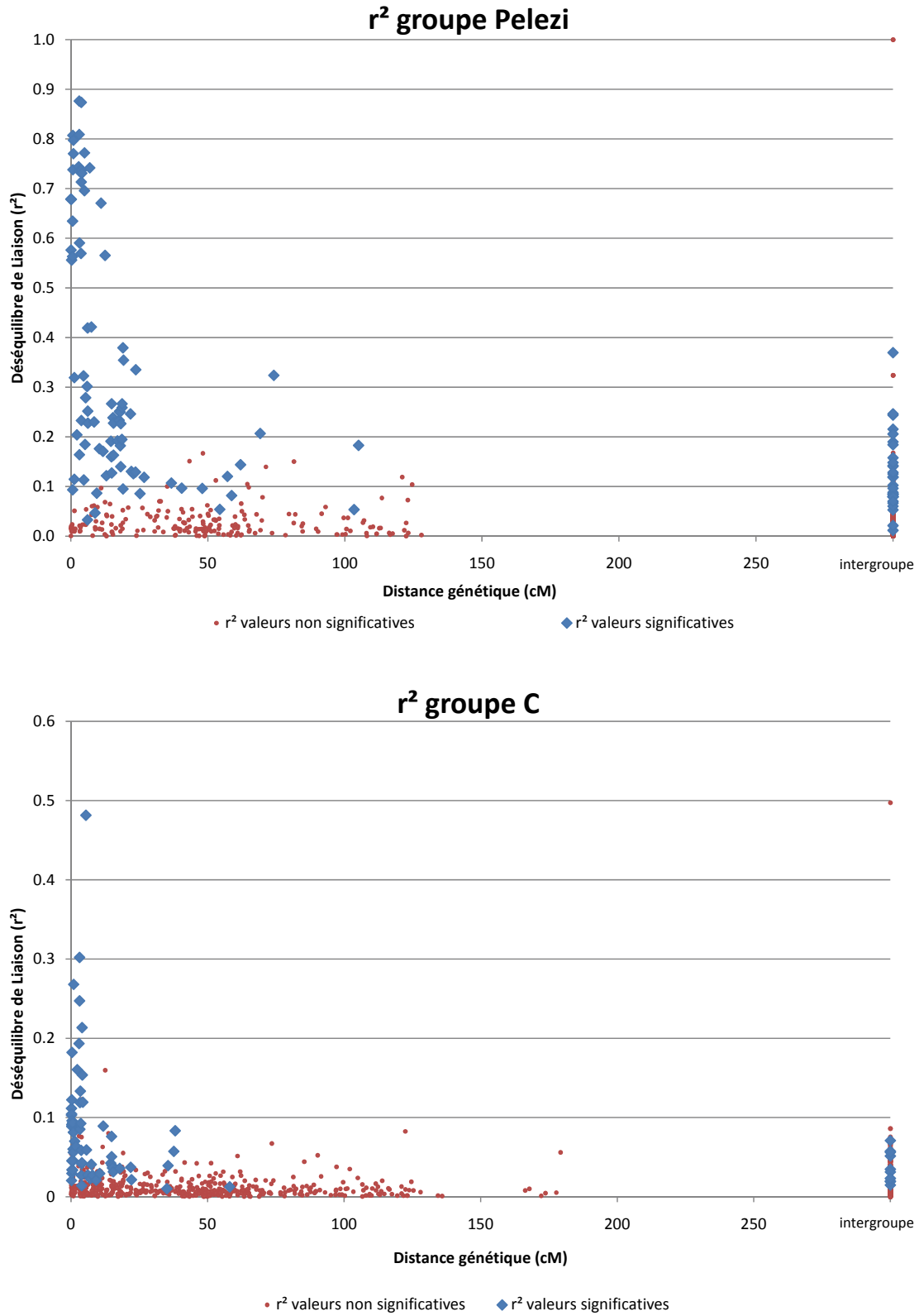
Figure 4.9 : r^2 en fonction de la distance génétique pour les groupes Pélézi (haut) et C (bas). Les valeurs en bleu sont les valeurs de r^2 significatives au seuil de 5% après correction de Bonferroni, les valeurs en rouge sont non significatives à ce seuil
