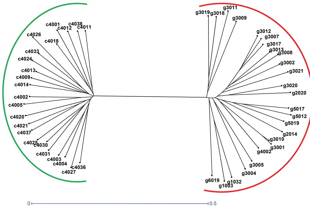
Figure 5.1 : Arbre NJ des 48 individus utilisés dans cette étude, à gauche les génotypes appartenant au groupe C (en vert), à droite ceux appartenant au groupe G (en rouge). L'échelle de distance donnée correspond à l'index de Simple-Matching utilisé pour calculer les dissimilarités entre individus à l'aide du logiciel DARwin (Perrier et al. , 2003)
