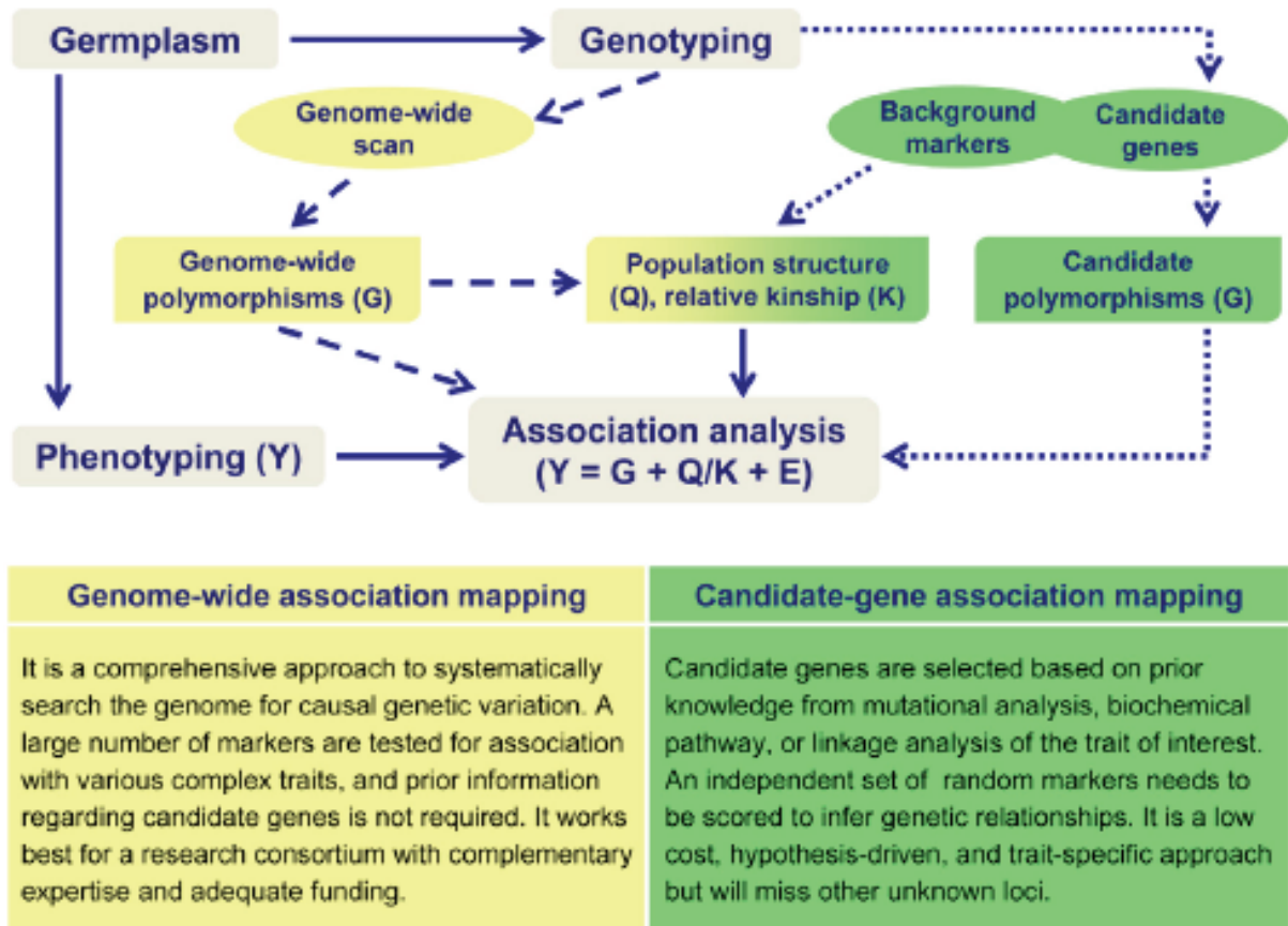
Figure 1.12 : Diagramme schématisé et contraste entre les approches génome entier et gène candidats. Tiré de Zhu et al. (2008)
