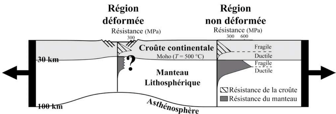
Figure i.1. Schéma d'un rift continental étroit à l'échelle de la lithosphère, qui illustre les résistances du manteau sous-continentale observées sous les régions déformées (rift ou chaîne de montagne) et les régions non déformées à partir des données géophysiques. La faible résistance du manteau sous les régions déformées n'est pas prédite par les données rhéologiques, ce qui a fait l'objet de cette thèse.
