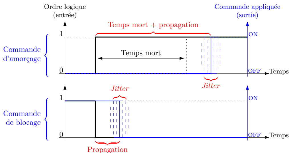
Figure 3.3 – Formes d’ondes schématisques des signaux de commande d’un transistor en entrée et en sortie de driver .
