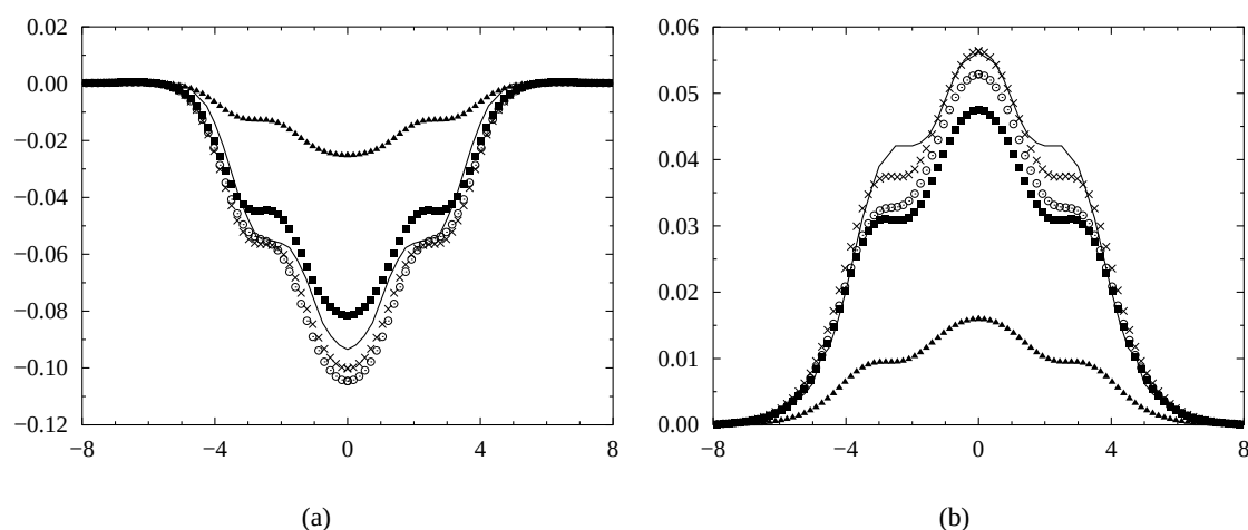
FIG. 4.2 – 150 kHz, partie réelle (a) et imaginaire (b) de la variation d'impédance de la sonde \Delta Z (Ω) selon l'axe x (mm); mesure (trait continu), solution exacte (croix), LN (cercle), QLS (triangle), QA (carré)
