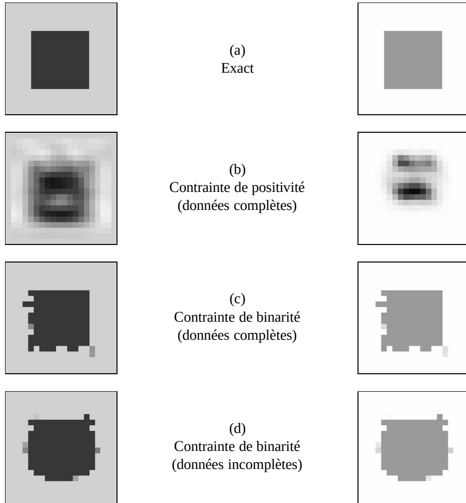
FIG. 3.3 – Comparaison de reconstructions obtenues par les différents gradients modifiés contraints développés au DRÉ. À droite, la carte de permittivité, et à gauche, la carte de conductivité.
