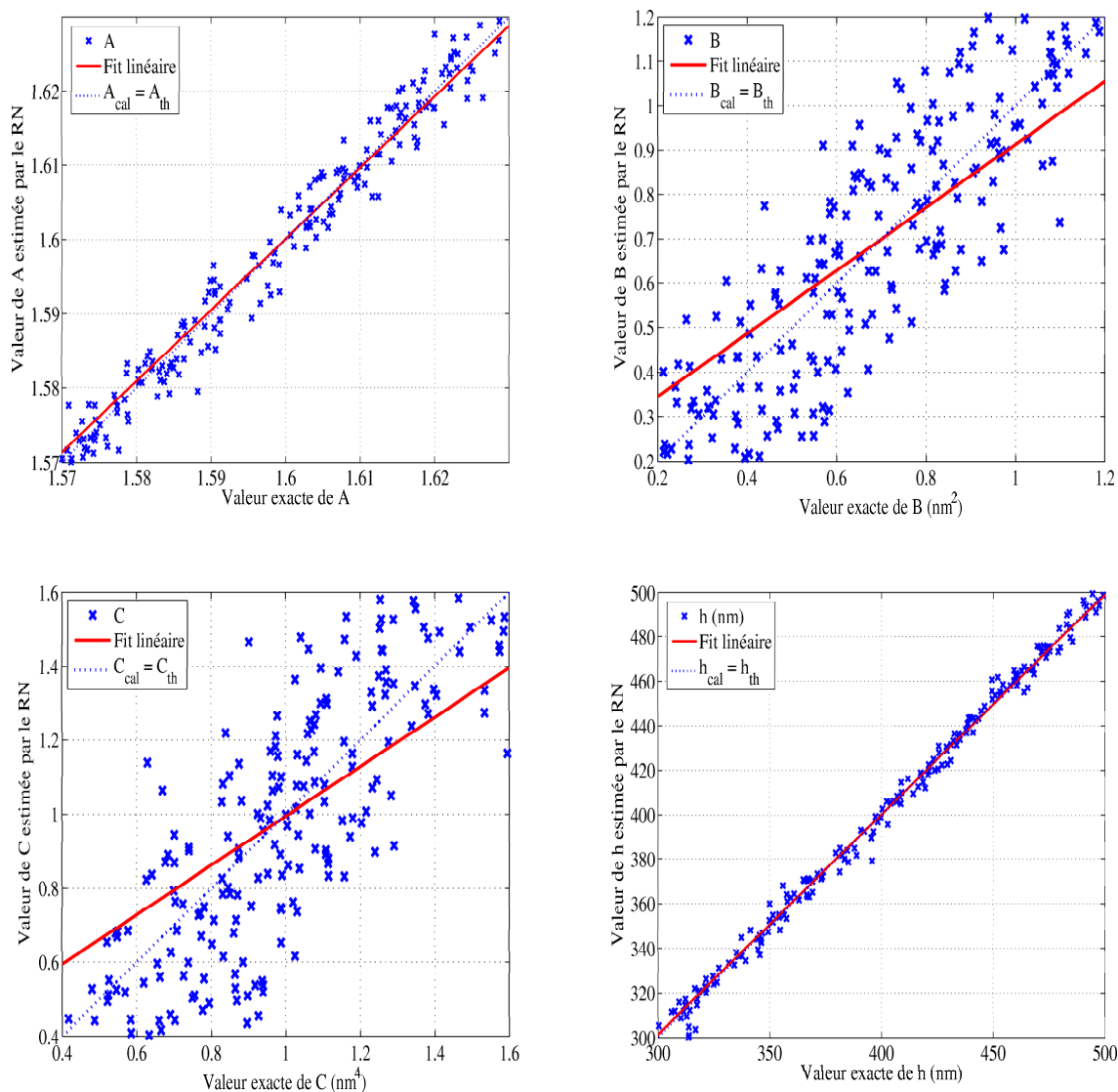
FIG. II.15: Représentation des différents paramètres opto-géométriques A , B , C et h calculés par le PMC à partir des signatures bruitées de 200 échantillons test en fonction de leurs paramètres exacts connus.
