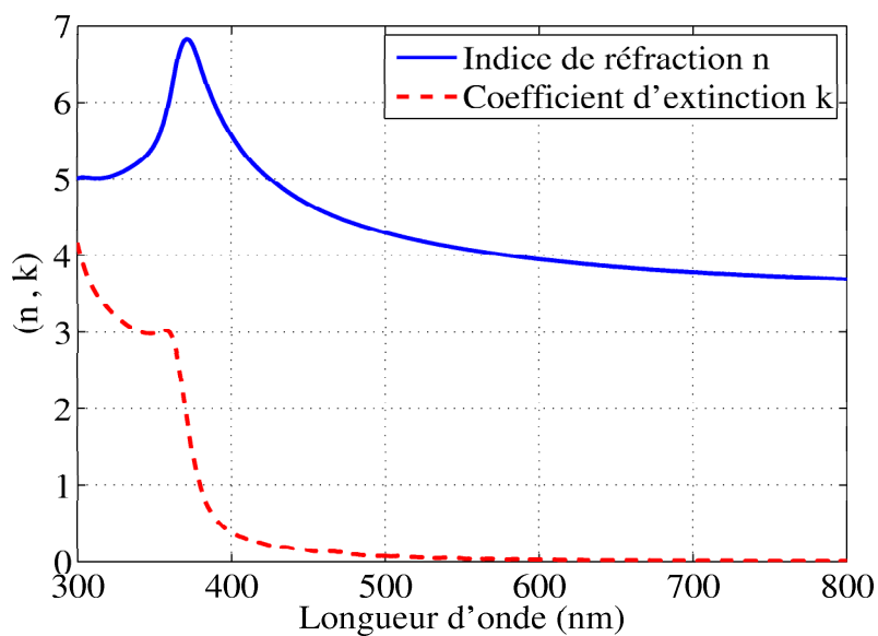
FIG. III.53: Indice de réfraction n et coefficient d'extinction k du silicium.
