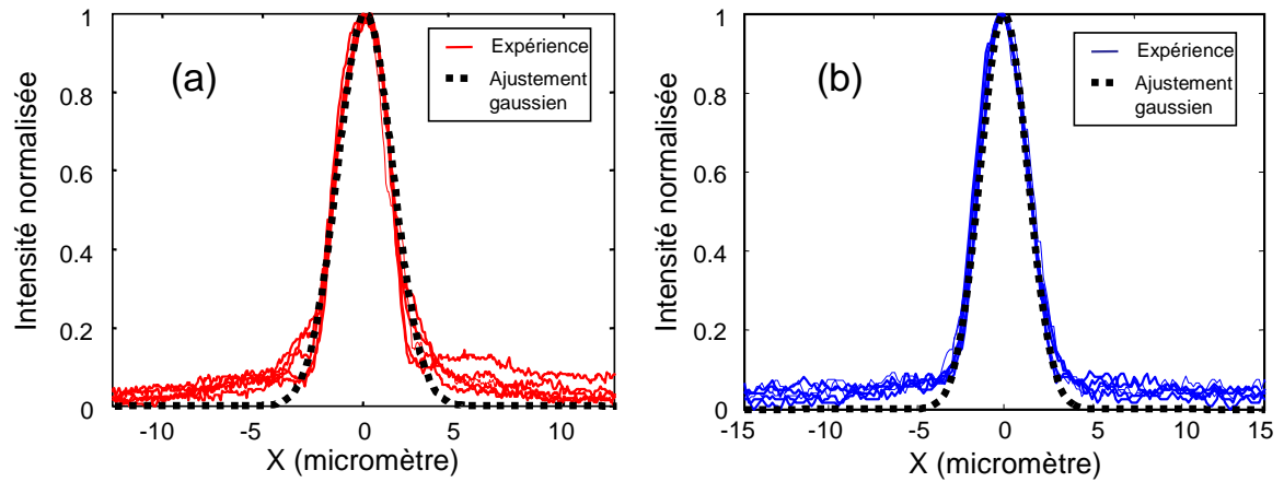
FIG. 3.4 – Distribution de la lumière en sortie de la fibre FMC 2S1G (a) et FMC \text{As}_2\text{Se}_3 (b).
