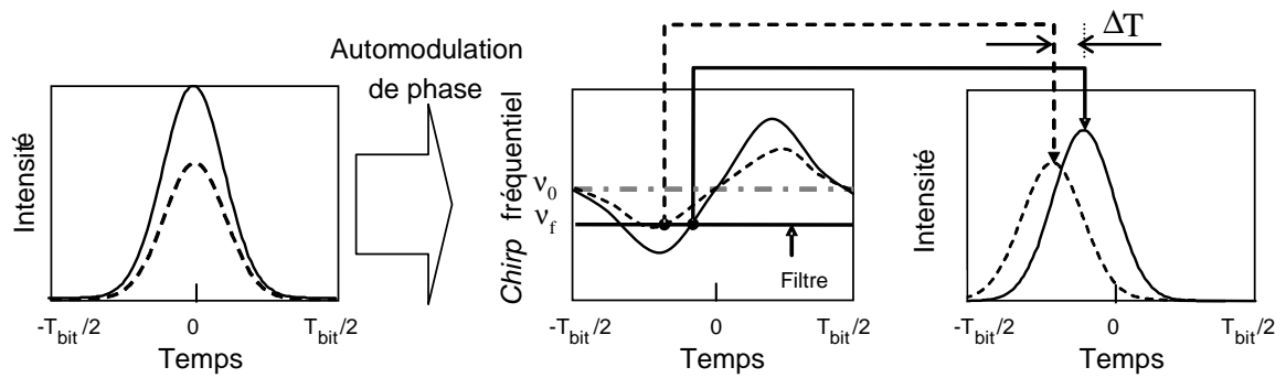
FIG. 4.26 – Illustration du décalage temporel induit par automodulation de phase entre deux impulsions de puissance crête différente.
