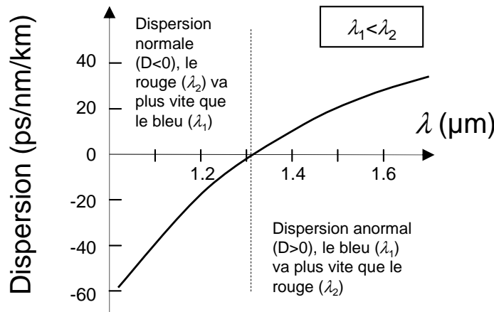
FIG. 1.16 – Courbe de dispersion de la fibre SMF.
