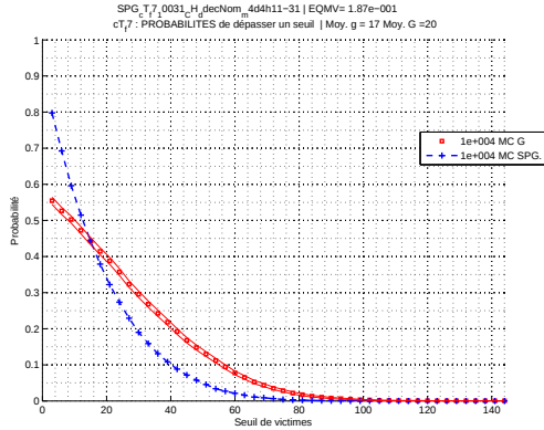
(c) Sparse grid à 1000 points : courbe des probabilités
