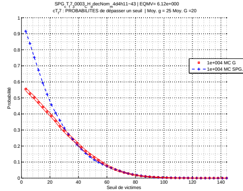
(d) Sparse grid à 3000 points : courbe des probabilités
