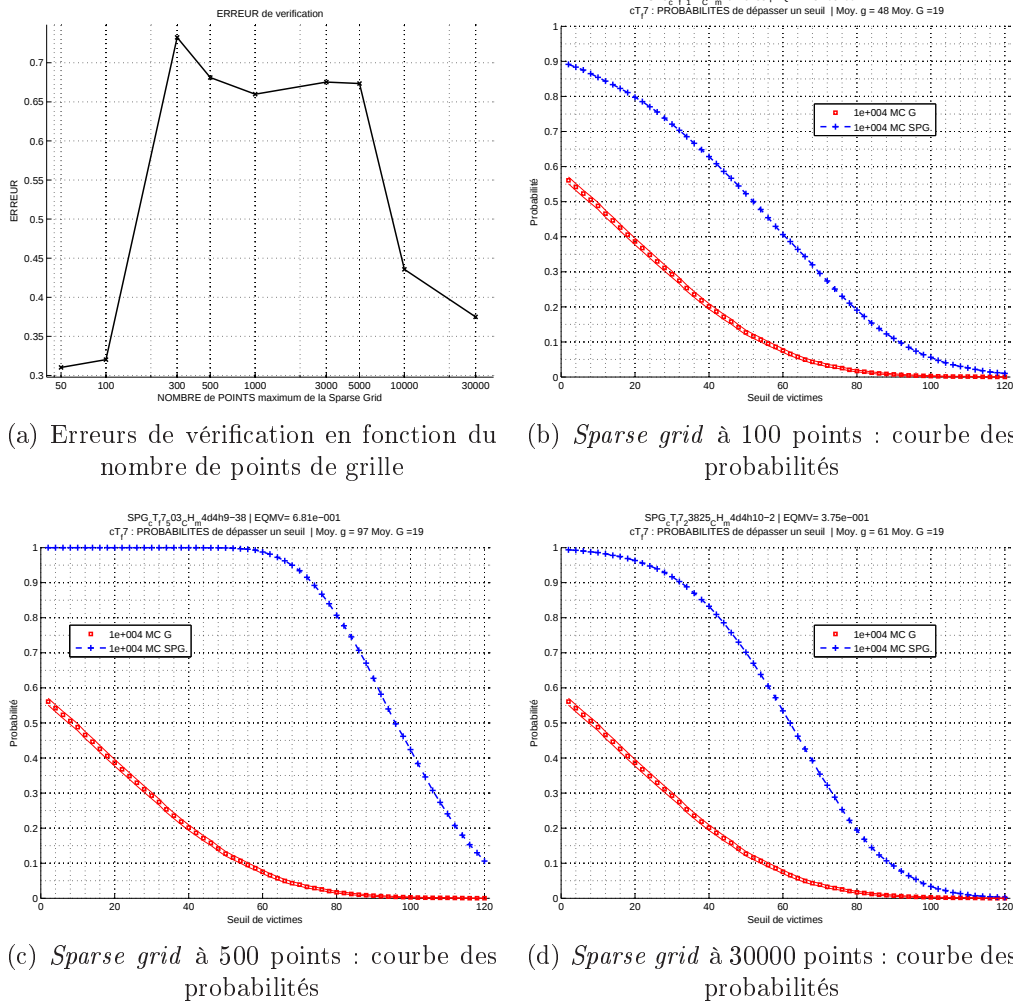
FIG. VI.24 – Sparse grids globales sans déplacement ( G_t ) : courbes des probabilités de dépasser un seuil et erreurs de vérification
