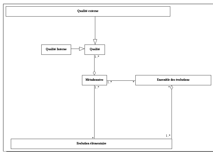
FIG. 3.6 – Métadonnées de qualité pour les évolutions
