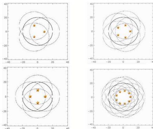
FIG. 7.3 – Recouvrement des pupilles à 10km pour un télescope de 42m. Les séparations sont données en mètres.
