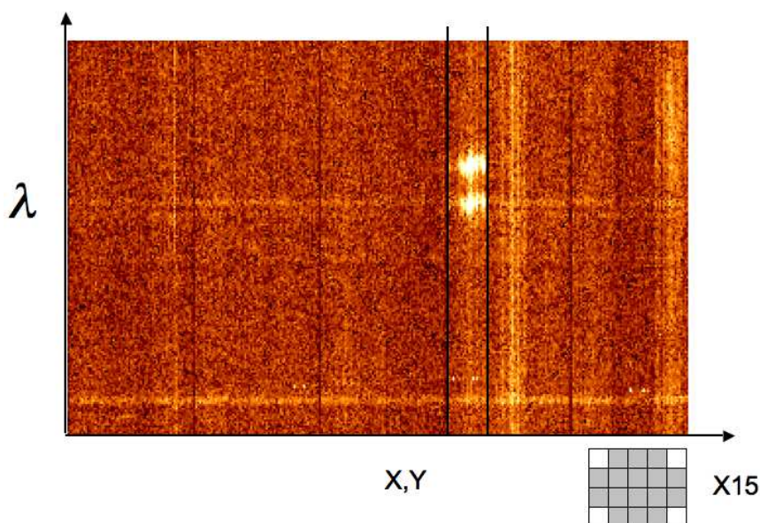
FIG. 3.1 – Exemple de spectres GIRAFFE. Chaque colonne représente un spectre obtenu par une fibre différente. Les colonnes sont rangées pour regrouper chaque objet. Un objet représente 20 fibres. Les raies en émissions d'un objet ont été détectées ici : on reconnaît le doublet [OII] (l'image n'est qu'une petite partie de la bande passante spectrale). Les bandes horizontales sont les raies du ciel.
