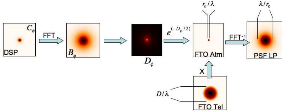
FIG. 5.8 – Principe de la simulation d'une PSF longue pose (pose infinie). C_\phi , B_\phi , D_\phi les FTO et la PSF sont en échelle Log inversée.
